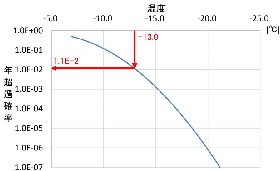
図 1 最低気温ハザード曲線
