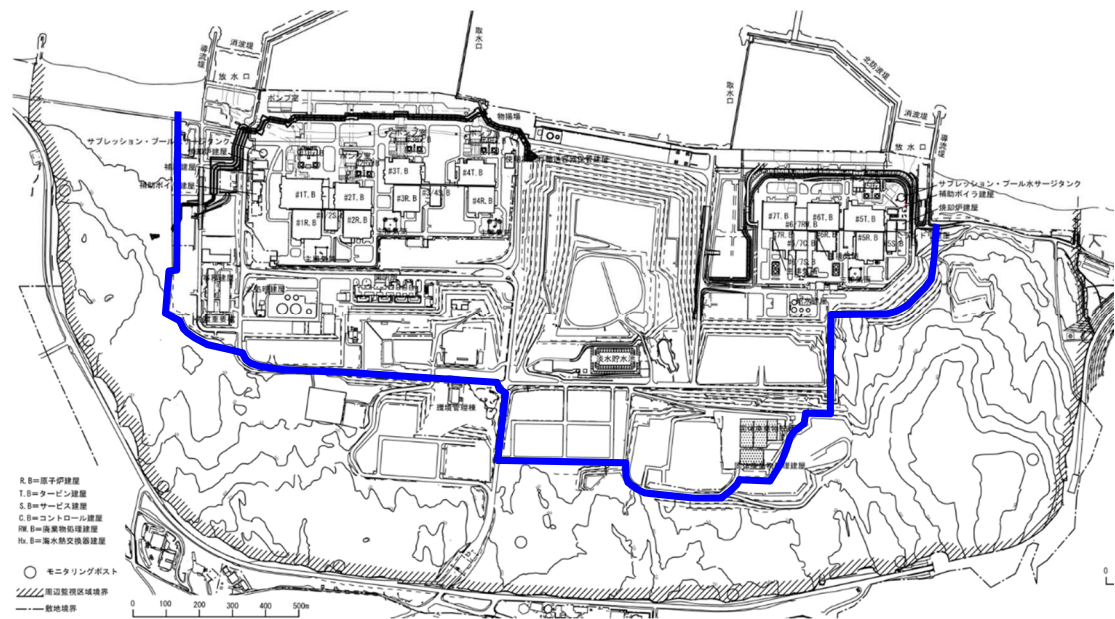
第 2.4.3.1-1 図 防火帯配置図
