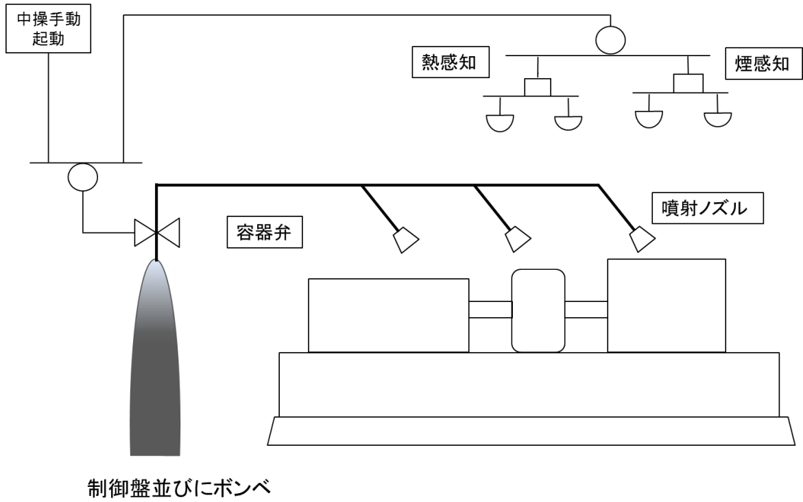
(a) 油内包機器消火設備の例
