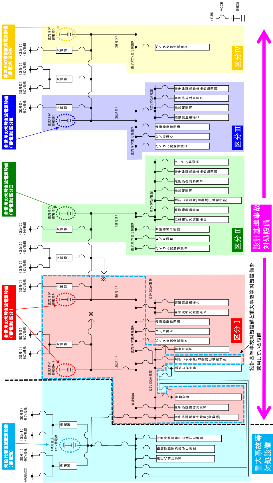
図6：直流電源設備の遮断器及びメカニカルインターロックによる分離（7号炉）
