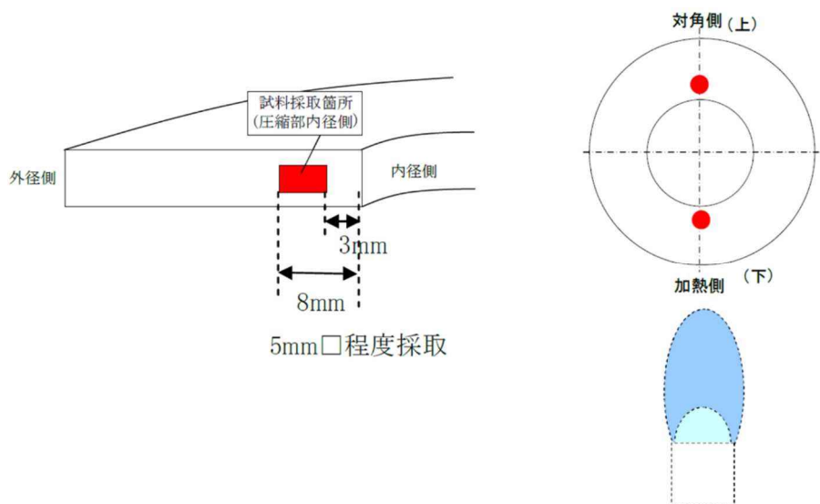
図 3 熱定量測定 of 測定箇所
