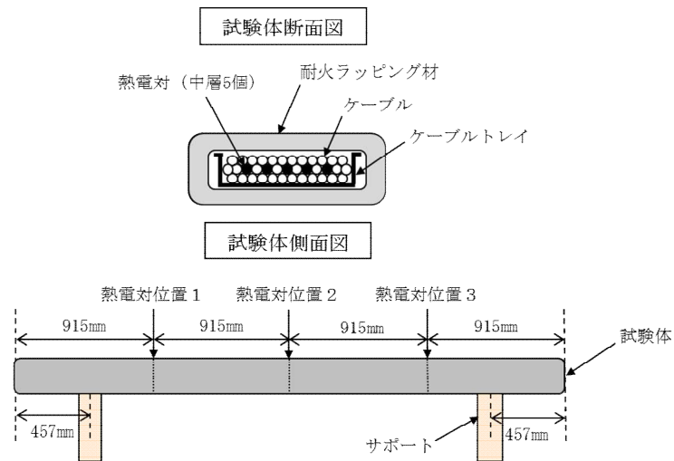
図 14 許容電流低減率（ADF）の評価用試験体の構造の例
