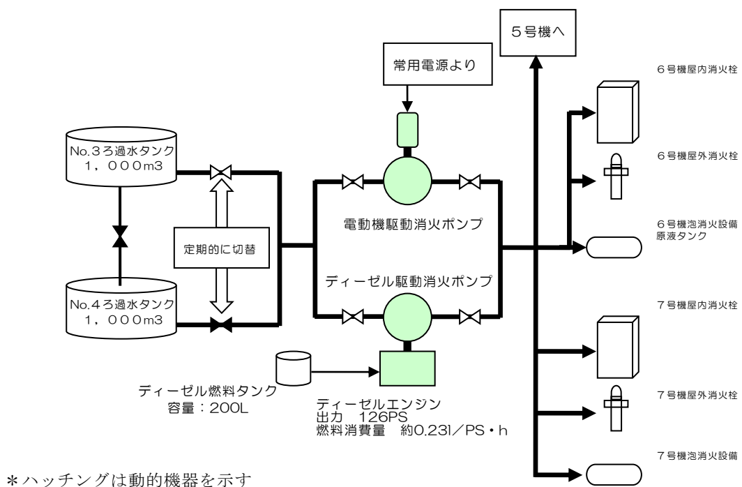
図 1-22：消火水系の概要
