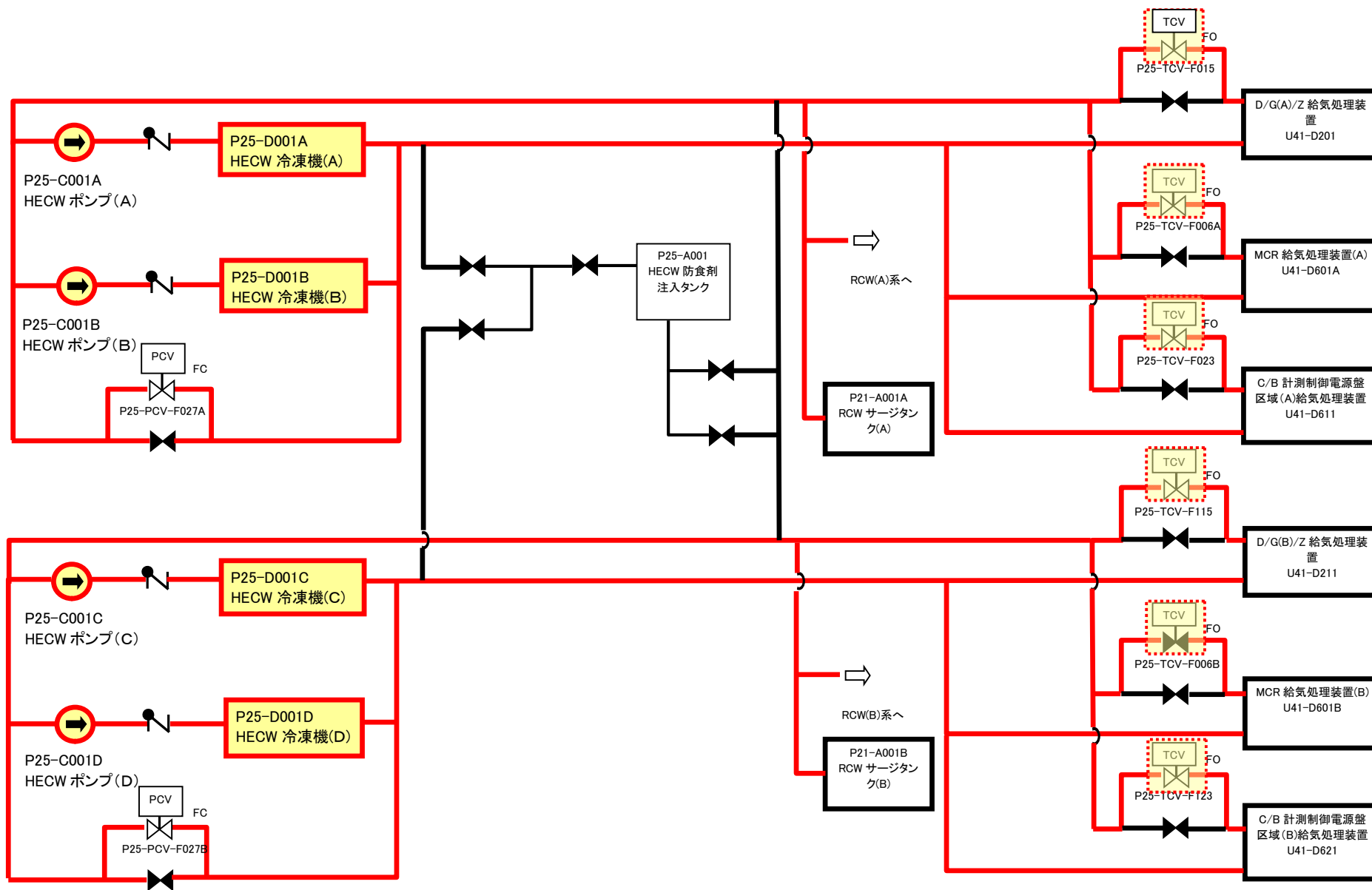
図 7 換気空調補機非常用冷却系
