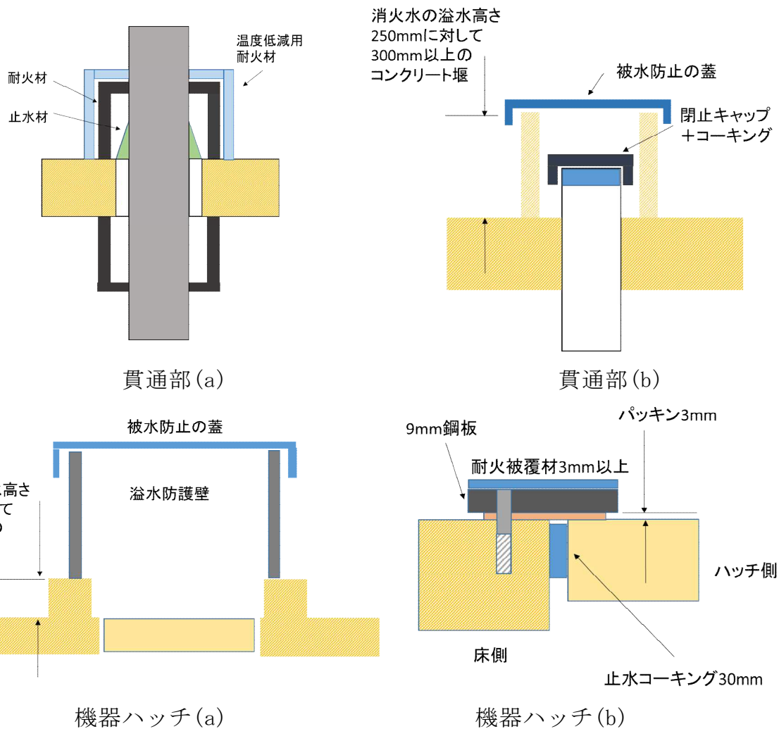
図 5-2 : タービン建屋 (2)
