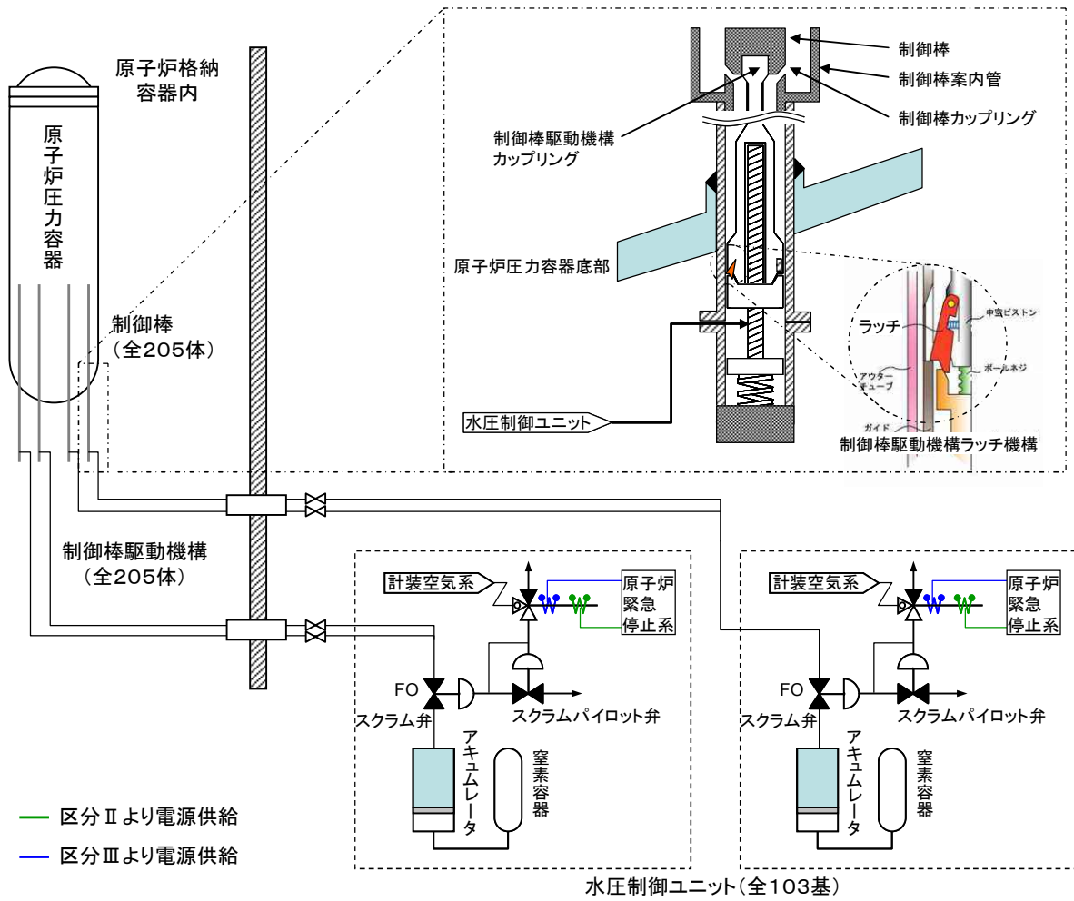
図 2-1：制御棒及び制御棒駆動系（水圧制御ユニット）の系統概略図
