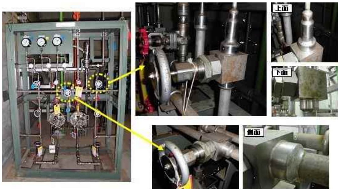
図 1-3 : 溶接構造・ベローズ弁の例 (発電機水素ガス供給装置)
