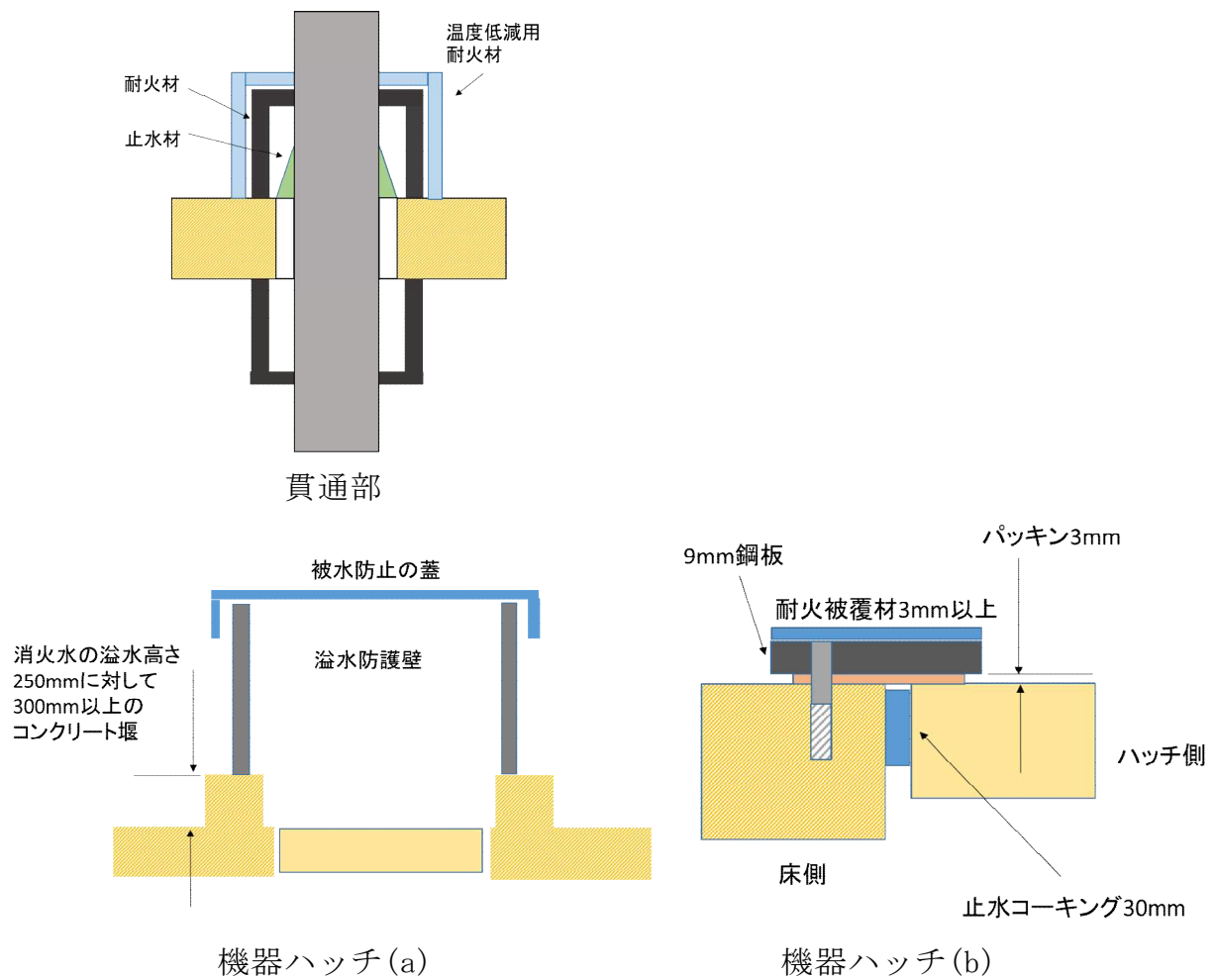
図 5-1 : タービン建屋 (1)
