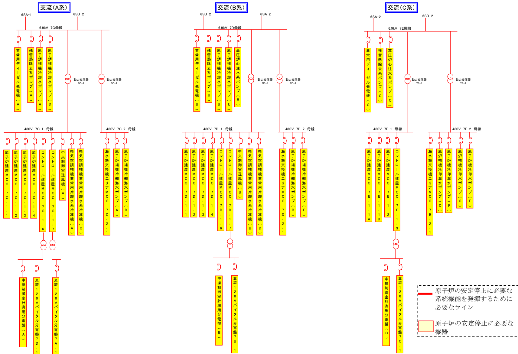
図 13 非常用電源系
