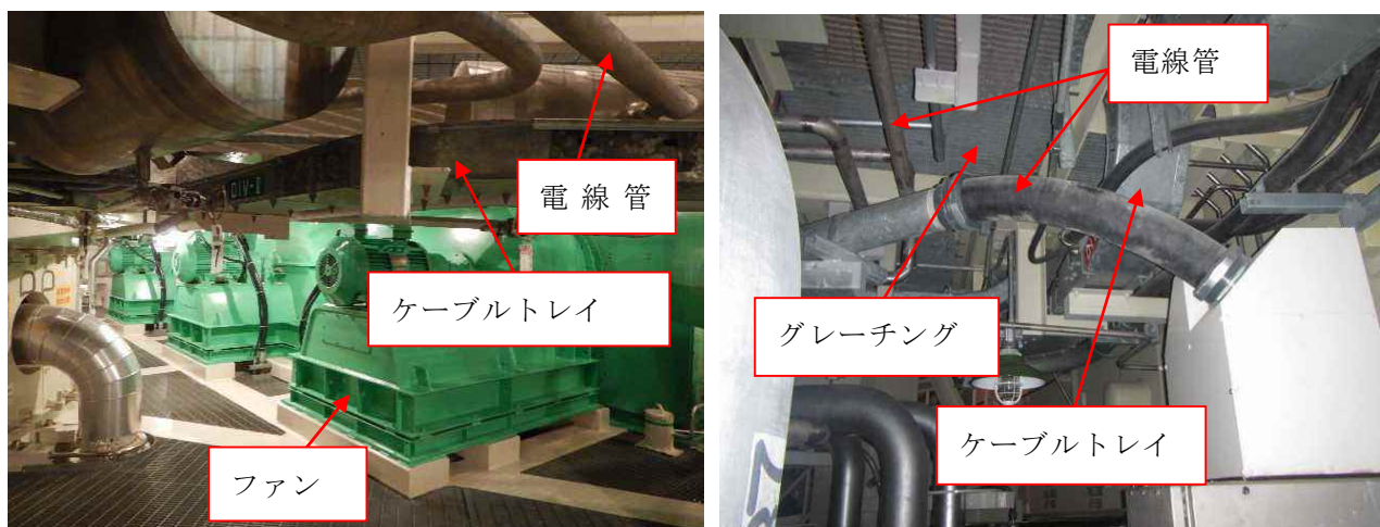
図 8-6 原子炉格納容器内の機器等の設置状況
