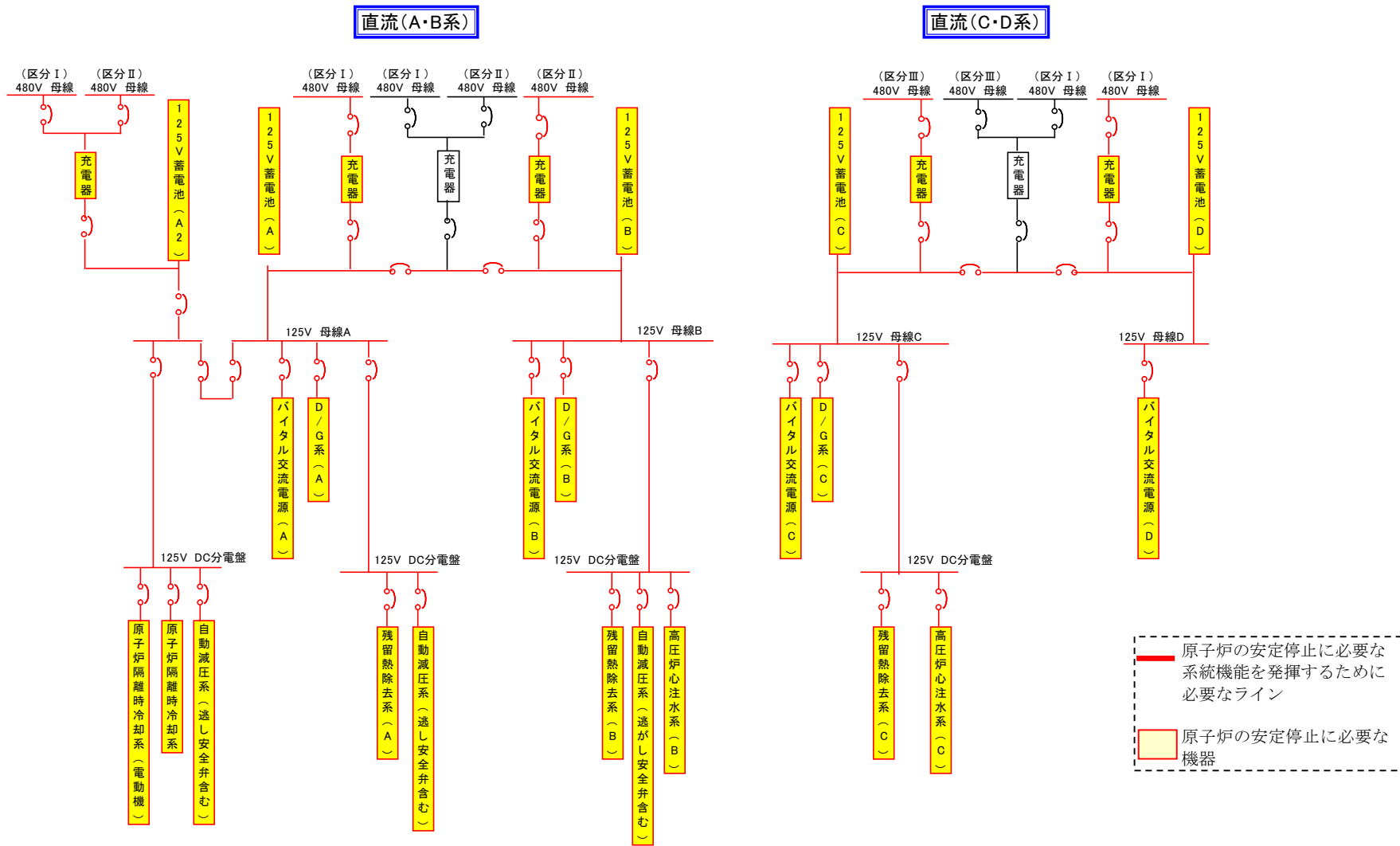
図 14 直流電源系
