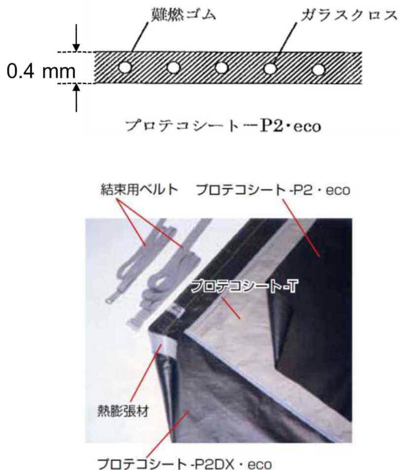
図 1：延焼防止シート（プロテコシート P2・eco）の概要
