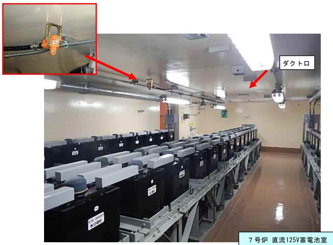
図 1-7：蓄電池室内の水素濃度検出器設置状況
