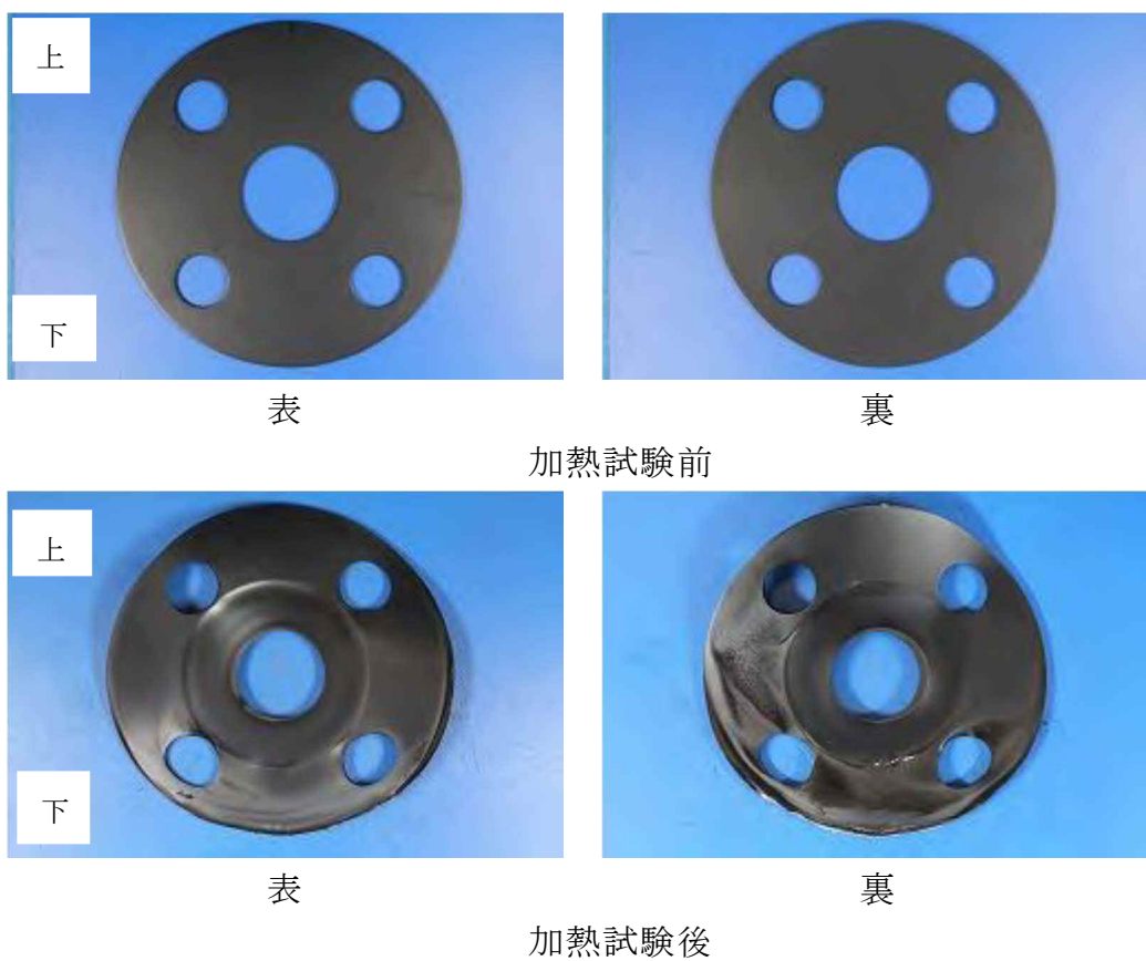
図6 加熱前後の試験体シート面（ゴム打ち抜きガスケット）
