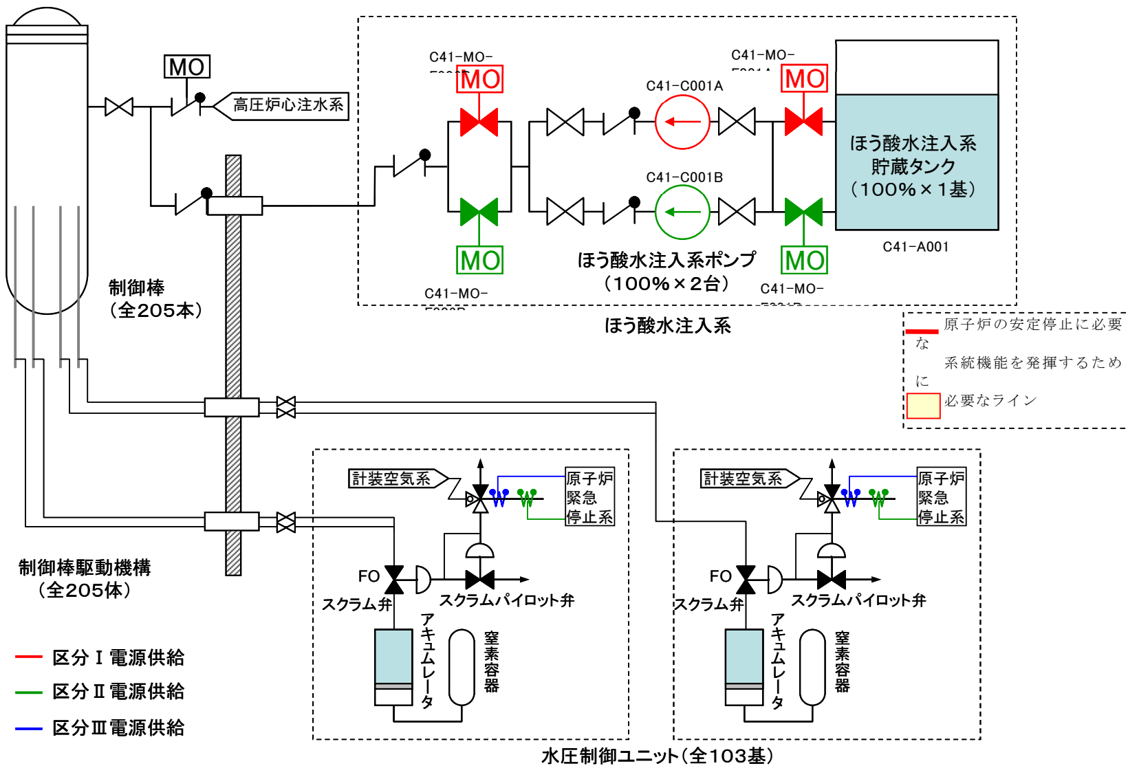
図8-18 ほう酸水注入系及び制御棒による系の概要
