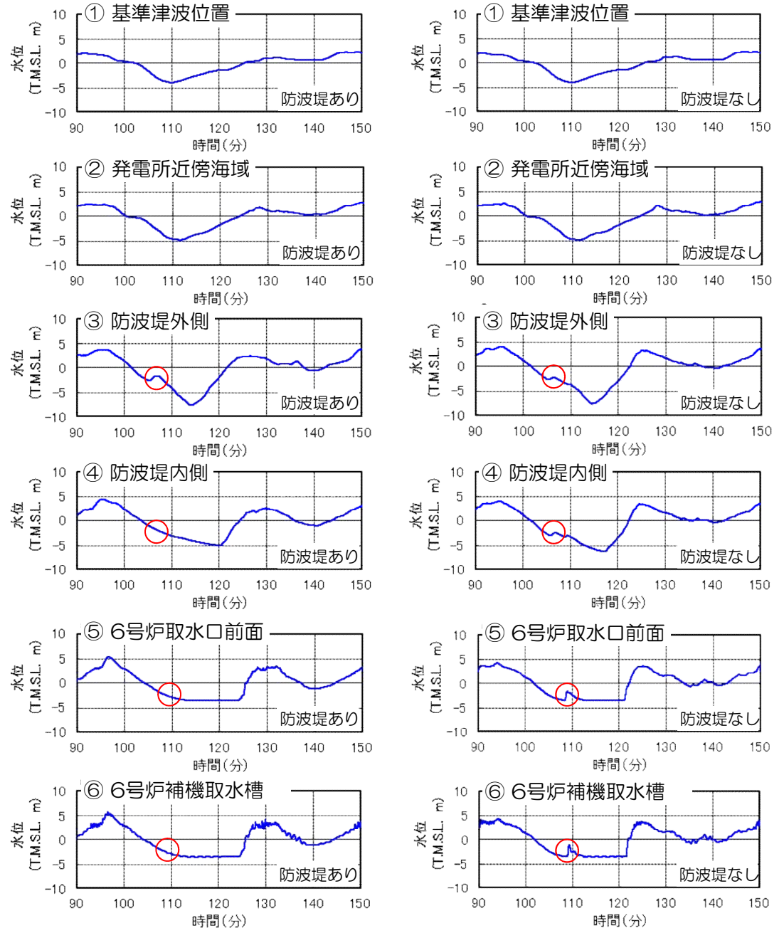
時刻歴波形（左：防波堤あり 右：防波堤なし）
