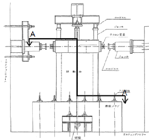
既往の加力試験装置 (1/10縮尺試験体) の概要
