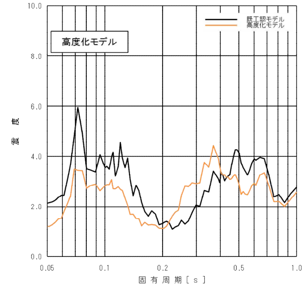
原子炉遮蔽壁(T.M.S.L.18.440m, Ss-1, NS方向, 減衰2.0%) における応答スペクトル比較
