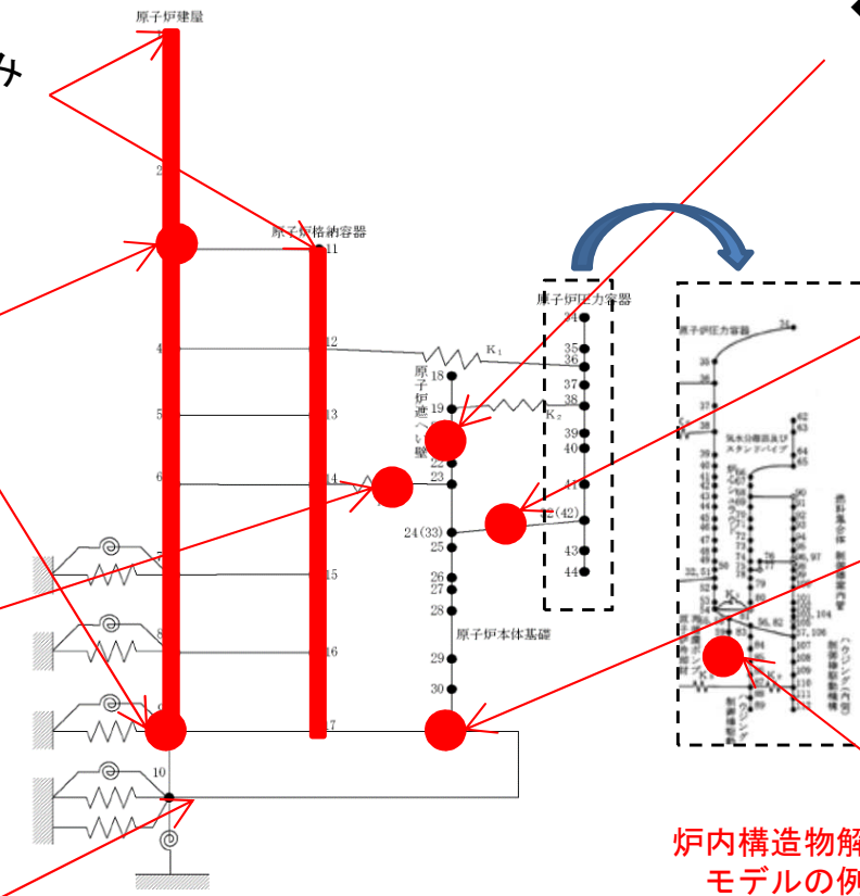
原子炉建屋—大型機器連成解析モデルの例
