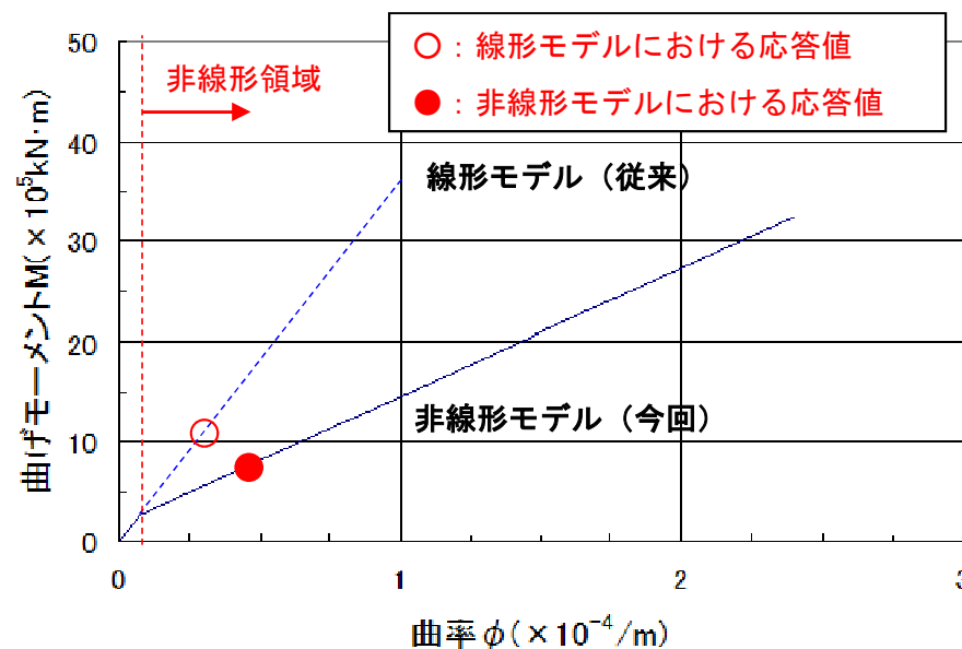
原子炉本体基礎のスケルトンカーブの例 (7号炉, Ss-1, NS方向の概算値)
