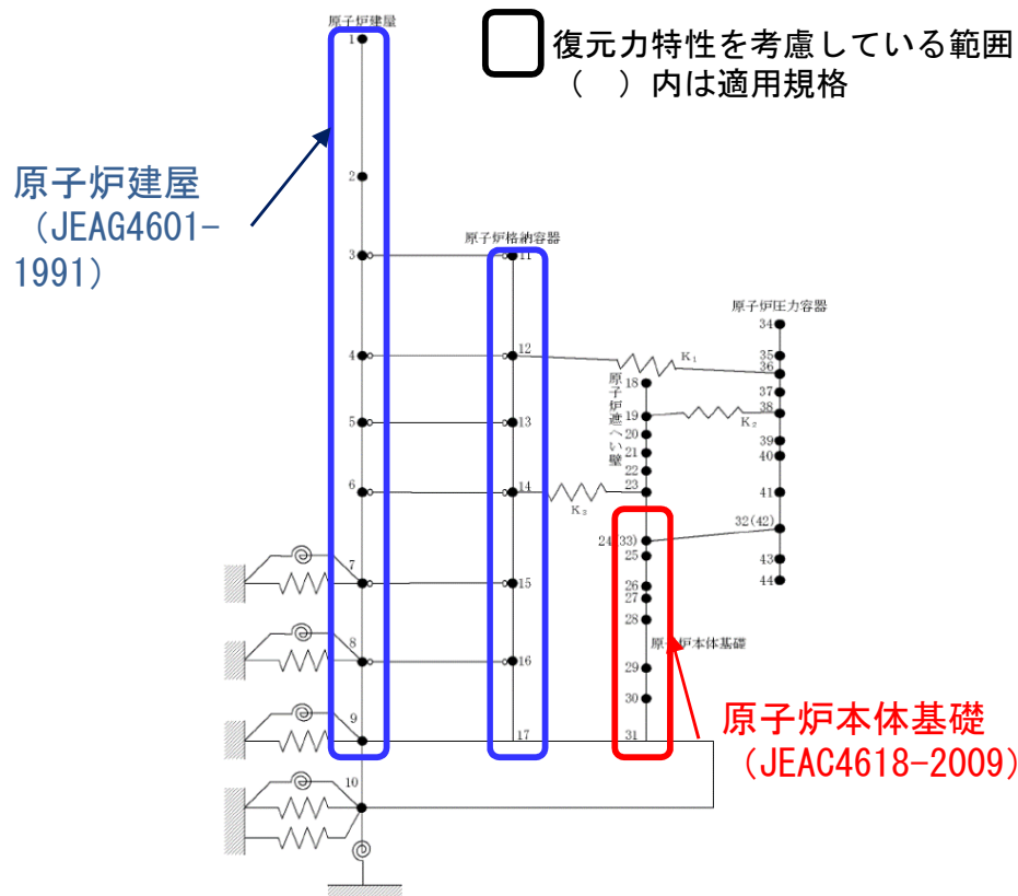
原子炉本体基礎の地震応答解析モデルの例
