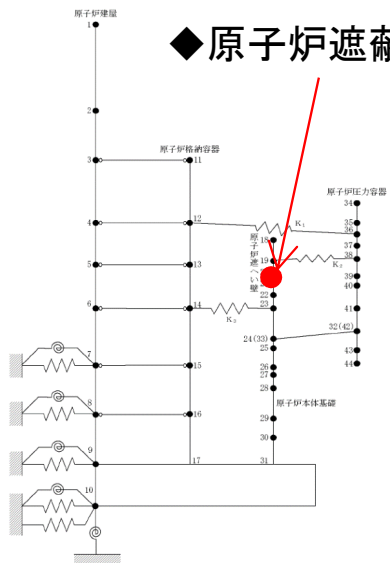
主蒸気系配管評価用 構築物間相対変位 (水平方向)
