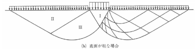
図 10.10 一般的なすべり面の形状
