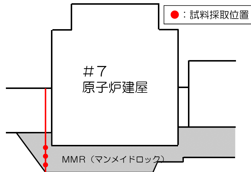
A-A'断面図
