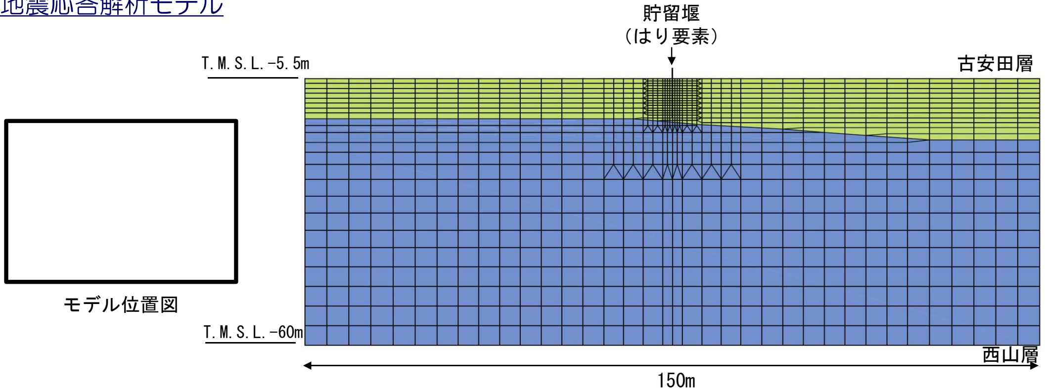
地震応答解析モデル
