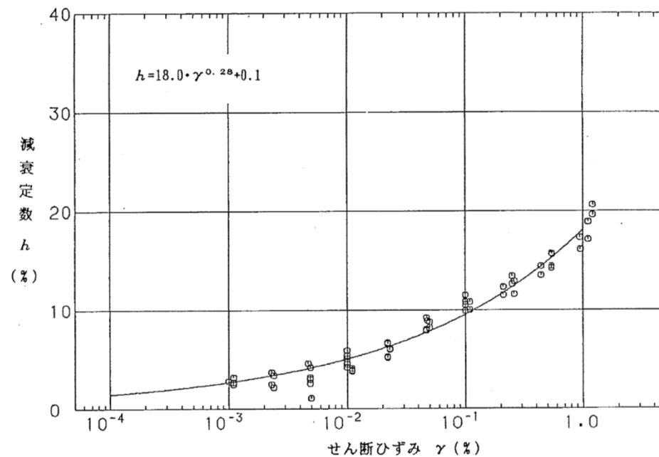
V 2 断層の動的変形特性
