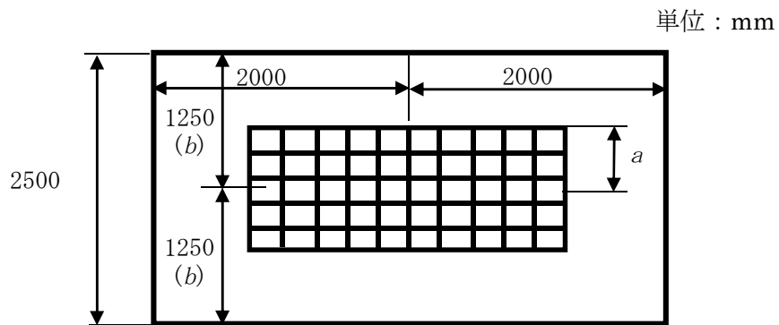
図一別紙 6 - 2 試験水槽形状図
