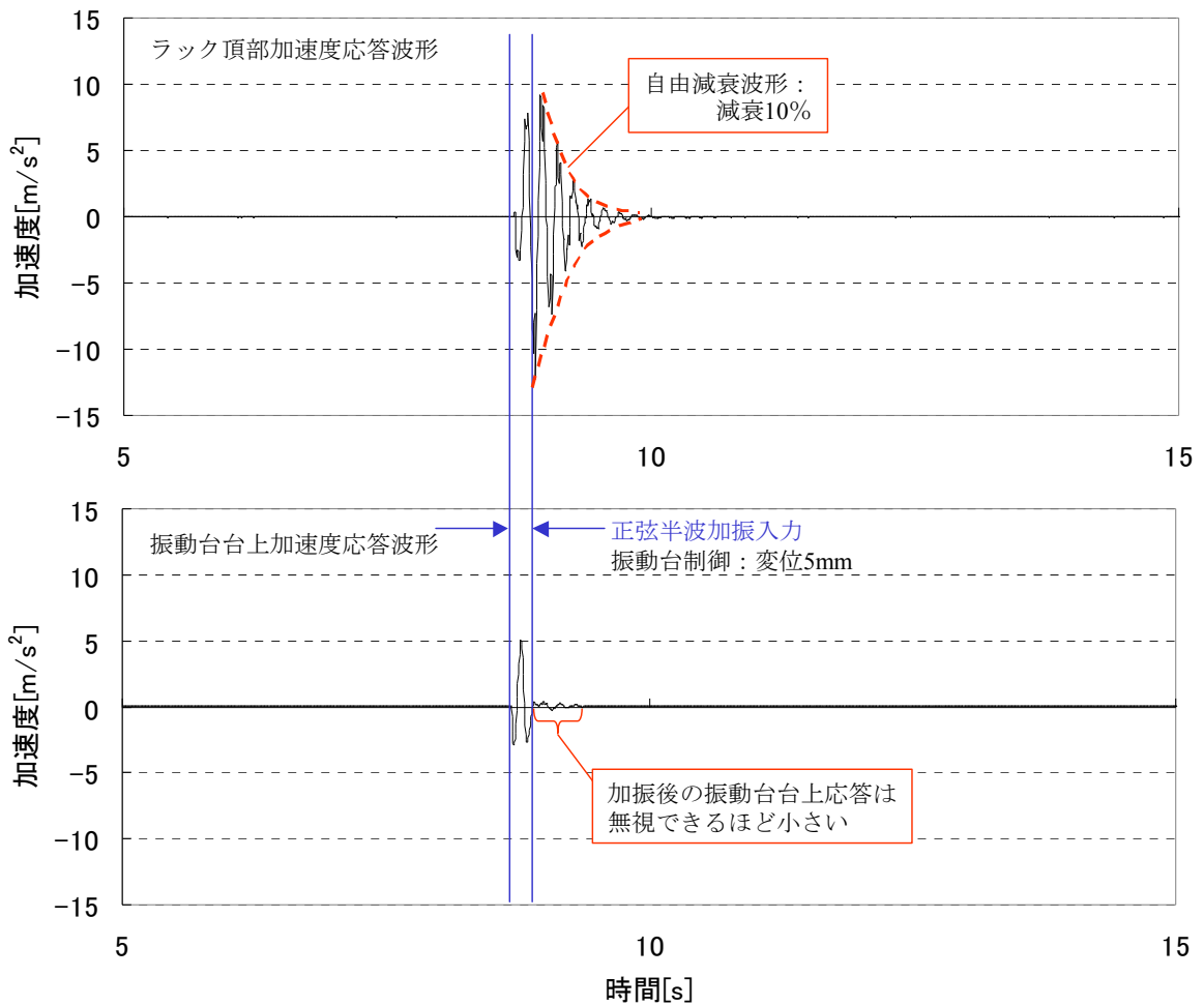
図－別紙4－1 燃料ラックの自由振動波形と減衰定数 (正弦半波加振試験, 短辺方向, 振動台上加速度 5.00m/s^2 )
