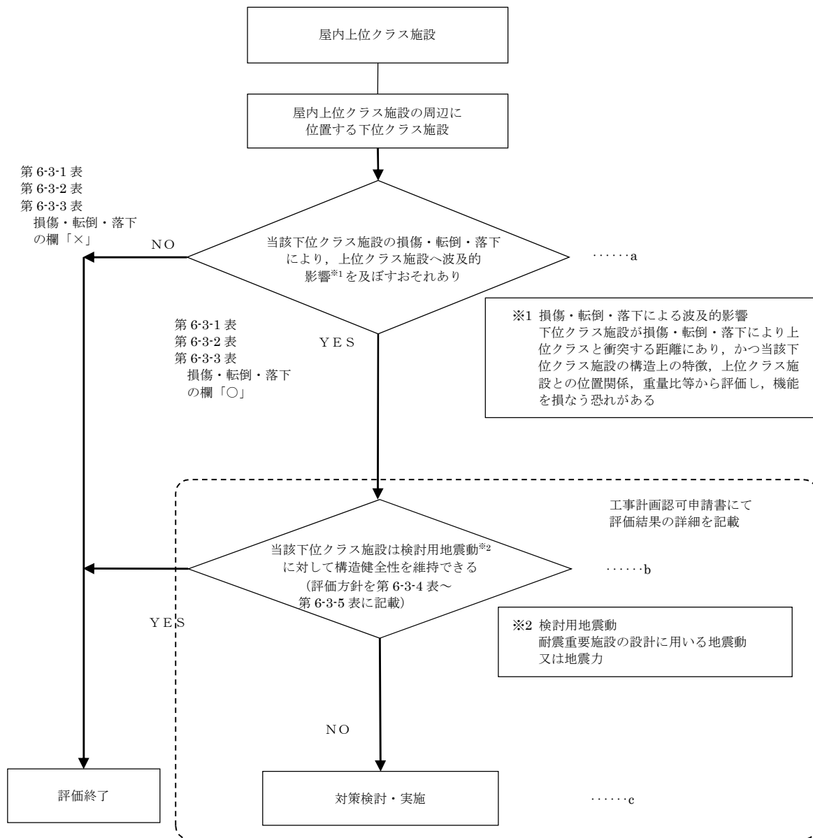
第5-3 図 損傷，転倒及び落下により屋内上位クラス施設へ影響を及ぼすおそれのある下位クラス施設の抽出及び評価フロー
