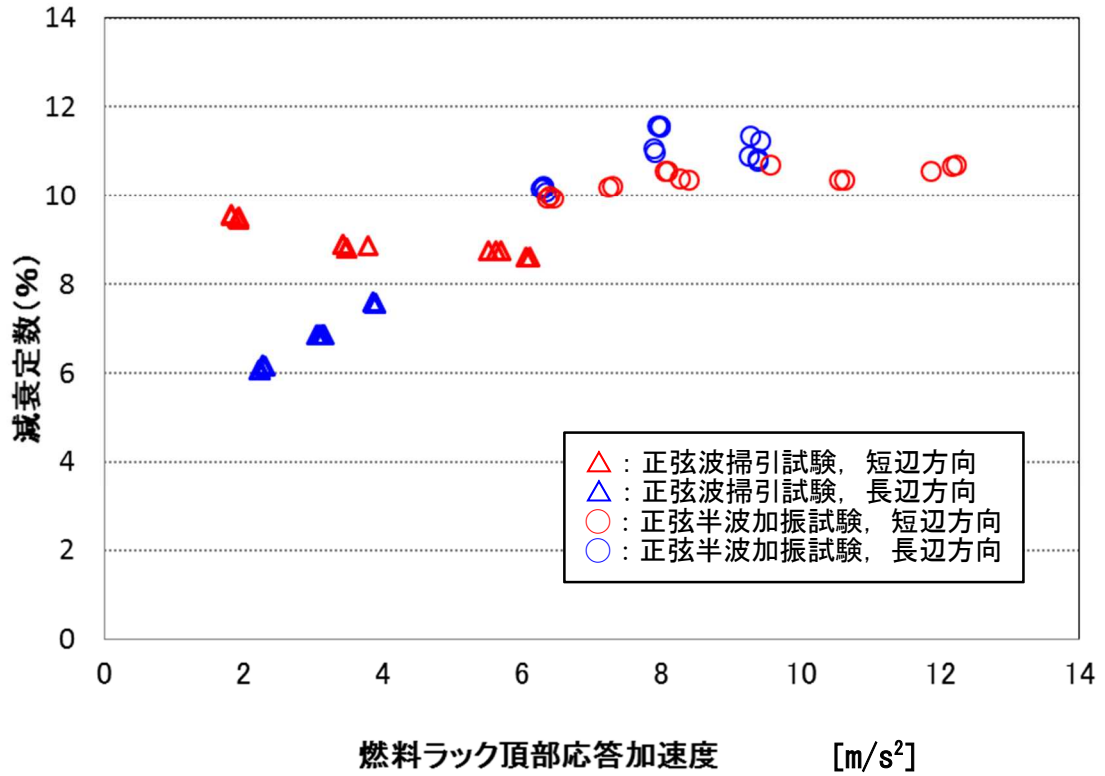
図 10 燃料ラック頂部最大応答加速度と減衰定数の関係
