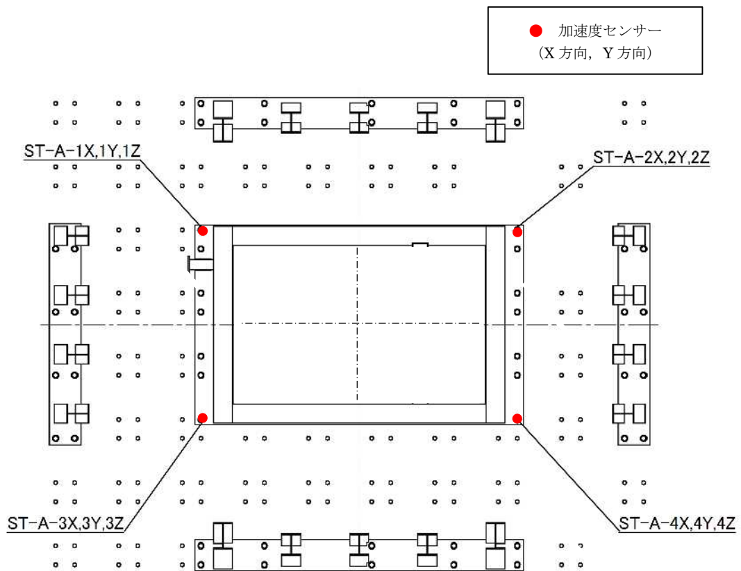
図 8 ( 2 / 2 ) 振動台上の加速度の計測位置
