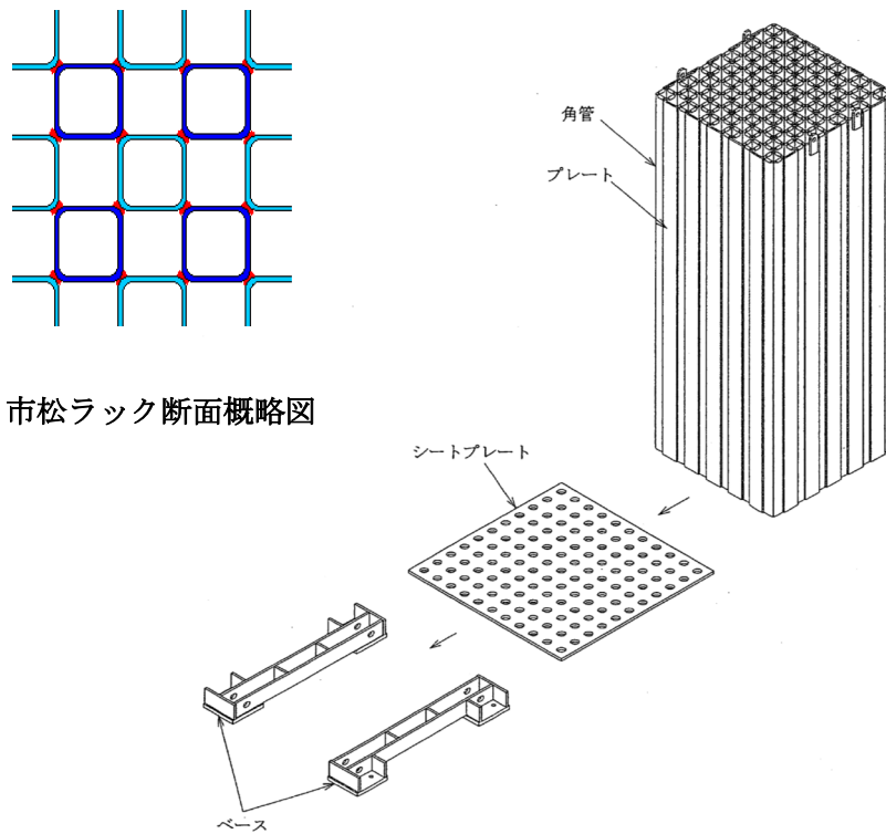
図 4 燃料ラックの構造図
