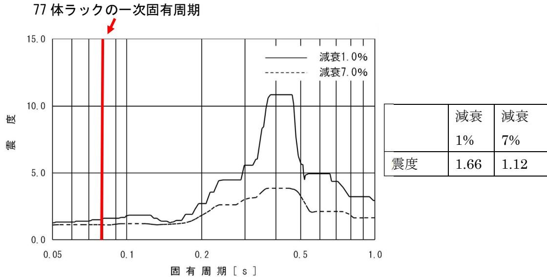
図 2 基準地震動 Ss, 燃料ラック設置位置における水平床応答スペクトル比較 (R/B, T.M.S.L 23,500 mm)
