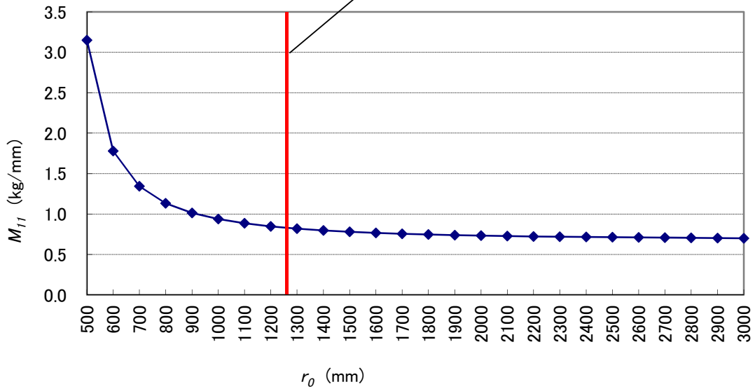
図一別紙 6-1 ラックとプールの隔壁間の距離とラックの付加質量
