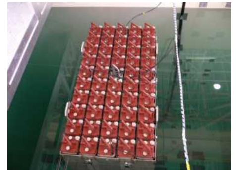
(4) 市松ラック (供試体) の 水槽内設置状態
