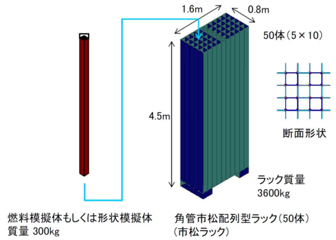
(2) 市松ラック (供試体) [2]
