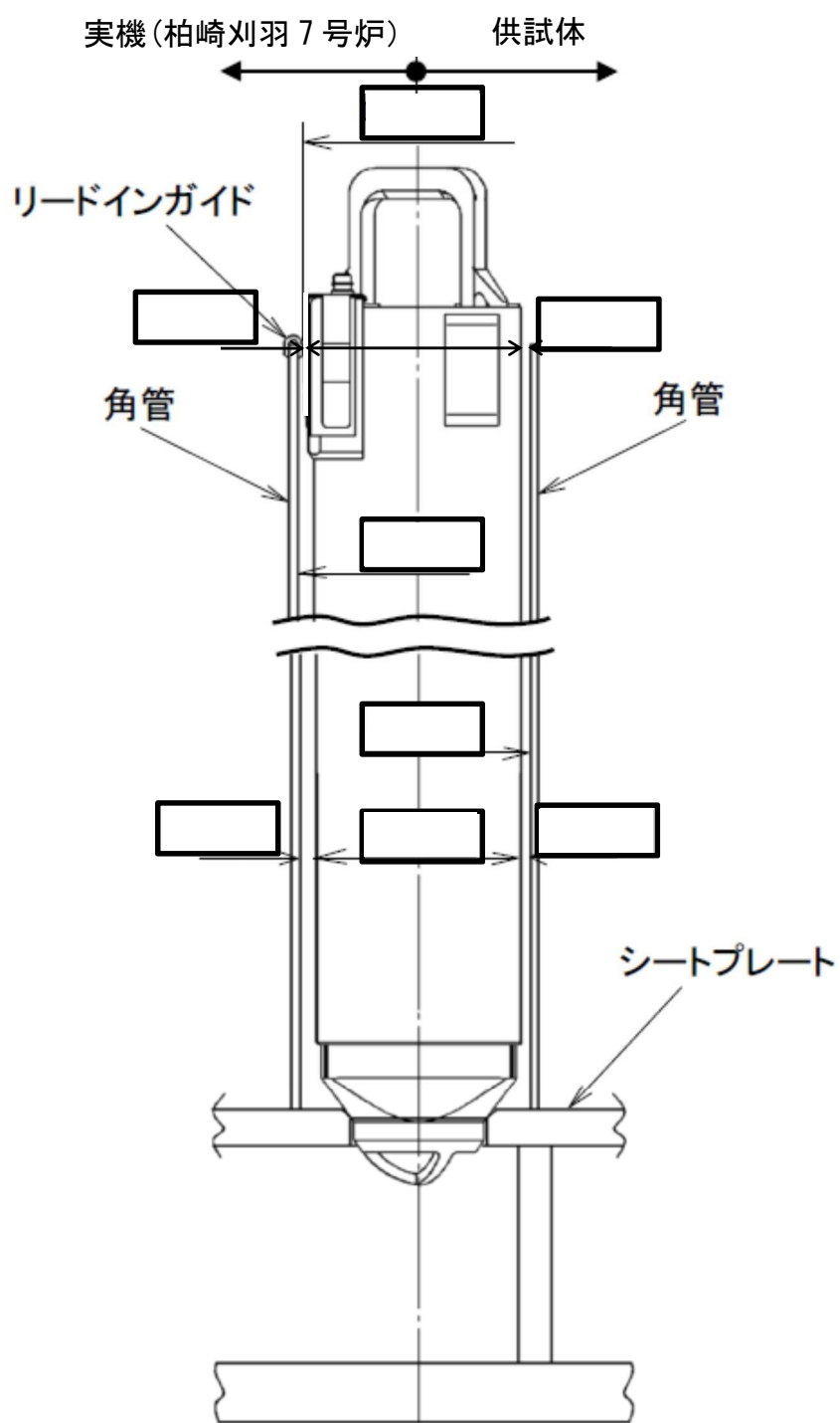
図 1 1 ラックセルと燃料集合体の隙間 (概念図)
