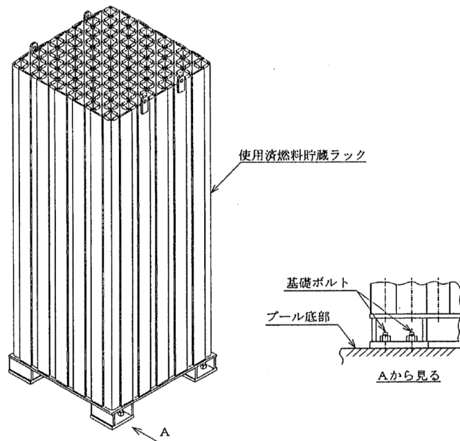
図 5 燃料プール床と固定部の詳細
