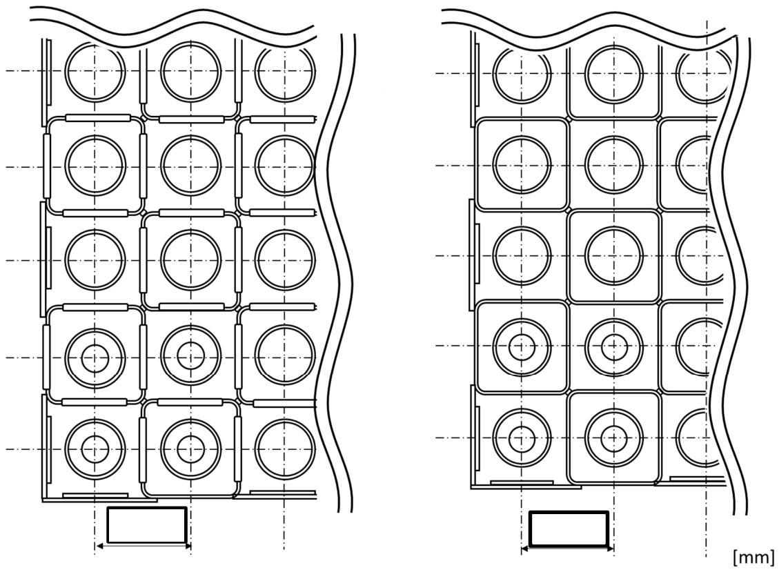
柏崎刈羽 7号炉 供試体 図12 ラックセルのピッチ (概念図)
