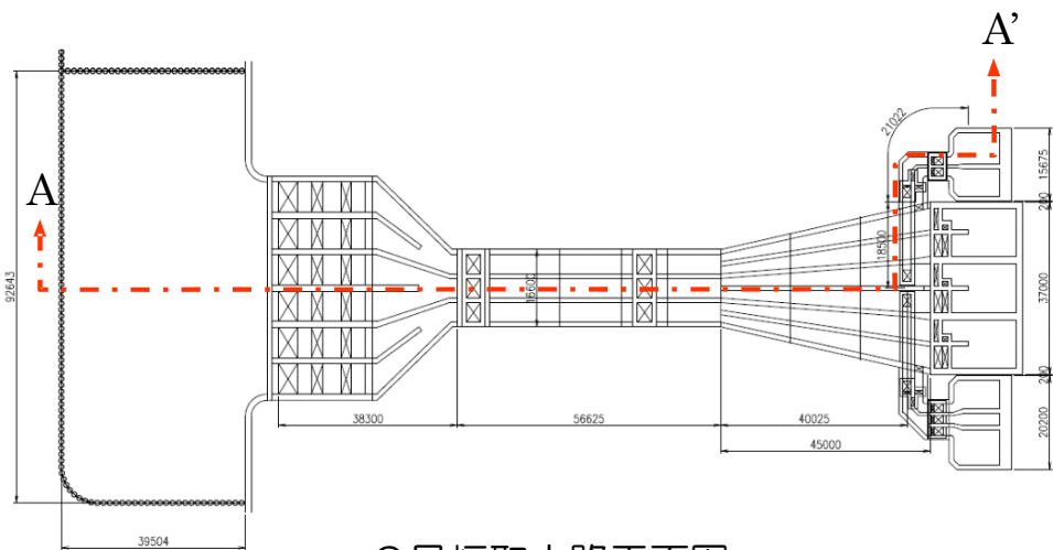
6号炉取水路平面図
