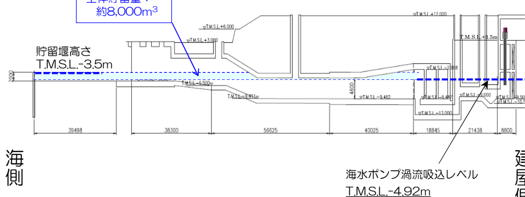
7号炉取水路 B-B'断面図
