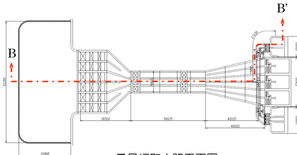
7号炉取水路平面図
