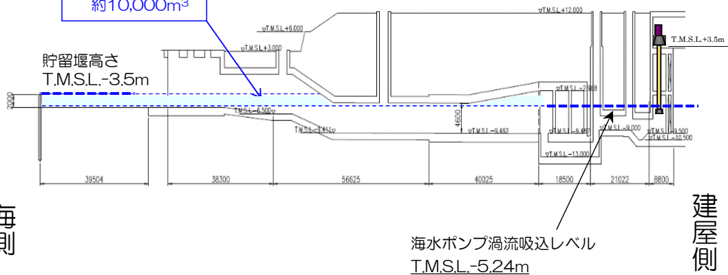
6号炉取水路 A-A'断面図
