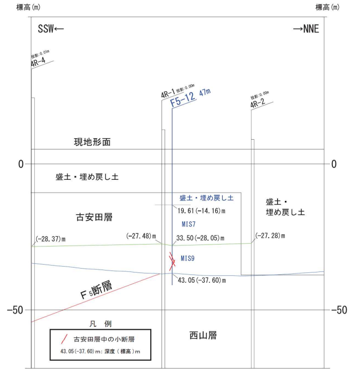
地質断面図
