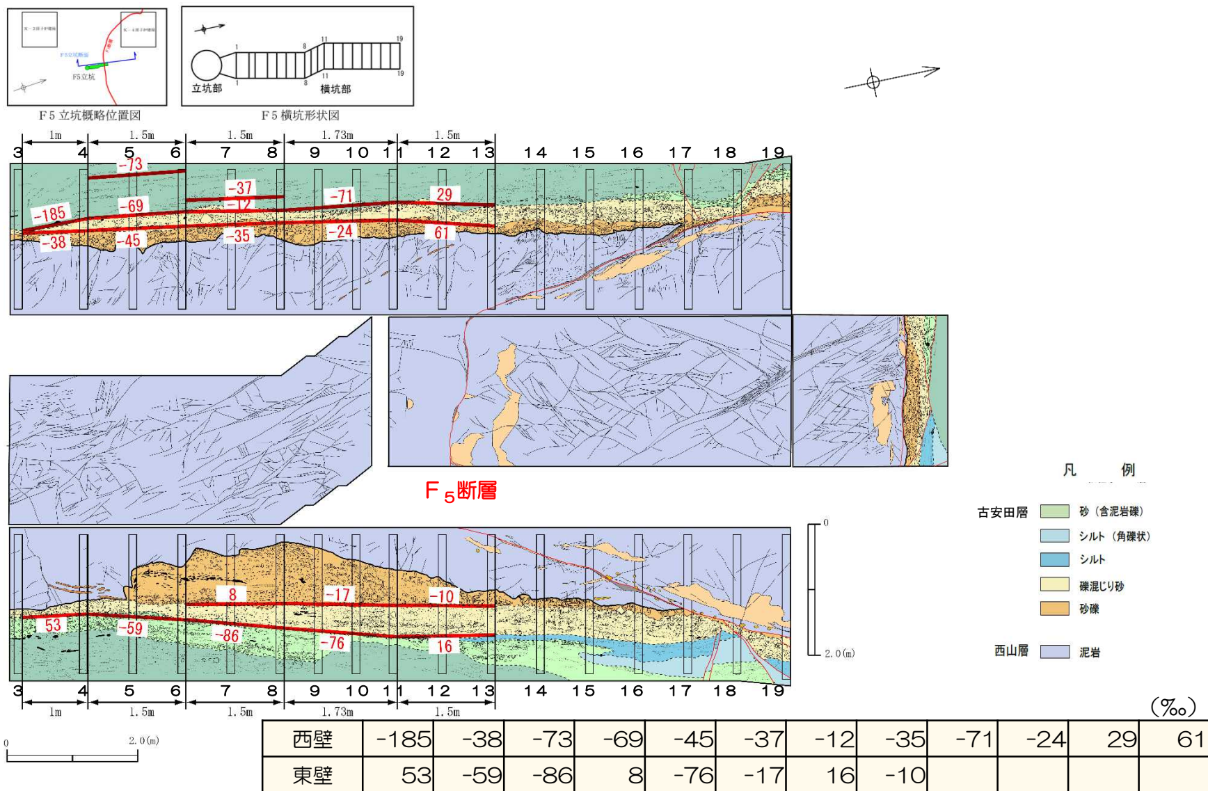
F5立坑横坑部における古安田層の勾配（絶対値） 最大値185%，最小値8%，平均値50.2%
