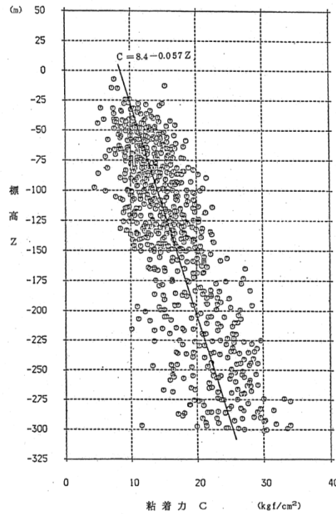
西山層 (泥岩) の粘着力 [高圧部]
