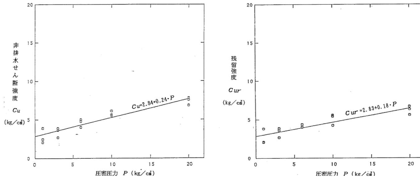
F 3 断層（破碎部）のせん断強度及び残留強度 ※F系断層は、粘土部と破碎部の強度の低い方を用いる。
