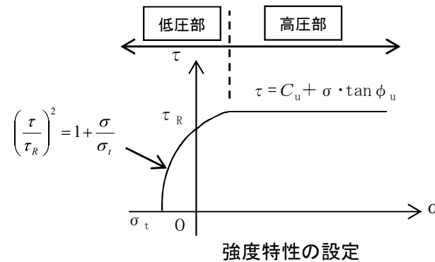
西山層 (泥岩) の粘着力 [高圧部]
