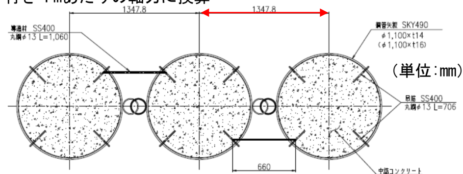
詳細平面図
