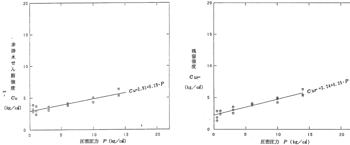
F 3 断層（粘土部）のせん断強度及び残留強度
