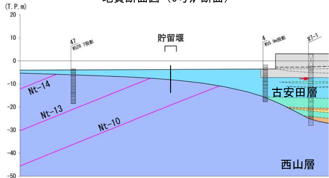
地質断面図 (7号炉断面)
