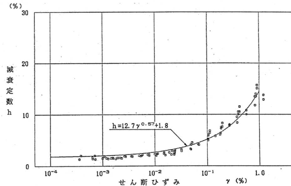
3V-1断層の動的変形特性
