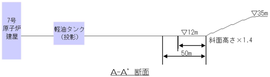
第2図 抽出された周辺斜面（6, 7号炉経由タンク周辺斜面） （上段：拡大平面図，下段：A-A'断面図）
