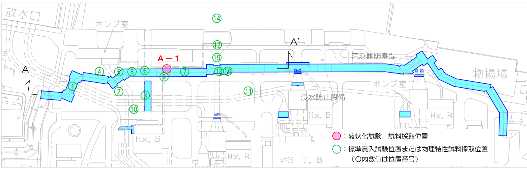
N値及び物理特性の調査位置図：荒浜側 A-1（洪積砂層 I）
