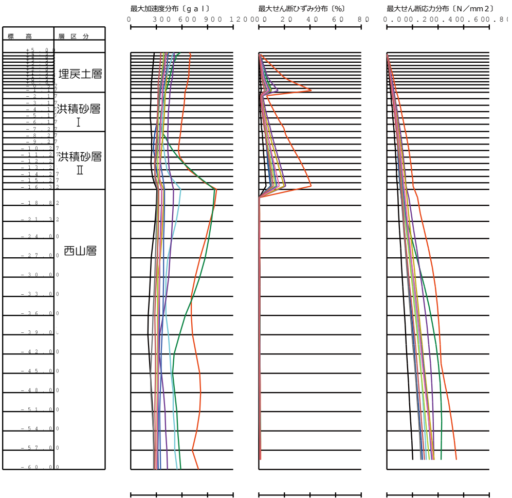
最大応答値分布
