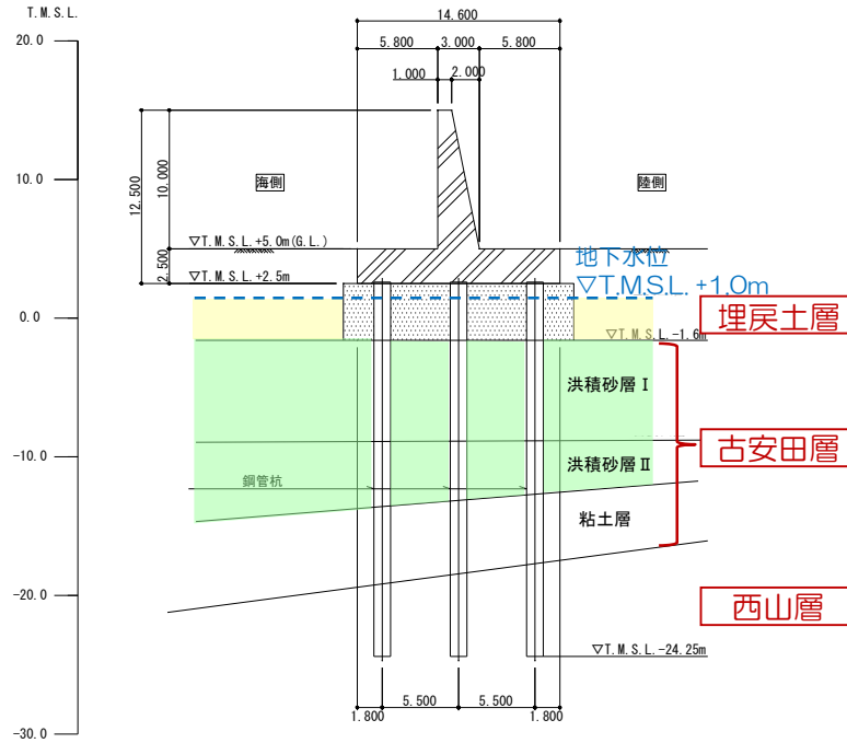
A-A断面
