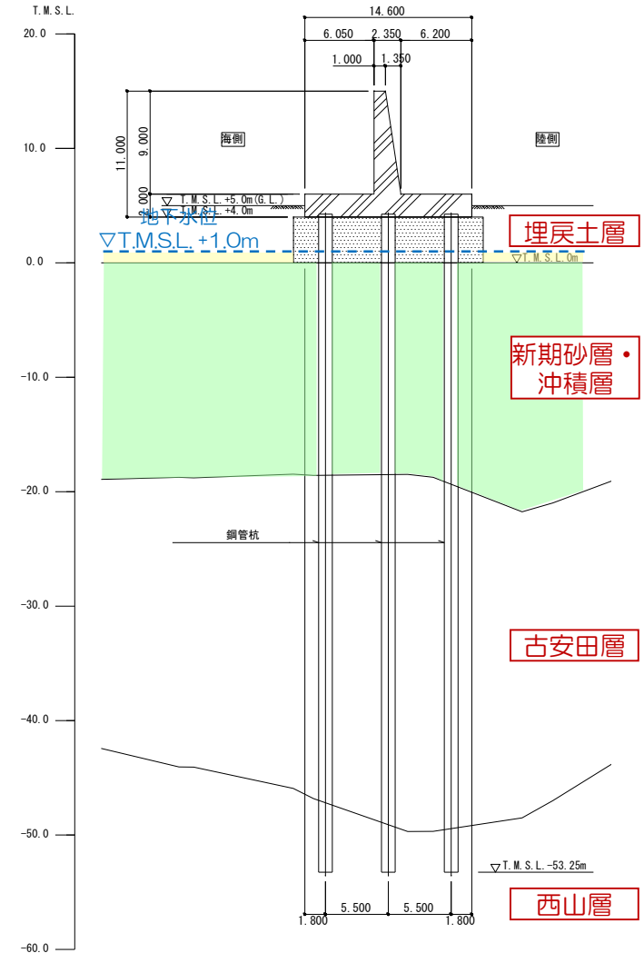
B-B断面
