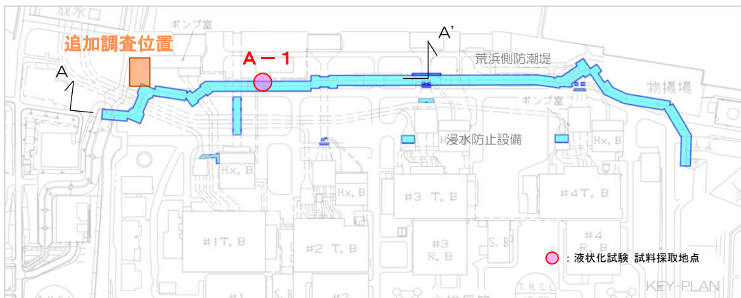
荒浜側 調査位置図
