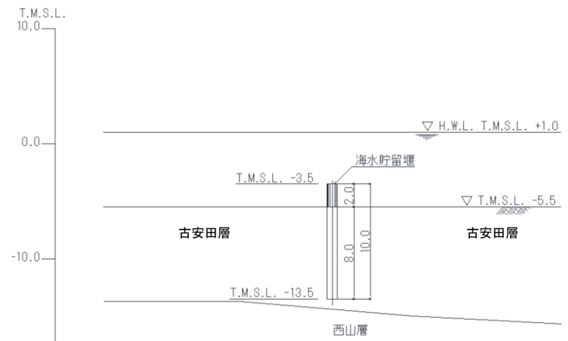
6号炉海水貯留堰断面図 (単位：m)
