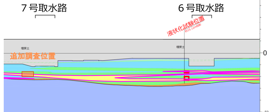
大湊側 地質断面図（6号～7号炉取水路）
