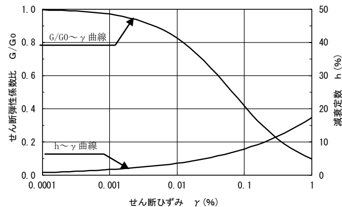
洪積砂層 I, II
