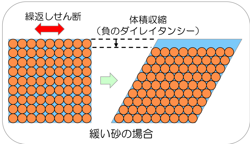
地盤のダイレイタンス特性の概要
