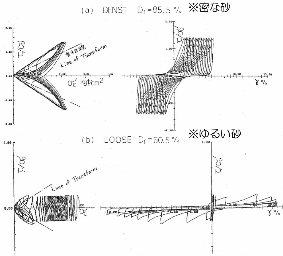
図3-2 密な砂(a)とゆるい砂(b)の中空ねじりせん断試験による有効応力径路(左側)と応力・ひずみ関係 Effective Stress Path and Stress - Strain Curve for Dense Sand (a) and Loose Sand (b)
