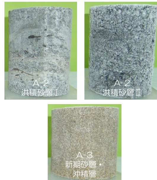
図 試験供試体例 (左上：洪積砂層 I 右上：洪積砂層 II 下：新期砂層・沖積層 )
