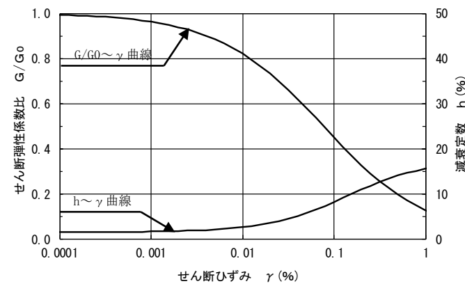
洪積砂質土層 I, II
