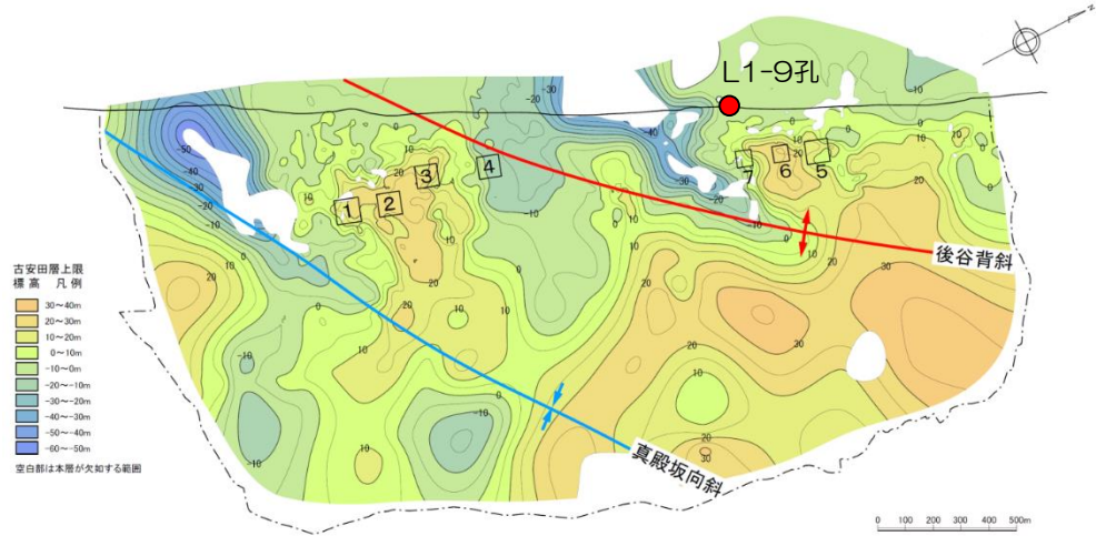
古安田層上限面図
