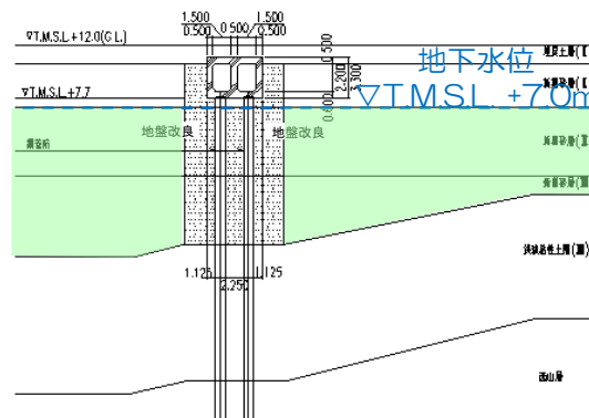
燃料移送系配管ダクト断面図
