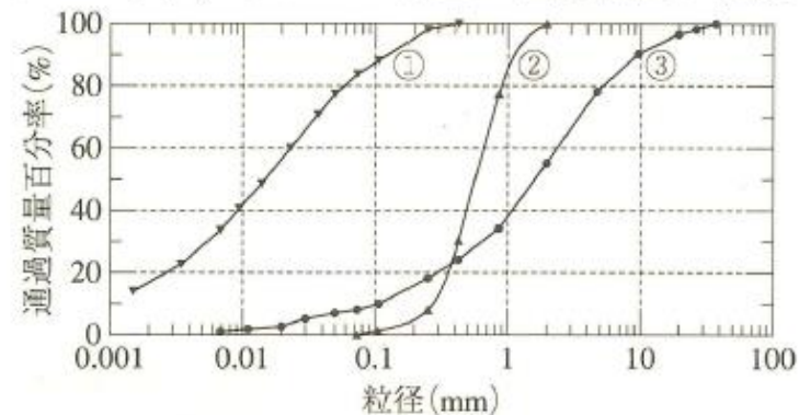
粒径加積曲線の例
