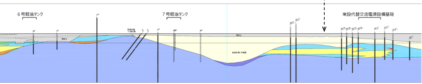
地質断面図 ① - ①' 断面
