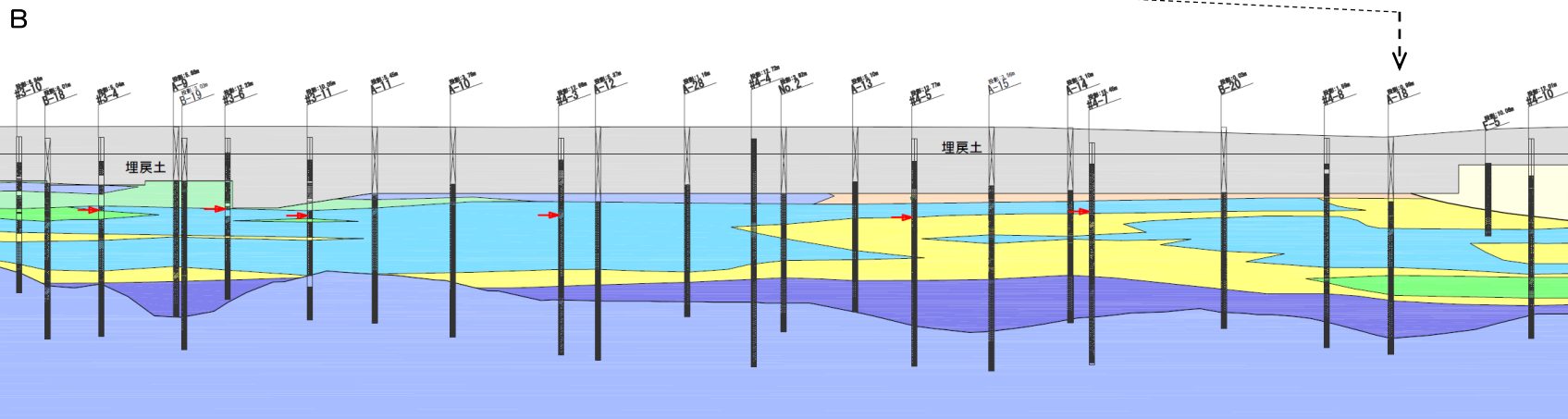
荒浜側防潮堤地質縦断面図 ① - ①' (A~B) 断面
