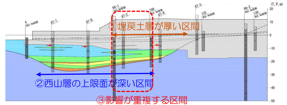
7号炉取水路縦断図（B-B' 断面）
