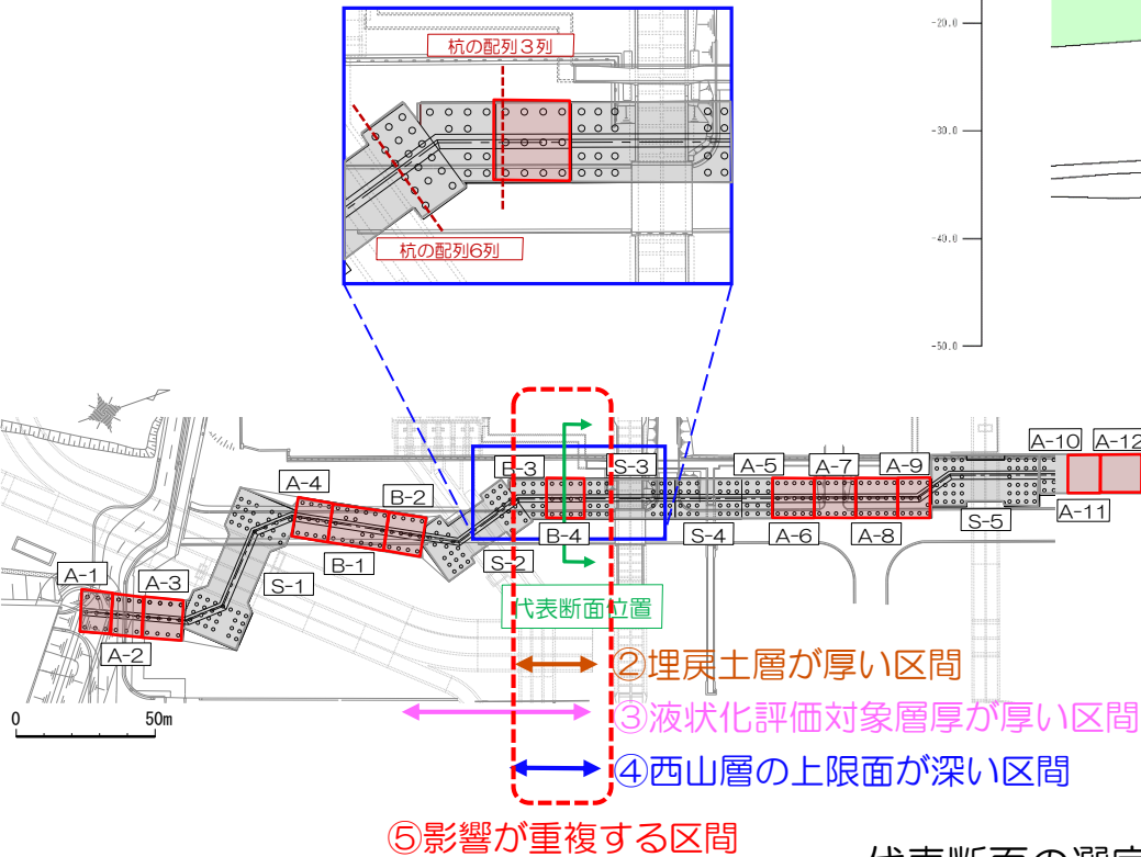
代表断面の選定（荒浜側防潮堤）
