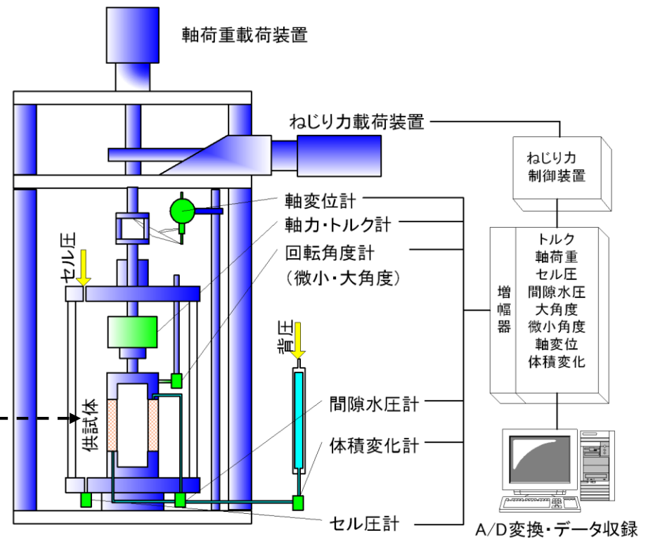
中空ねじり試験機の概要
