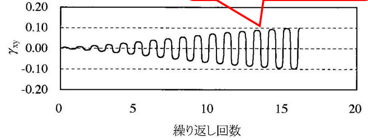
(c) せん断ひずみ 2)
