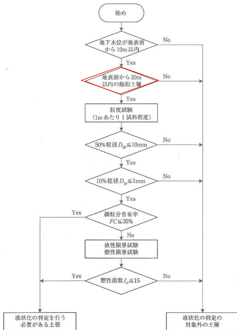
図-解8.2.1 液状化の評価を行う必要がある土層の評価の手順
