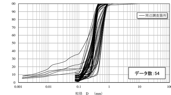
粒径加積曲線（大湊側）
