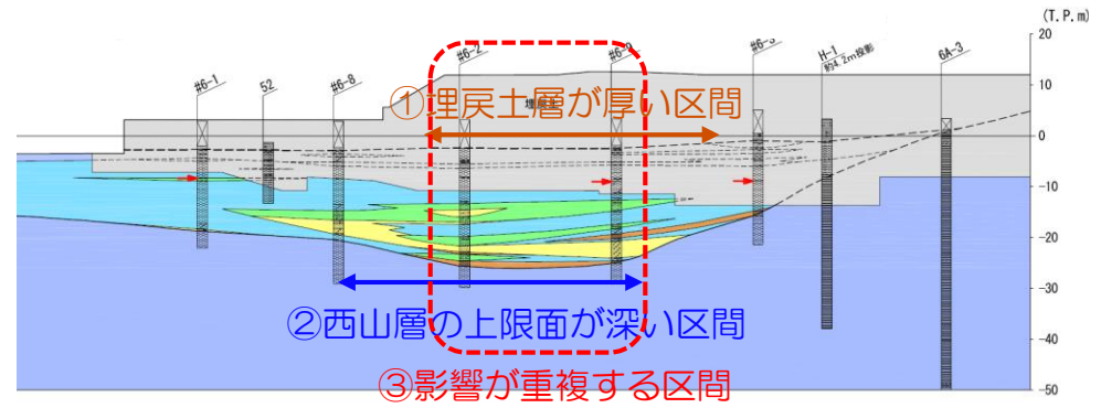
TEPCO 6号炉取水路縦断図（A-A' 断面）
