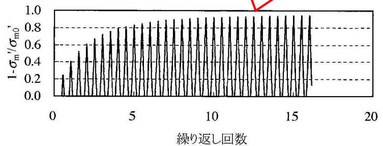
(d) 過剰間隙水圧比 2)
