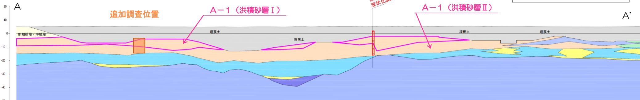
荒浜側 地質断面図
