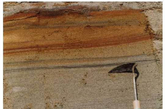
1号海水機器建屋南側法面 T.M.S.L. -5m~-7m 古安田層砂質土 (地点②)
