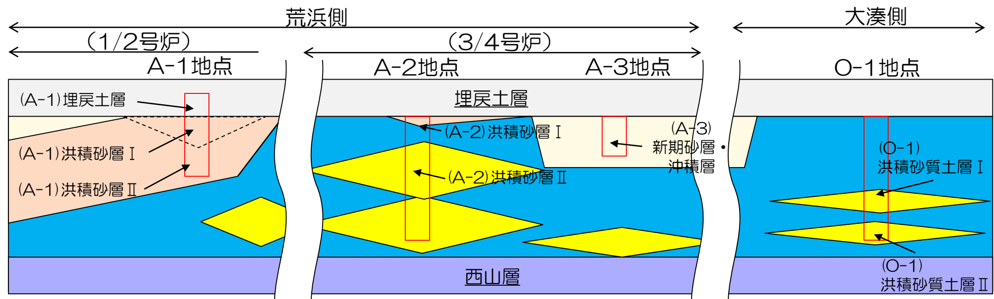
地質断面の概要と調査位置の概要
