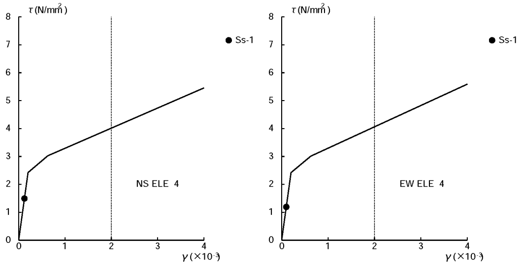
図 3.3-6 せん断スケルトン曲線上へのプロット(1F)
