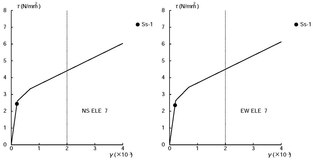
図 3.3-9 せん断スケルトン曲線上へのプロット(B3F)
