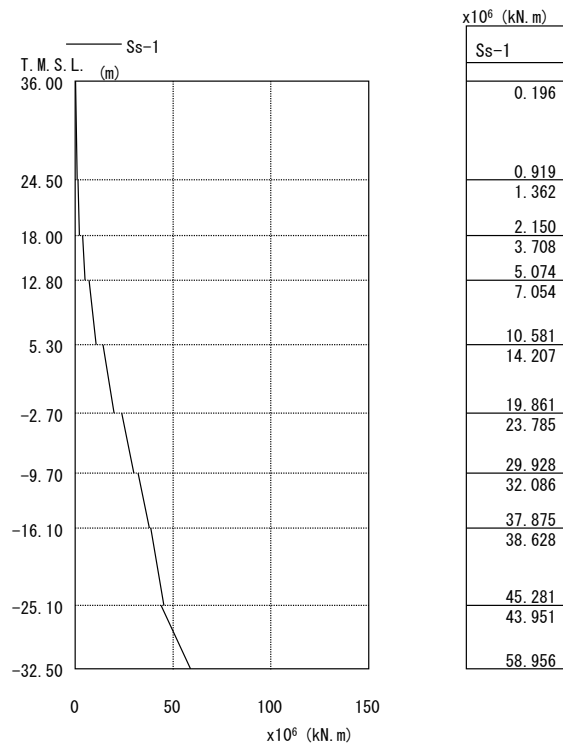
図 3.2-5 最大応答曲げモーメント NS 方向
