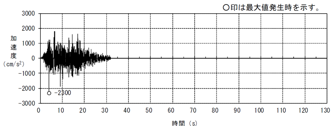
図 3.1-1 加速度時刻歴波形(基準地震動 Ss-1H)
