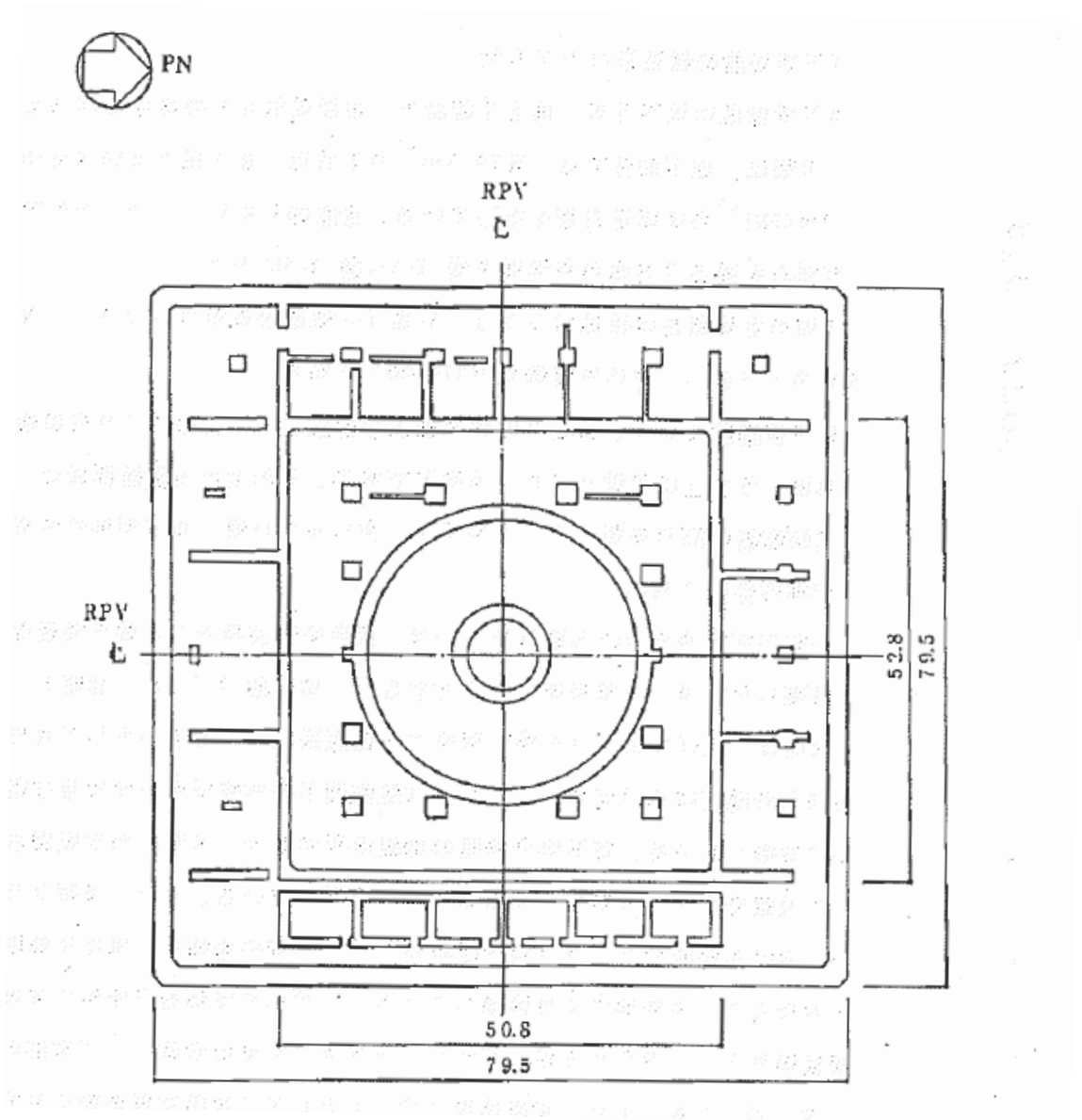
图 2.1-1 建屋概略平面图
