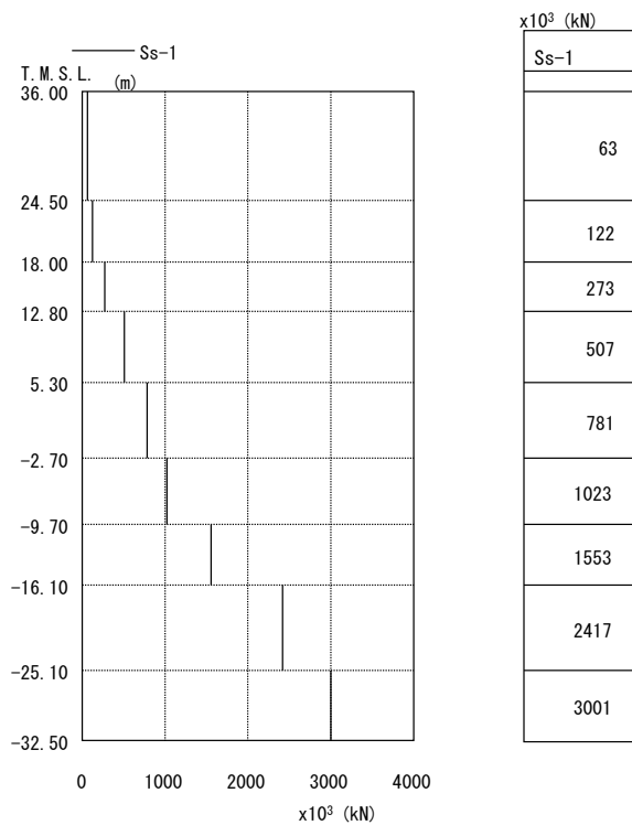
図 3.2-3 最大応答せん断力 NS 方向
