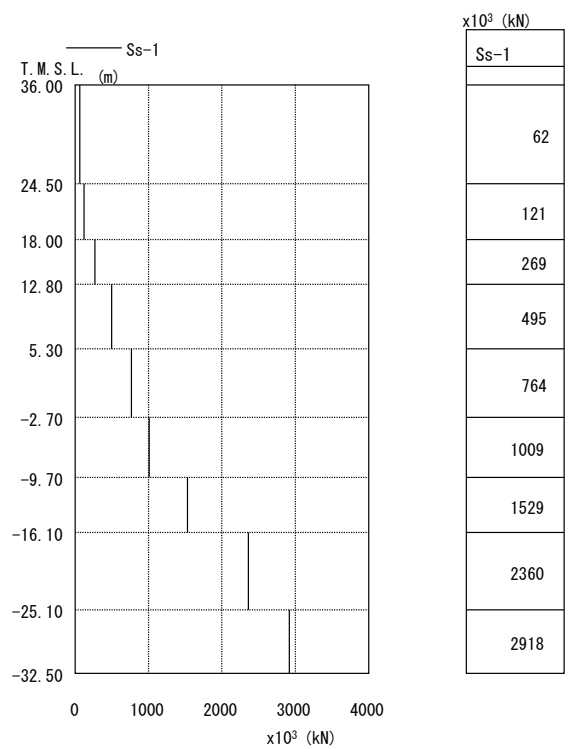
図 3.2-4 最大応答せん断力 EW 方向
