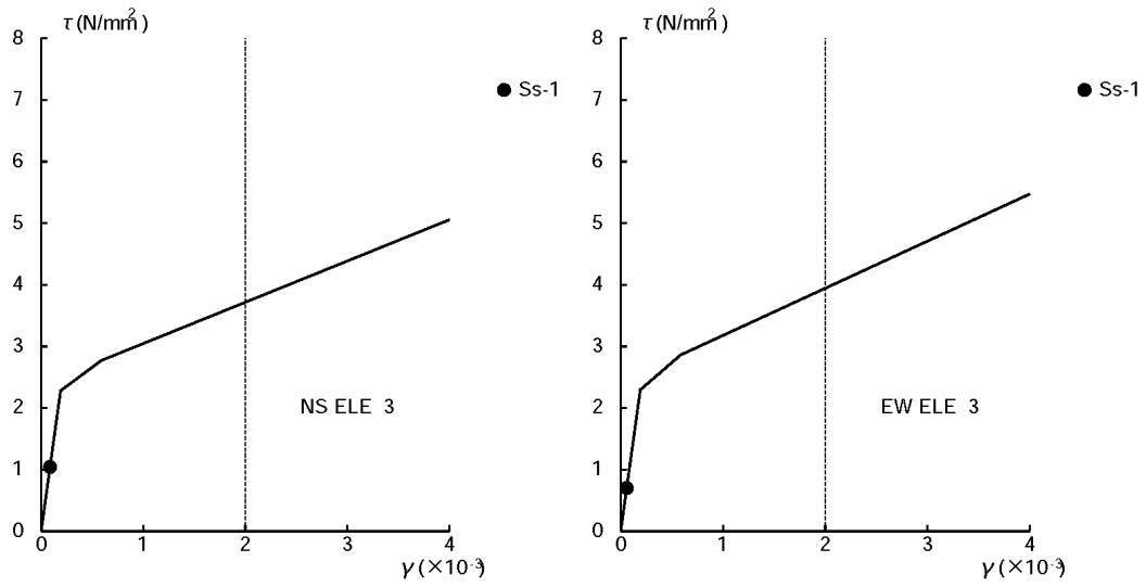
図 3.3-5 せん断スケルトン曲線上へのプロット (2F * )
