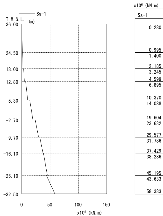
図 3.2-6 最大応答曲げモーメント EW 方向
