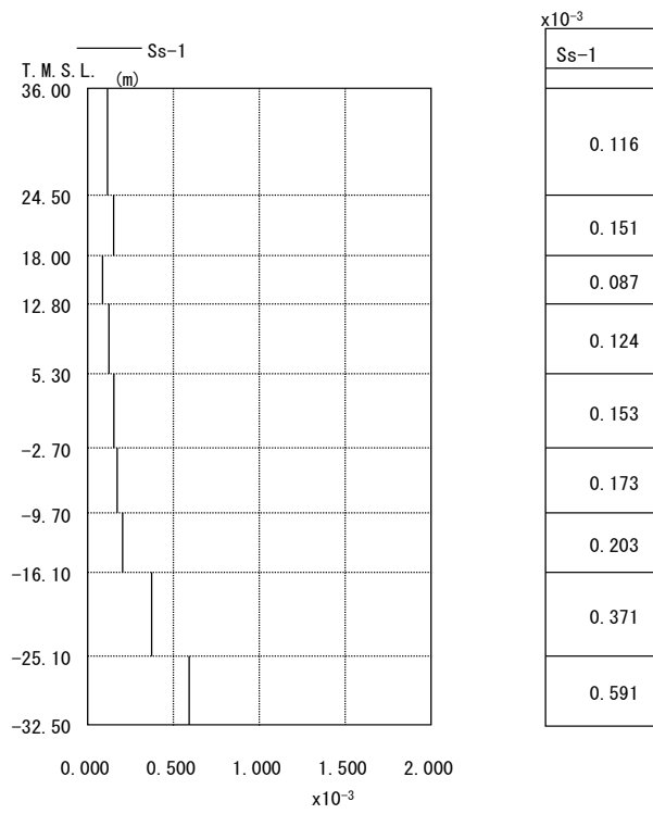
図 3.3-1 最大応答ひずみ NS 方向
