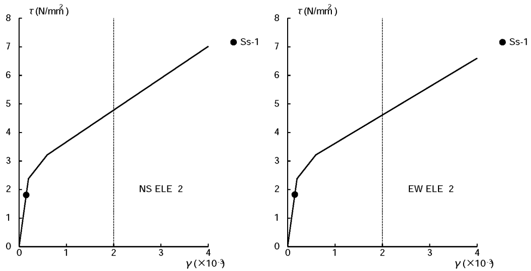
図 3.3-3 せん断スケルトン曲線上へのプロット (CRF)
