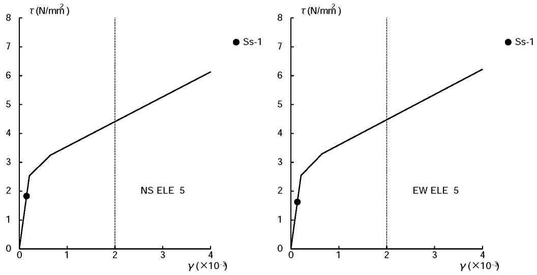
図 3.3-7 せん断スケルトン曲線上へのプロット (B1F)
