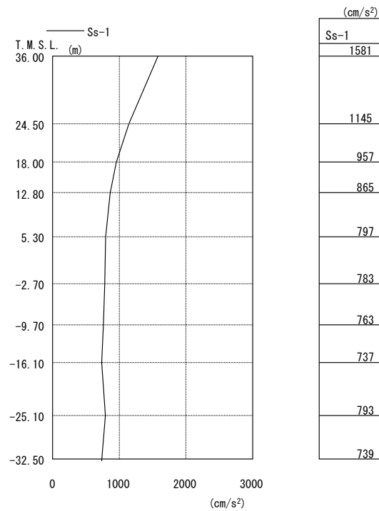
図 3.2-2 最大応答加速度 EW 方向
