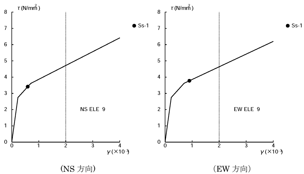
図 3.3-10 せん断スケルトン曲線上へのプロット(B5F)
