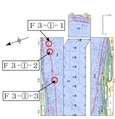
F 3立坑 横坑部地質展開図
