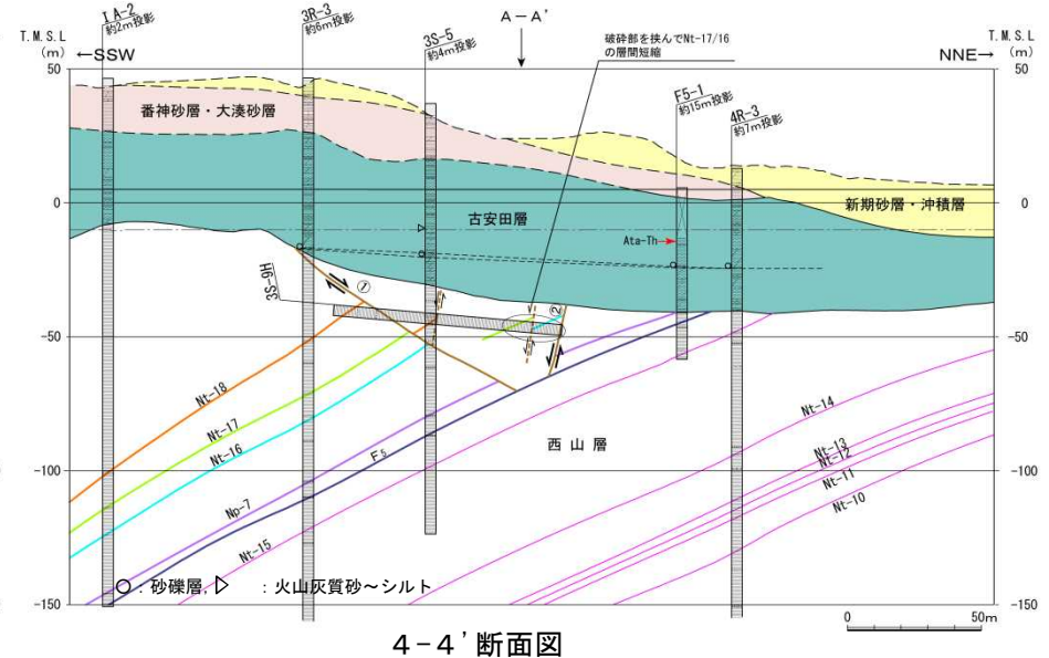
4-4' 断面図
