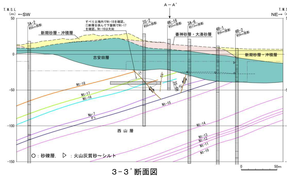
3-3' 断面図
