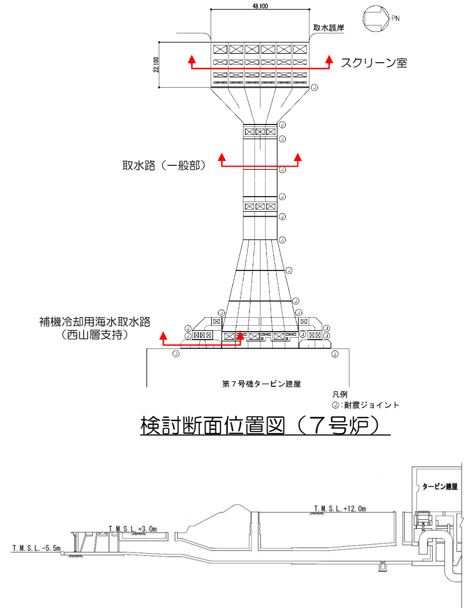
<参考> 取水路縦断図（7号炉）
