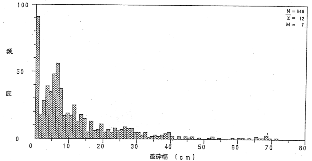
F 3 断層（破碎部）の層厚
