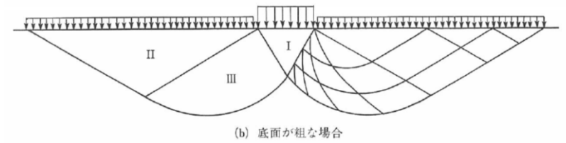
図 10.10 一般的なすべり面の形状
