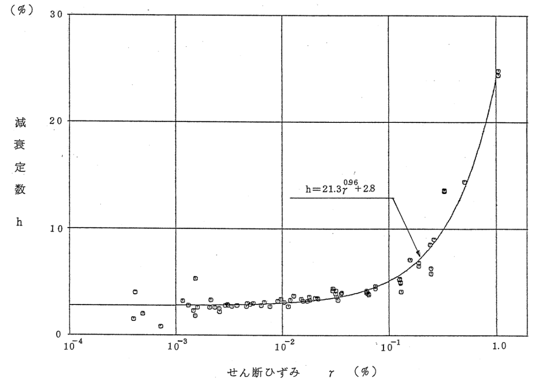
F 5 断層 (粘土部) の動的変形特性
