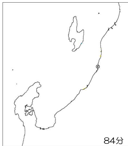
■二層流モデルに基づく手法による津波水位の経時変化 SD-2,3同時 (80分~90分)
