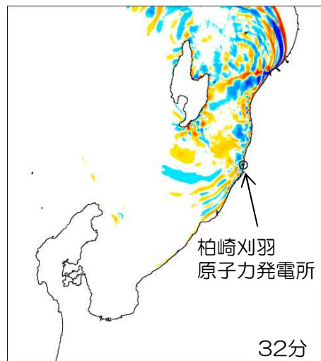
■二層流モデルに基づく手法による津波水位の経時変化 SD-5 (32分~46分)
