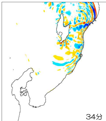
■二層流モデルに基づく手法による津波水位の経時変化 SD-5 (32分~46分)
