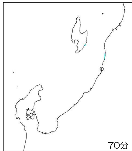
■二層流モデルに基づく手法による津波水位の経時変化 SD-2,3同時 (64分~78分)
