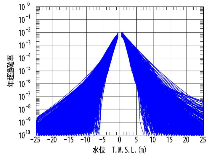
2,000本のハザード曲線（1号炉取水口前面）
