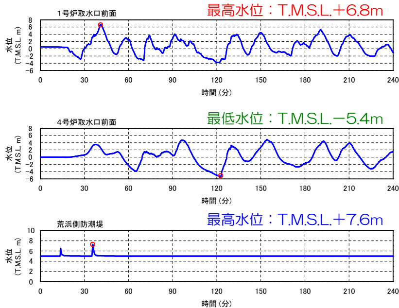
時刻歴波形（上：取水口前面上昇側，中：取水口前面下降側，下：荒浜側防潮堤）
