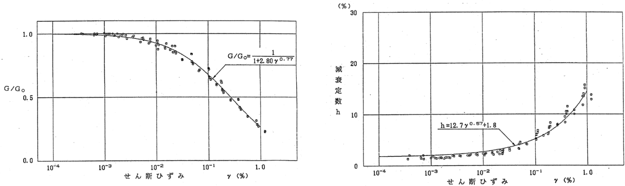
3V-1断層の動的変形特性
