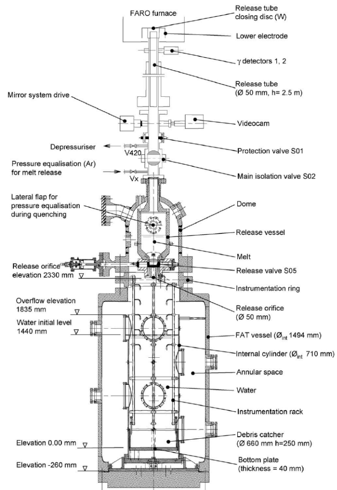
図 4.1.1 FARO 試験装置 [9][10]
