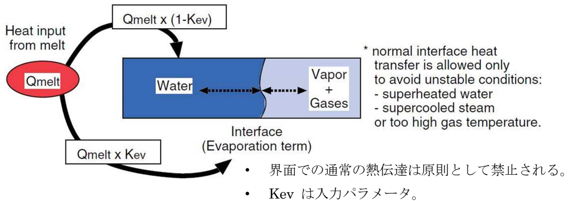
(b) 細粒から二相流への伝熱量分配機構
