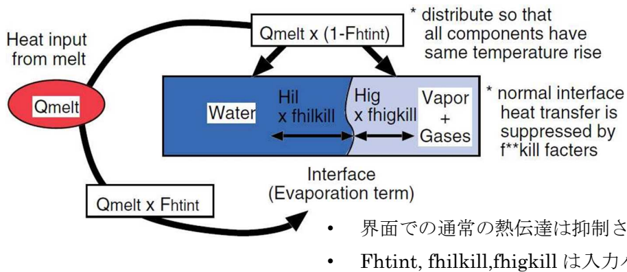
(a) 融体粒子から二相流への伝熱量分配機構 [1]
