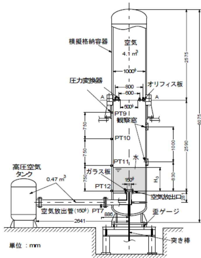
添付図1 水撃実験装置 (大型容器) (稲坂ら, 2004)
