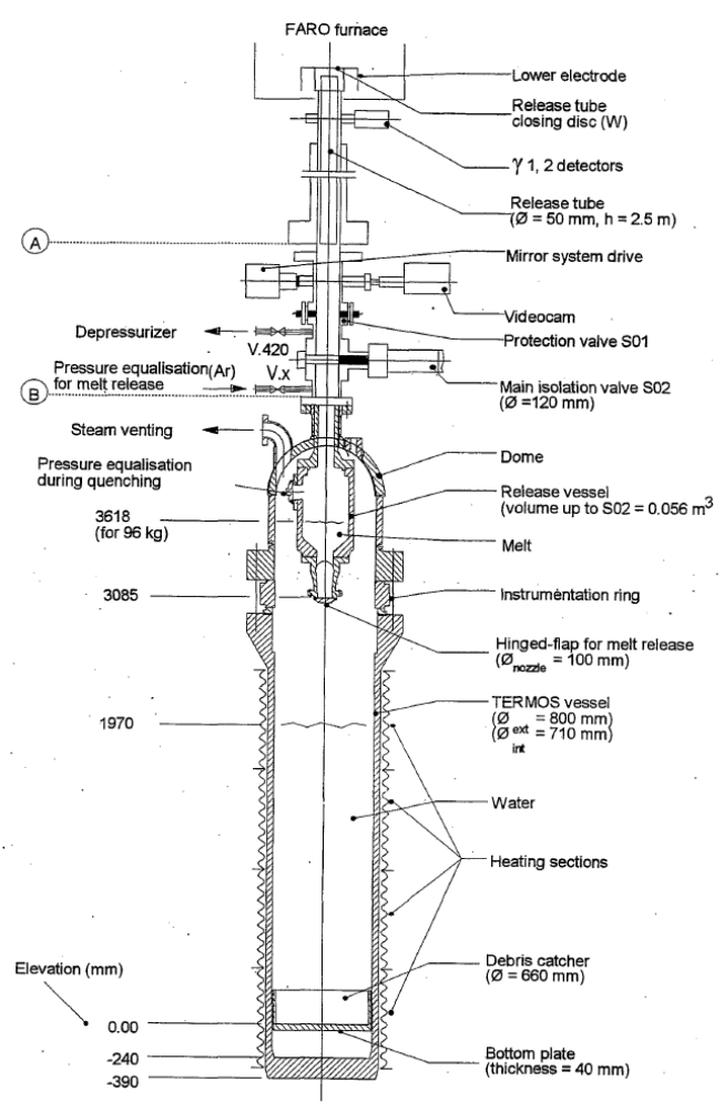
図 4.1.1 FARO 試験装置 [9][10]
