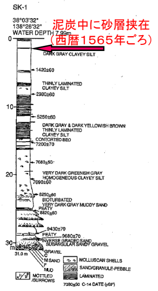
図7. ボーリング柱状図（佐渡島加茂湖、SK-1） 斎藤ほか（1997）を編集
