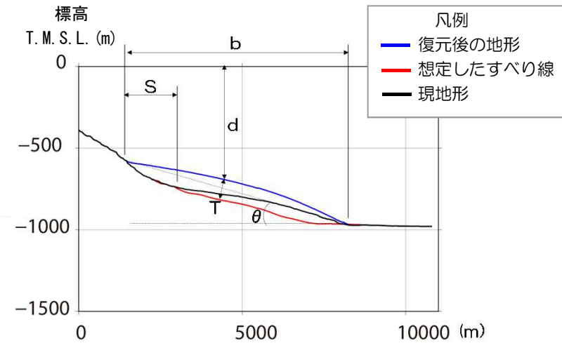
LS-2 地すべり地形断面図
