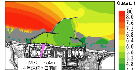
水位分布図（左：取水口前面上昇側，右：取水口前面下降側）
