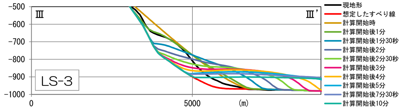
地すべり面と現地形、各時刻における土砂層厚の比較
