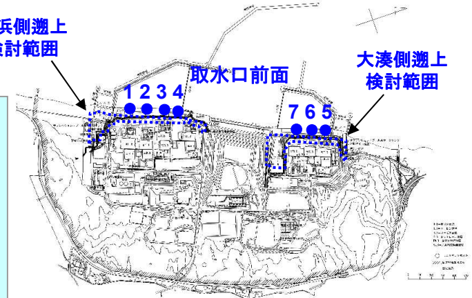
取水口前面における最高水位及び最低水位（地震による津波に潮位を重ね合わせ）
