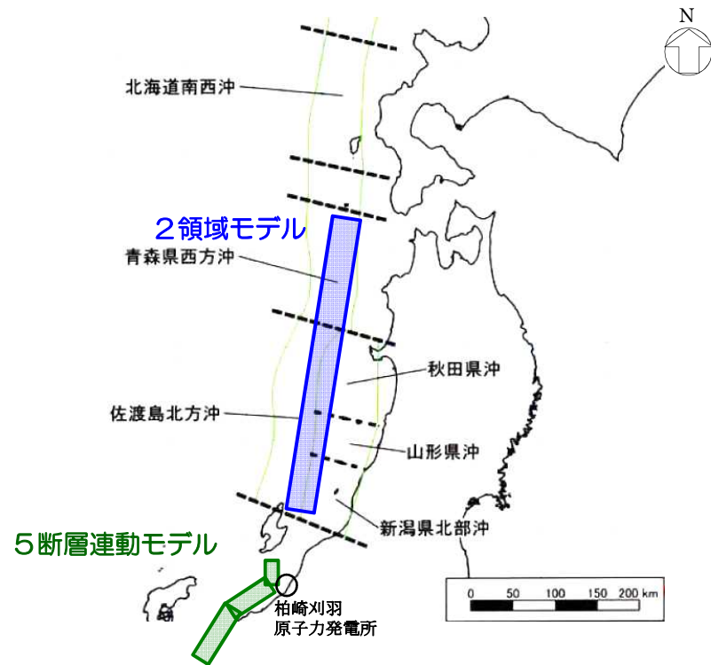
基準津波の想定波源図
