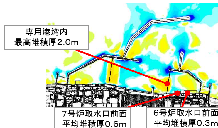
水位上昇側・日本海東縁部
