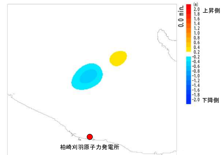
初期水位変動量分布
