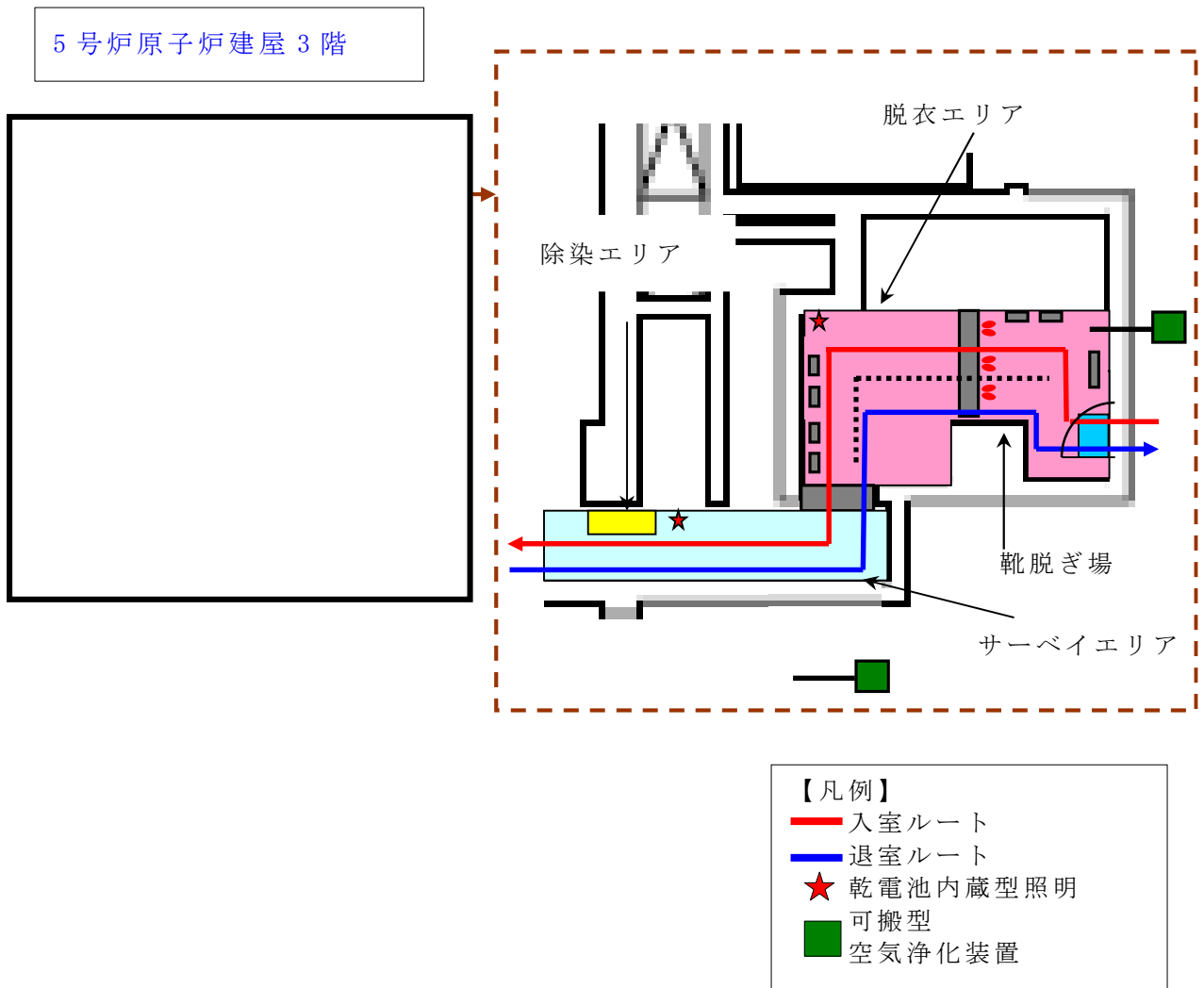
図 5.1-2 5号炉原子炉建屋内緊急時対策所チェンジングエリアの設営場所及び屋内のアクセスルート
