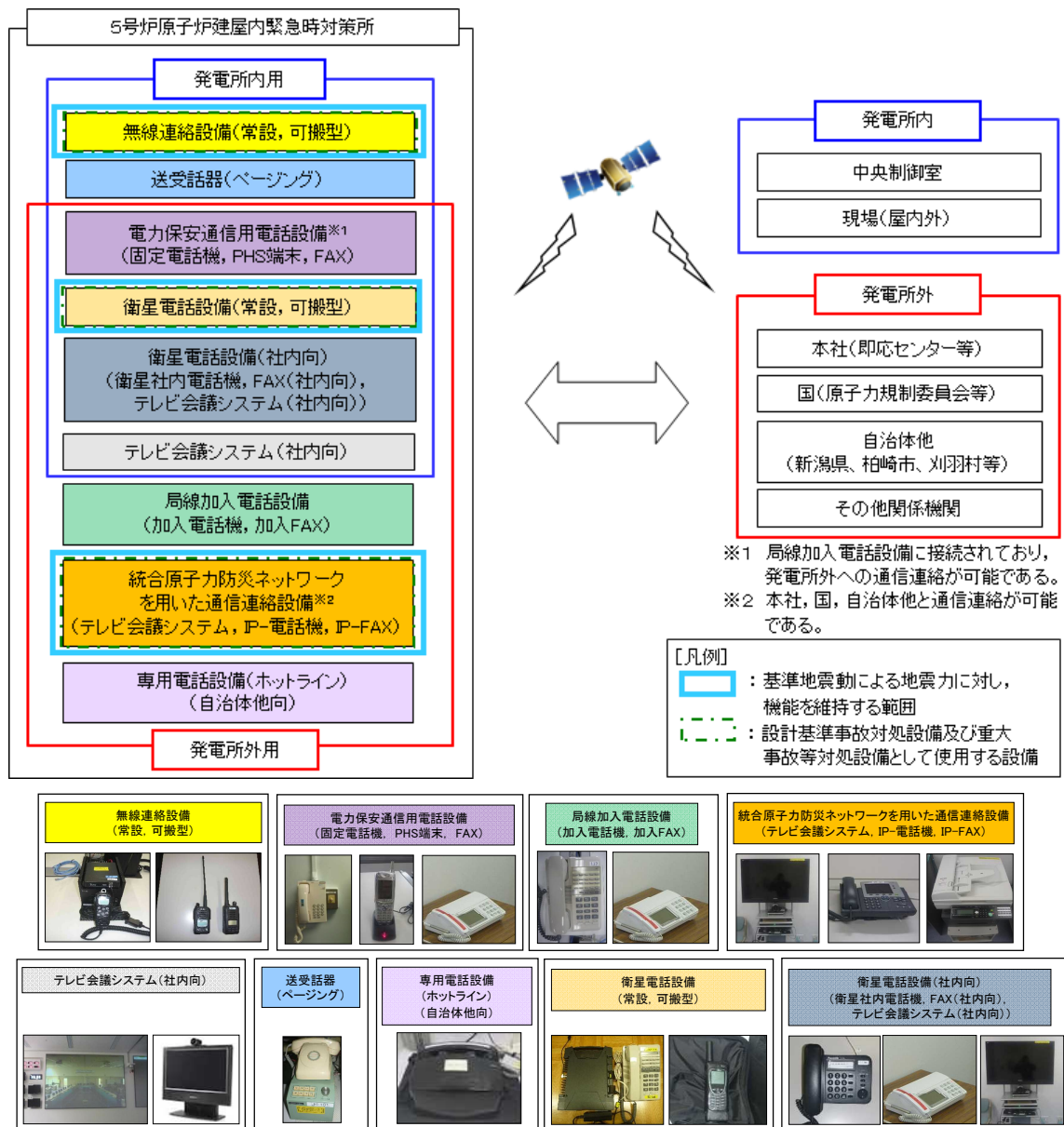
図 2.6-2 5号炉原子炉建屋内緊急時対策所 通信連絡設備の概要
