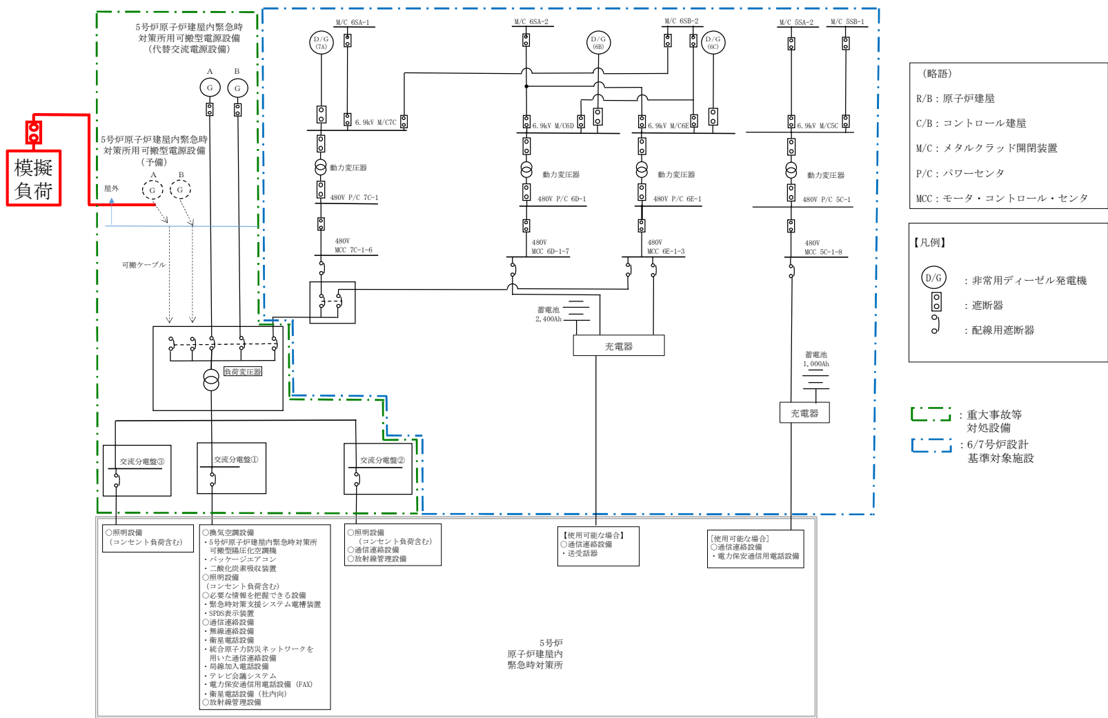
図 61-5-12 5号炉原子炉建屋内緊急時対策所用可搬型電源設備 試験系統図 (模擬負荷による電源設備の出力性能確認)
