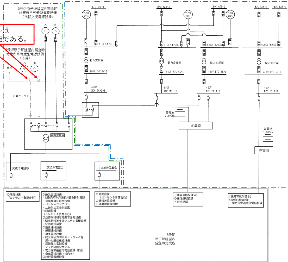
図 61-5-11 5号炉原子炉建屋内緊急時対策所用可搬型電源設備用ケーブル 試験系統図
