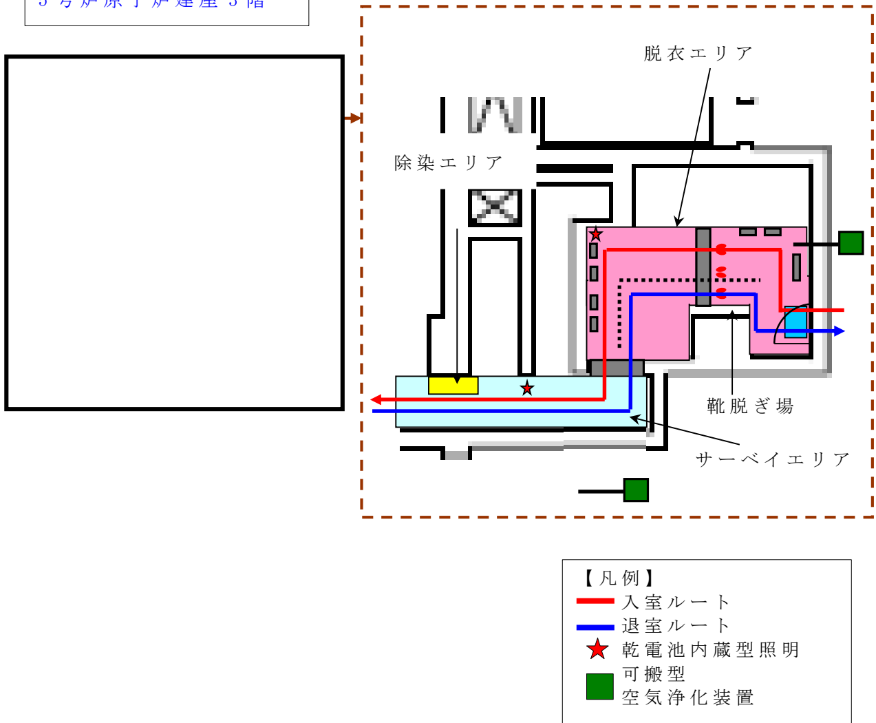
図 3.3-2 5号炉原子炉建屋内緊急時対策所チェンジングエリア 設営場所及び概略図
