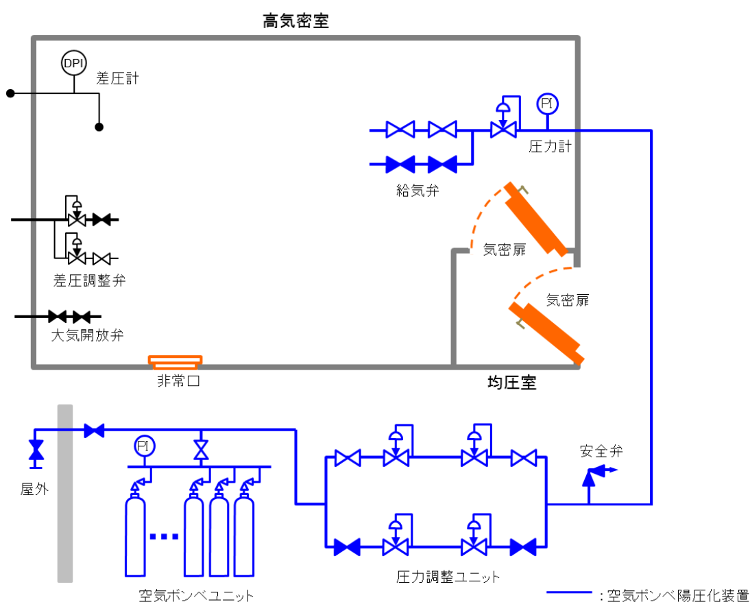
図2.4-17 空気ポンベ陽圧化装置 系統概要図
