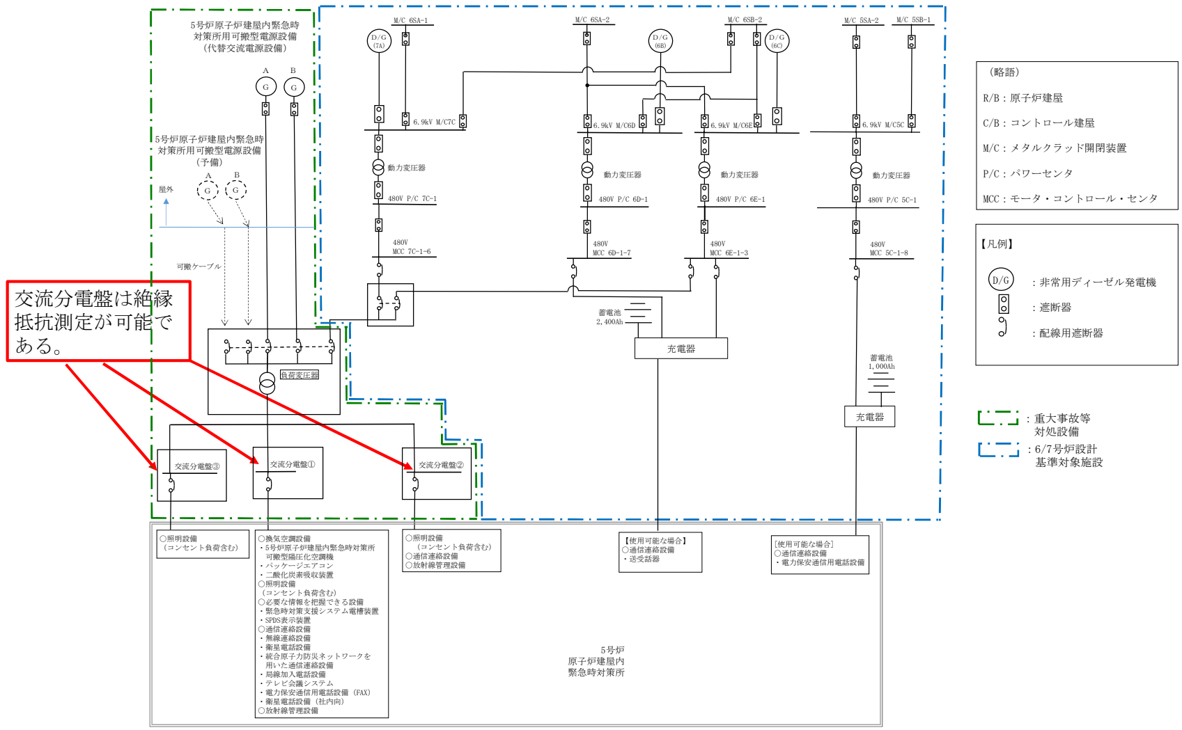
図 61-5-14 交流分電盤 試験系統図
