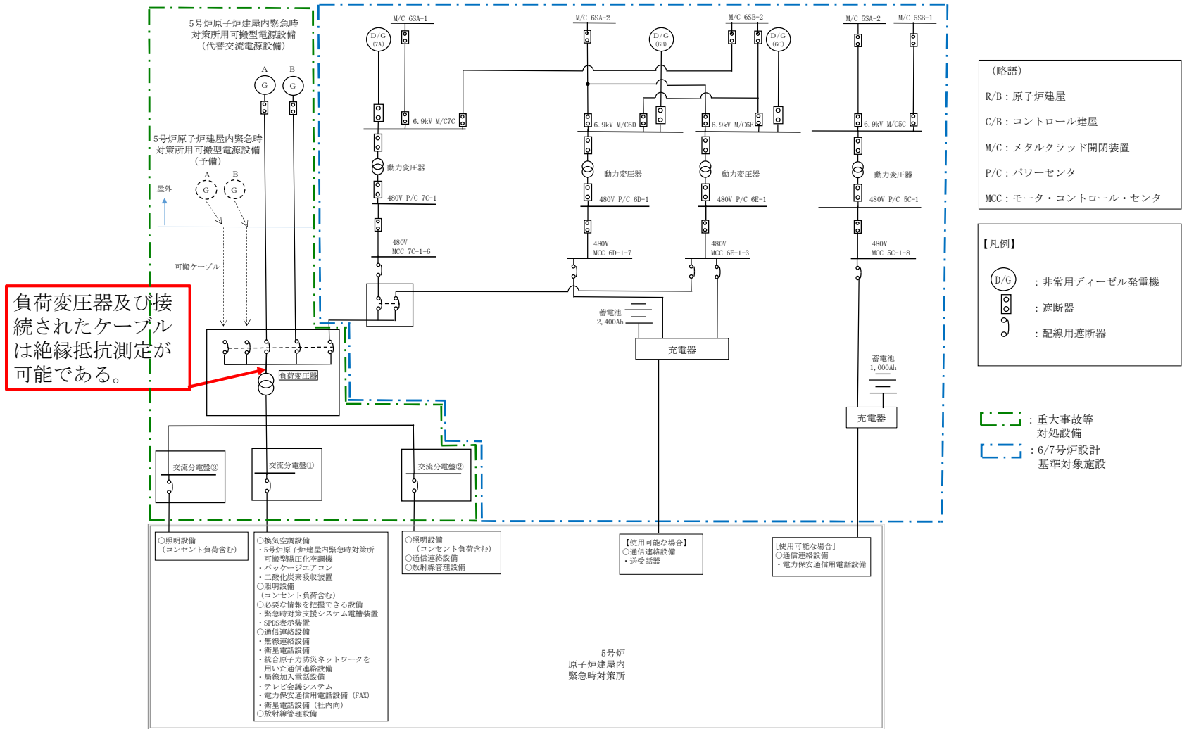
図 61-5-13 負荷変圧器 試験系統図
