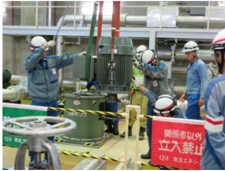
直営による堅型ポンプ用電動機を取替作業
