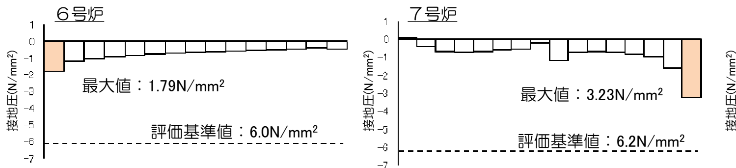
地震時（常時＋地震時増分）の接地圧分布（接地圧最大時刻）
