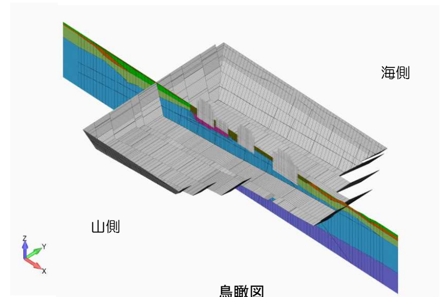
すべり安全率が最小となるケースのすべり面 (立上げ角度:67.5度, 立上げ位置:ケース4)
