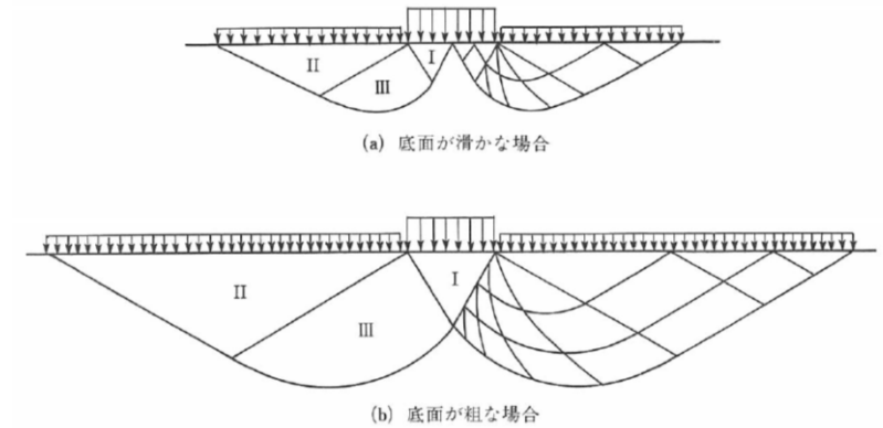
図 10.10 一般的なすべり面の形状
