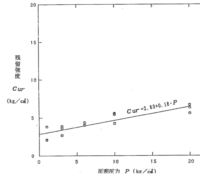
F 3 断層（破砕部）のせん断強度及び残留強度 ※F系断層は、粘土部と破砕部の強度の低い方を用いる。
