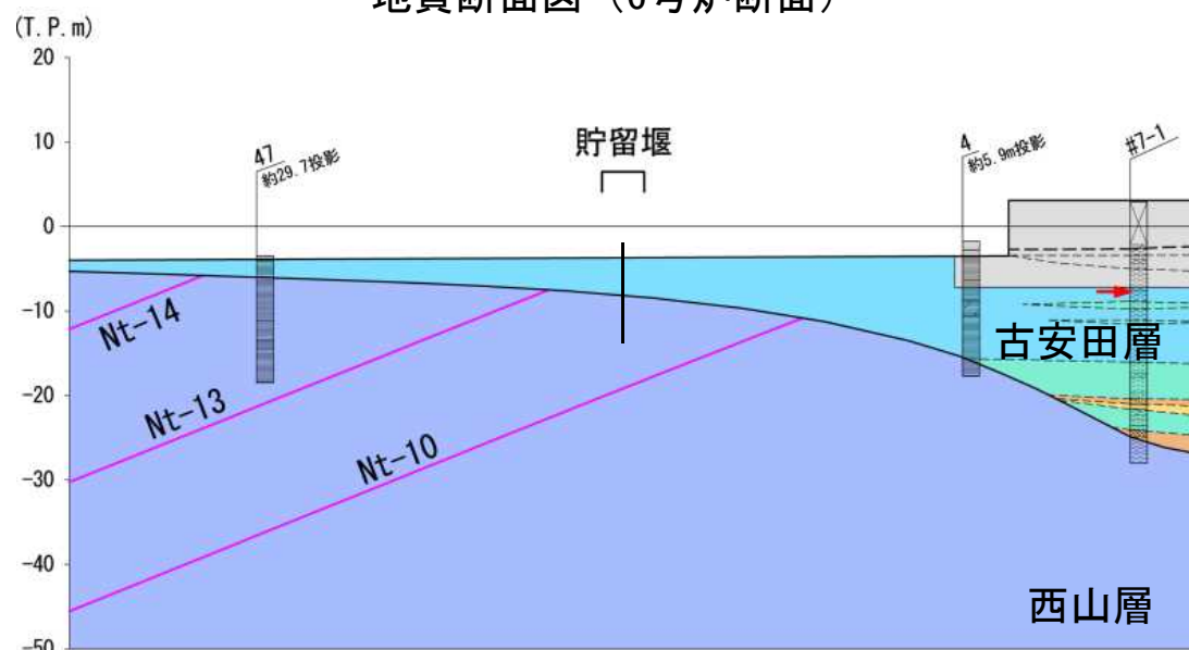
地質断面図 (7号炉断面)
