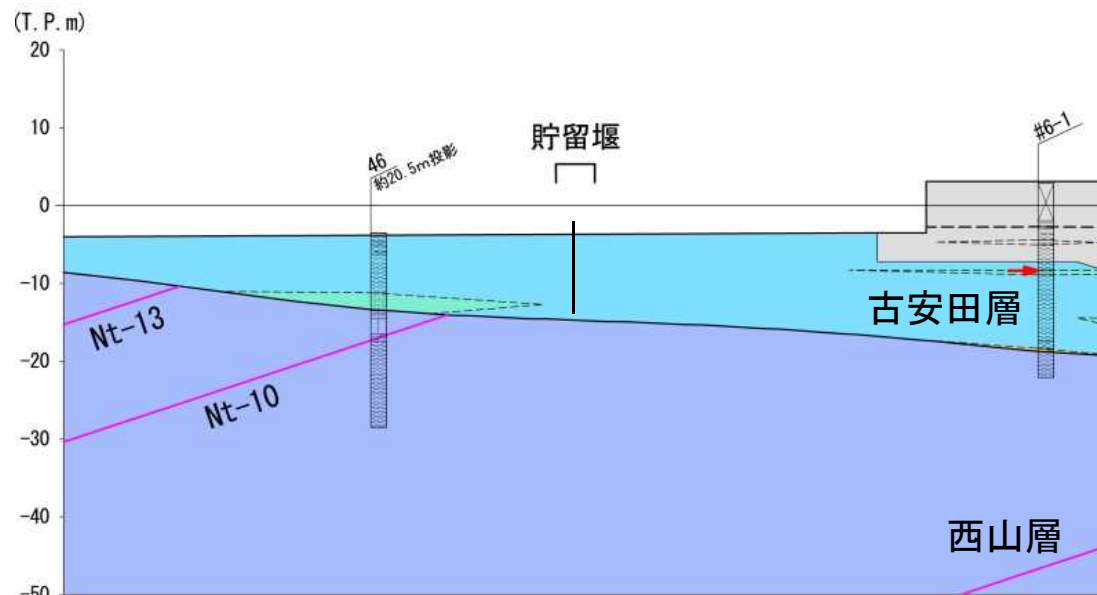
地質断面図 (6号炉断面)
