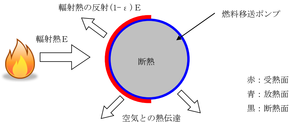
第 2.3.2.3-3 図 燃料移送ポンプ温度評価体系図
