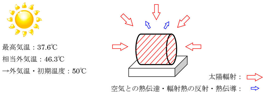
第4図 燃料移送ポンプ温度評価体系図
