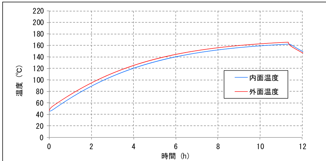
第 5.2.1-3 図 防護扉の外面および内面温度
