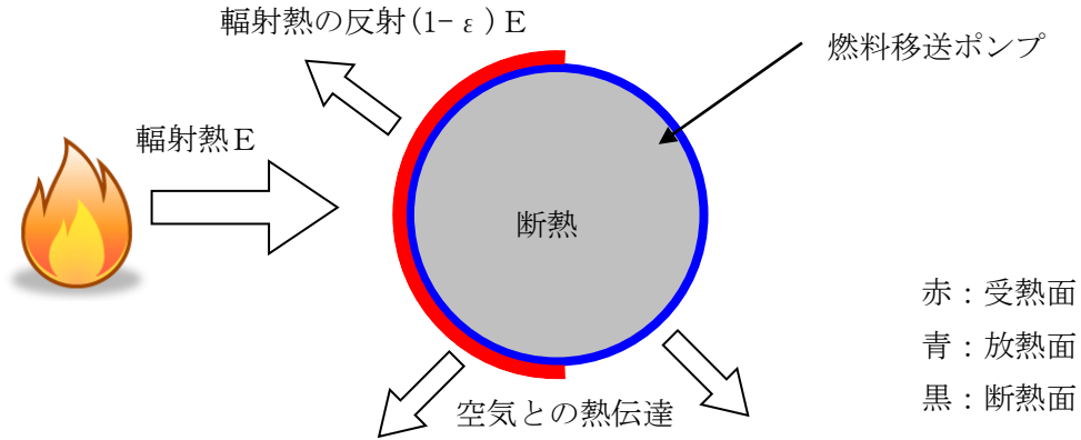
第2.2.2.3-8図 燃料移送ポンプ温度評価体系図
