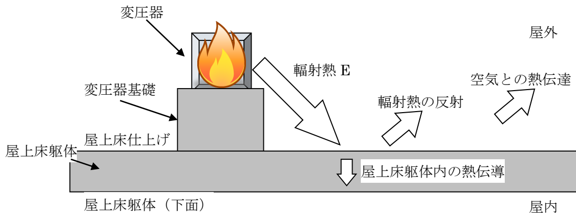
第 3.1.3.2-5 図 建屋屋上への熱影響
