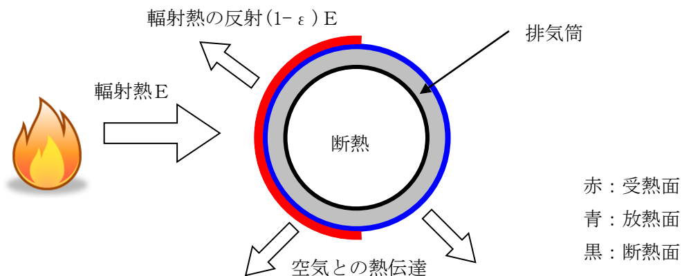
第2.2.2.3-4図 排気筒温度評価体系図
