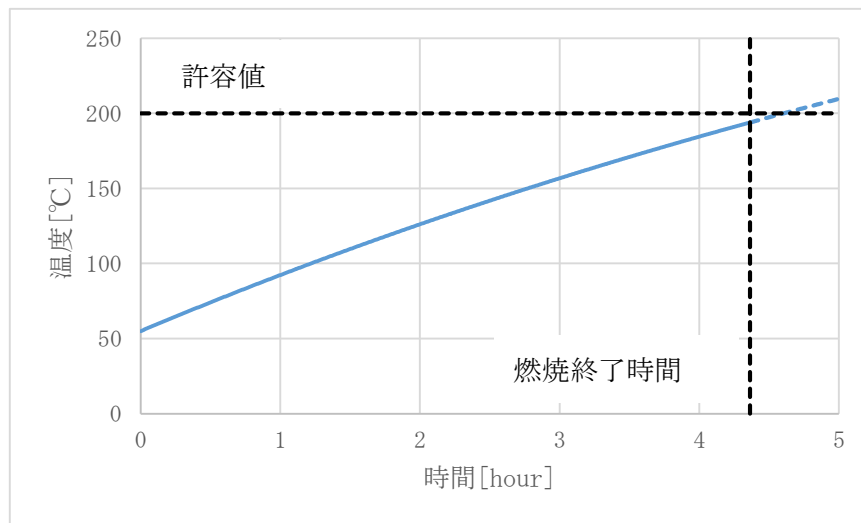
第 3.1.3.1-2 図 変圧器絶縁油温度の推移
