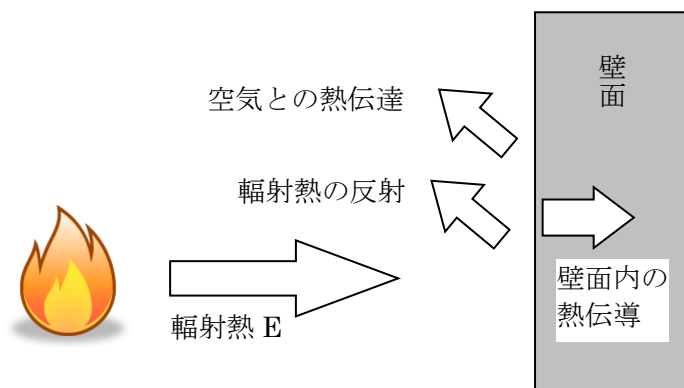
第 2-15 図 建屋温度評価体系図
