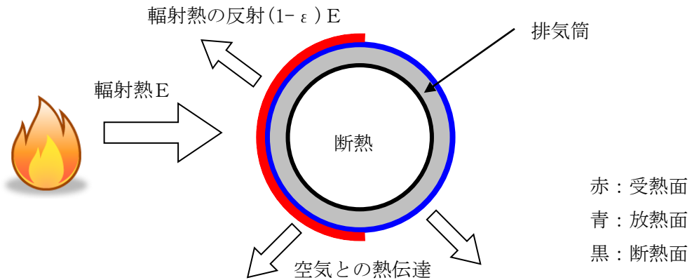
第2.2.2.3-9図 排気筒温度評価体系図
