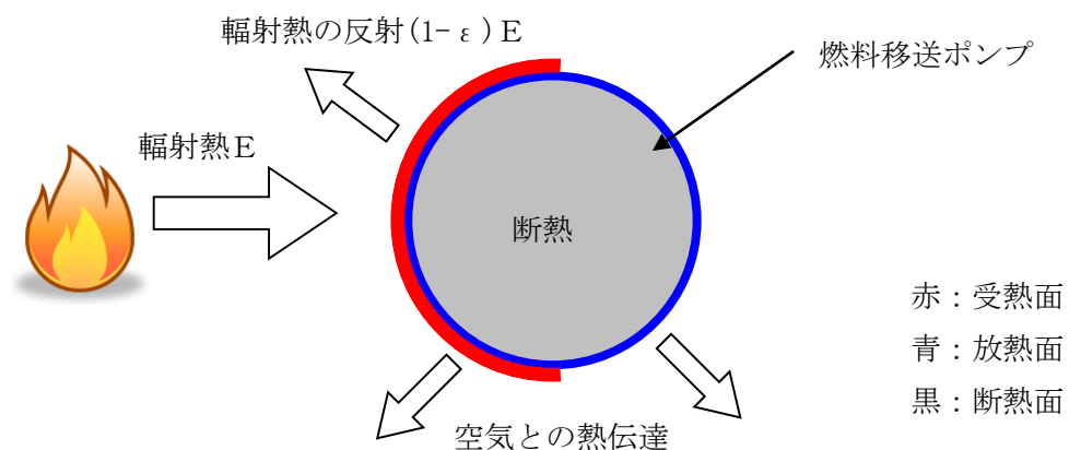
第2図 燃料移送ポンプ温度評価体系図
