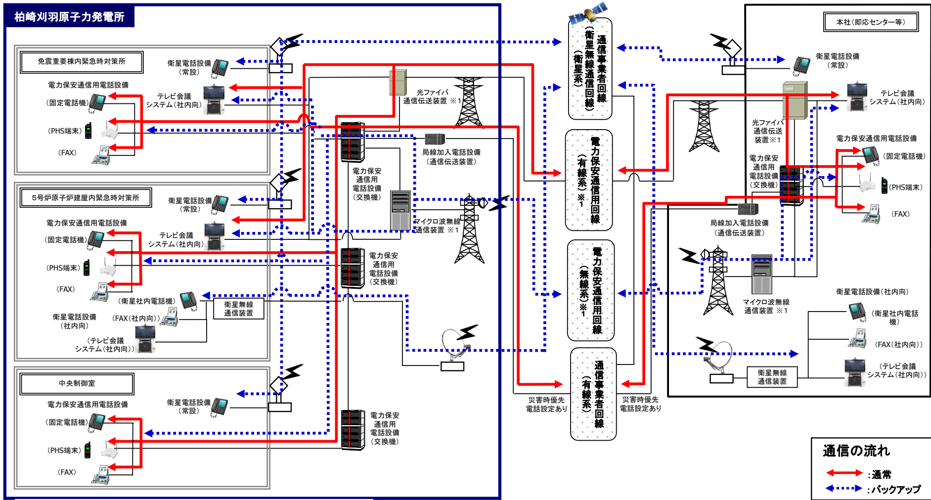
第 2.3-1 図 通信連絡設備 (発電所外 [社内関係箇所]) の概要 (電力保安通信用電話設備, 局線加入電話設備, 衛星電話設備, テレビ会議システム (社内向))
