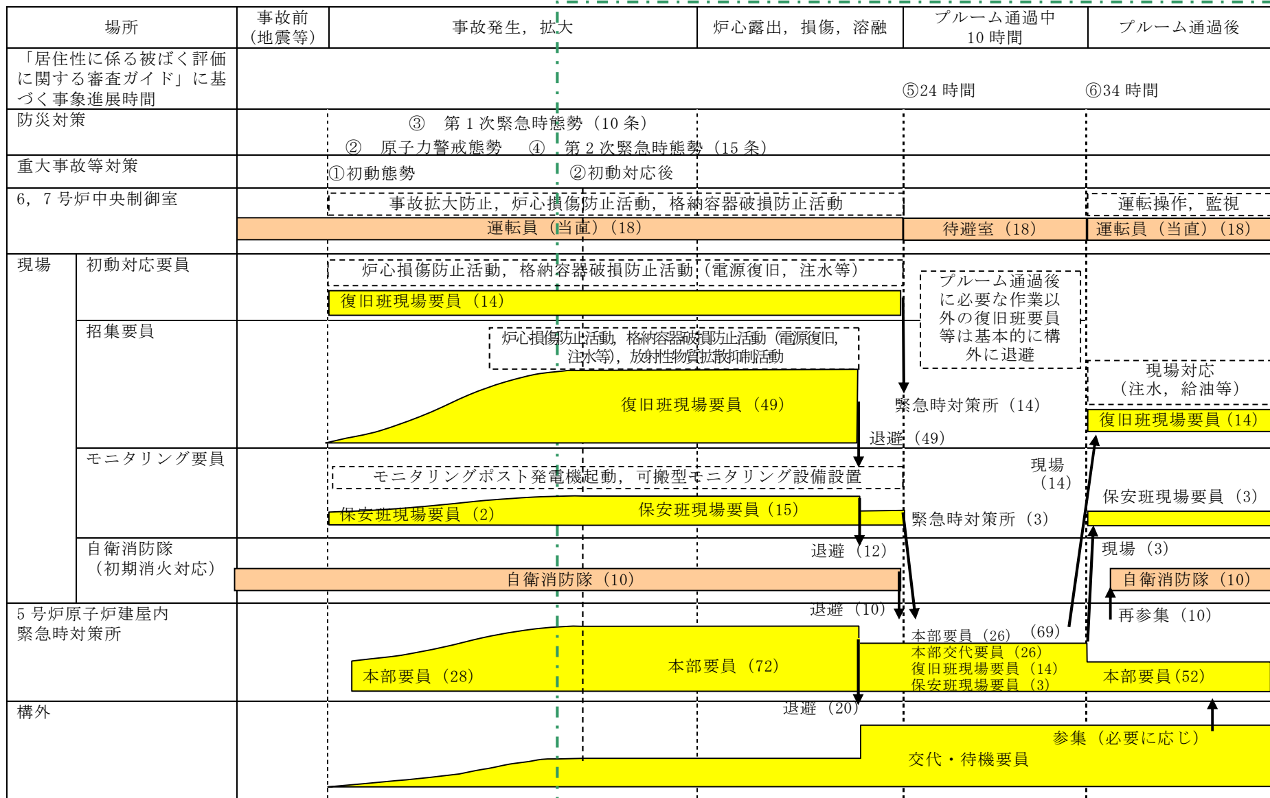
図 3.1-5 5 号炉原子炉建屋内緊急時対策所, 中央制御室 事故発生からブルーム通過までの要員の動き
