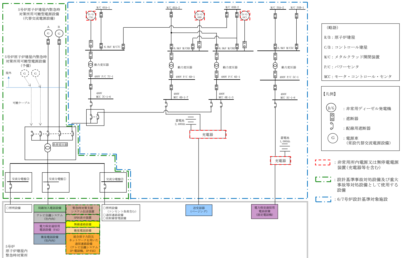
第2.6-4図 5号炉原子炉建屋内緊急時対策所における通信連絡設備の電源構成
