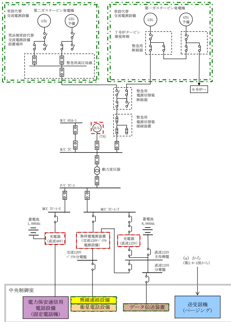
第2.6-2図 中央制御室における通信連絡設備の電源構成 (7号炉)
