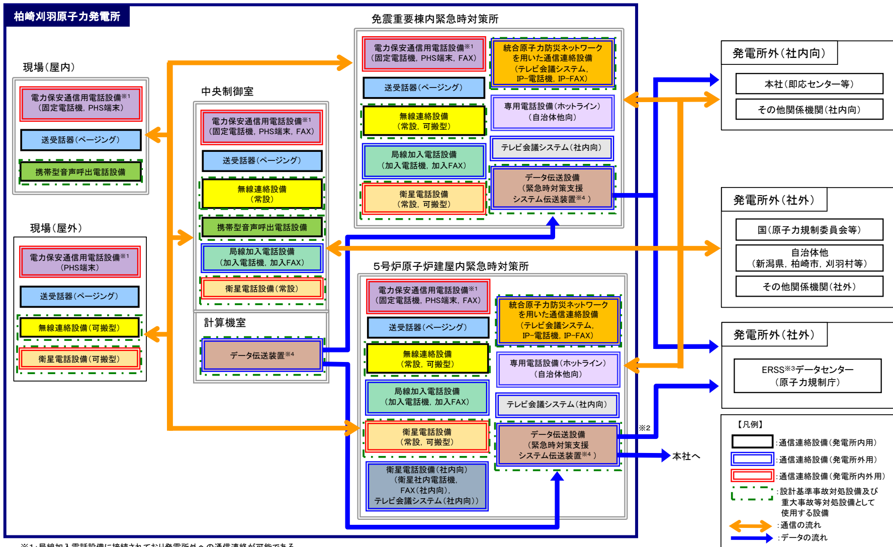
第 2-1 図 通信連絡設備の概要
