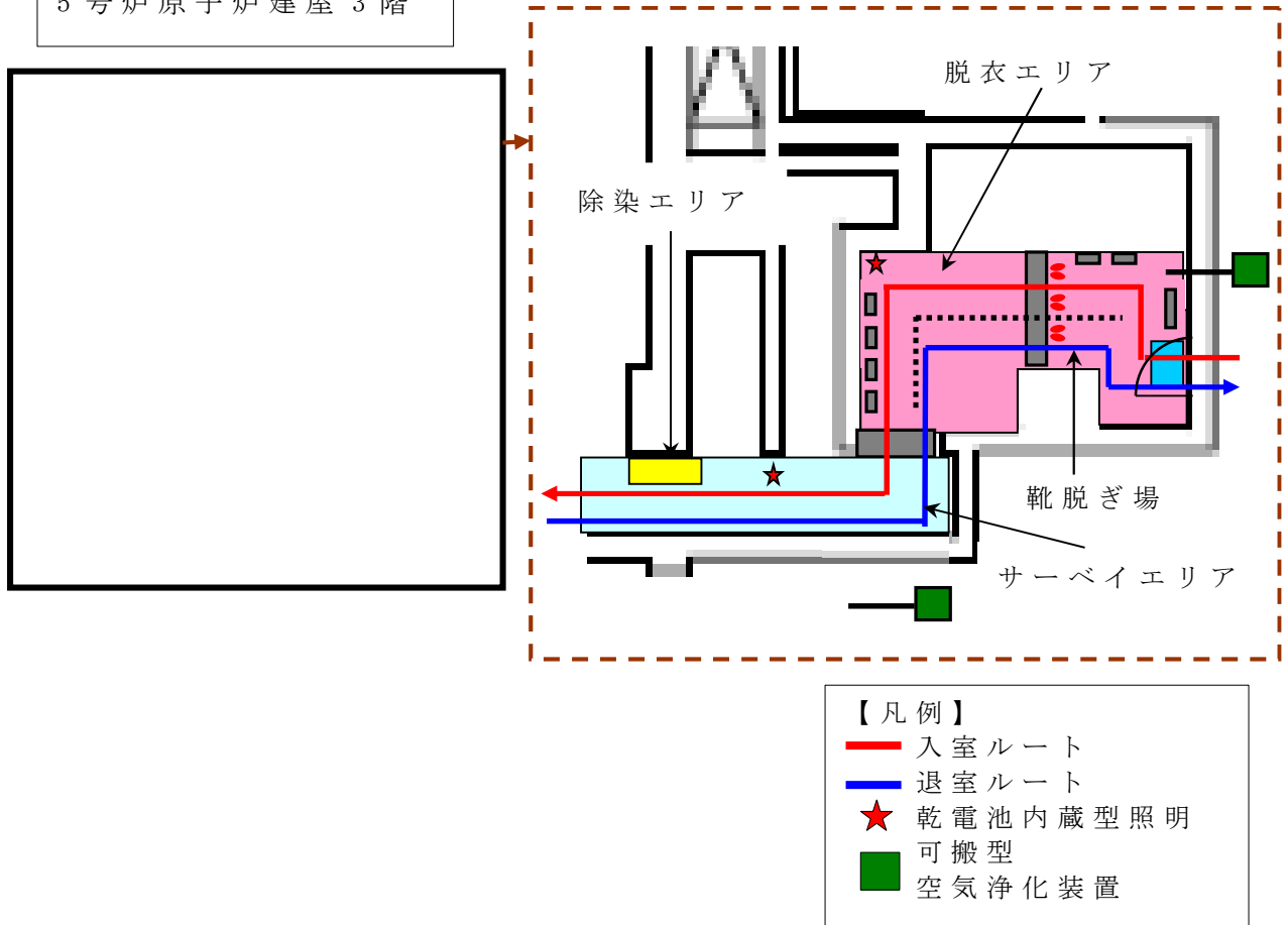
図 5.1-2 5号炉原子炉建屋内緊急時対策所チェンジングエリアの 設営場所及び屋内のアクセスルート
