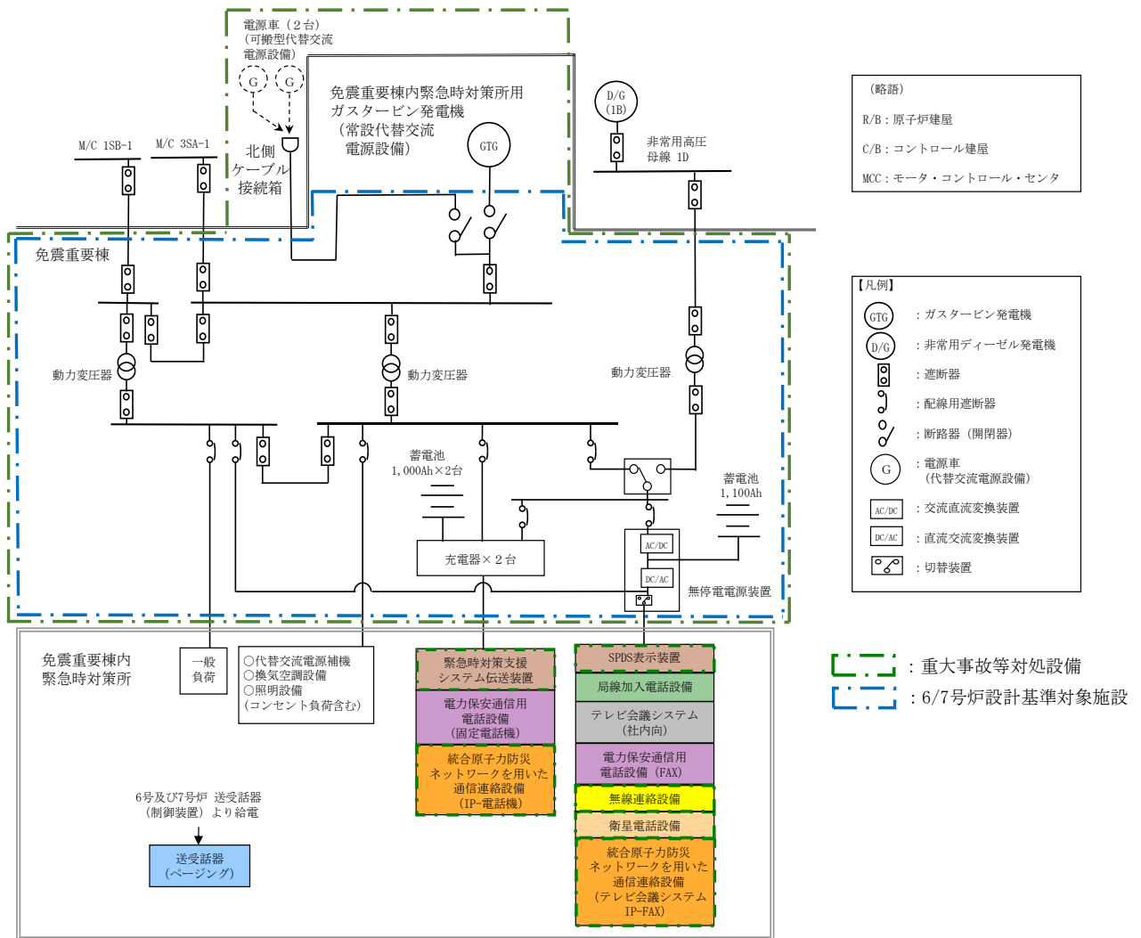
第 2.6-3 図 免震重要棟内緊急時対策所における通信連絡設備の電源構成
