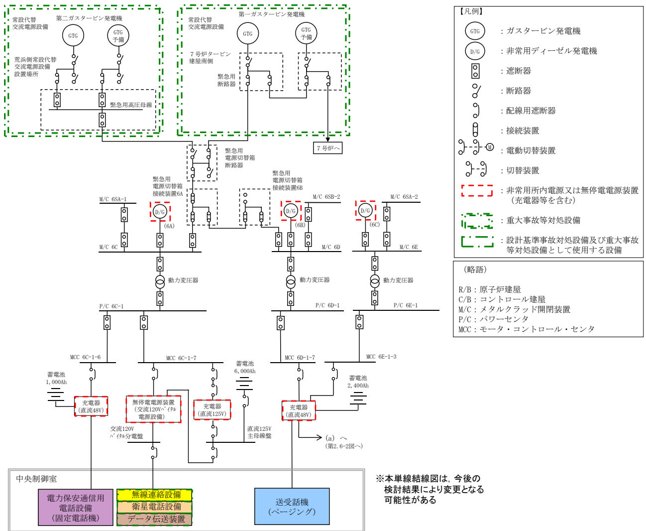
第2.6-1図 中央制御室における通信連絡設備の電源構成 (6号炉)
