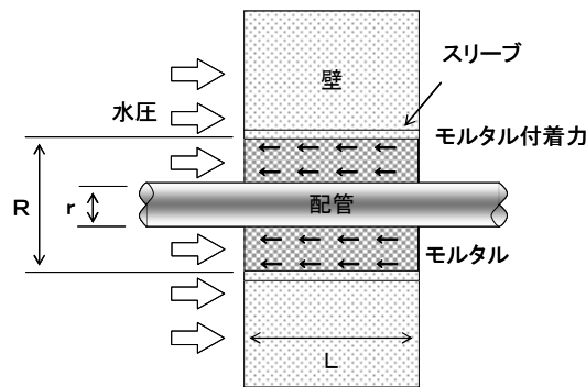
添付第 4.2.3-3 図 モルタル施工箇所概念図
