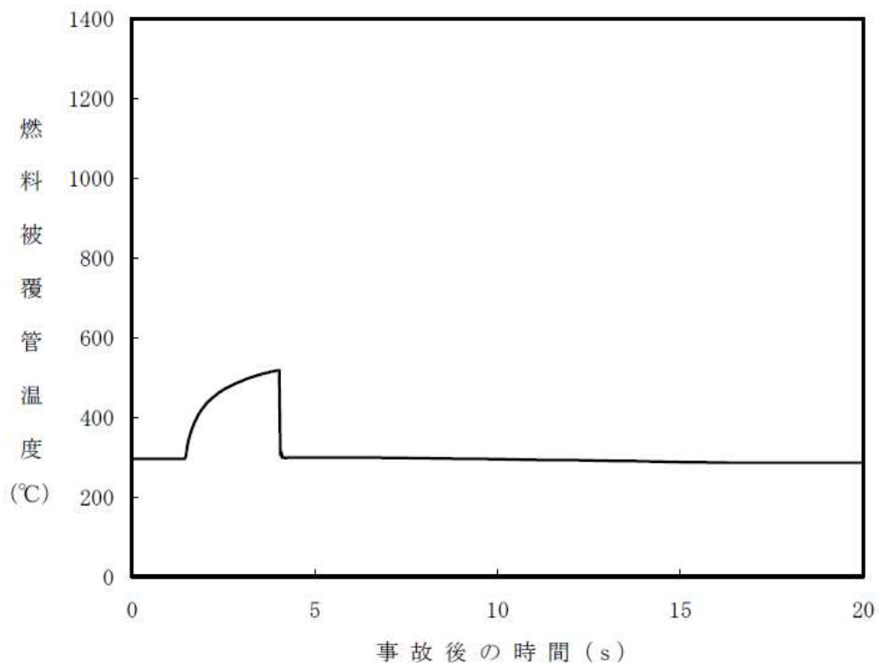
補足第 3.6.4.1-3 図 原子炉冷却材流量の喪失 + 給水制御系の故障解析結果 (原子炉建屋起因)
