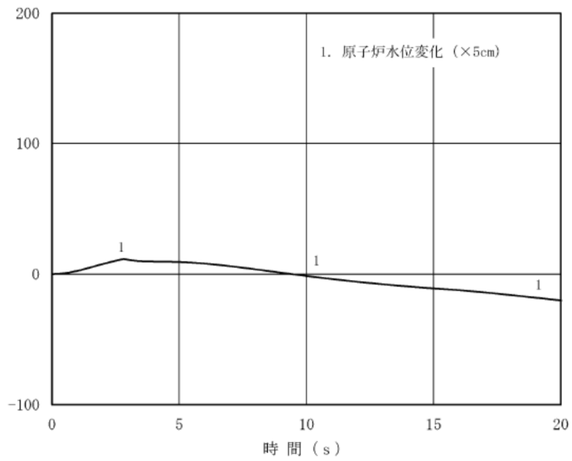
補足第 3.6.4. 1-3 図 原子炉冷却材流量の喪失 + 給水制御系の故障解析結果 (原子炉建屋起因)
