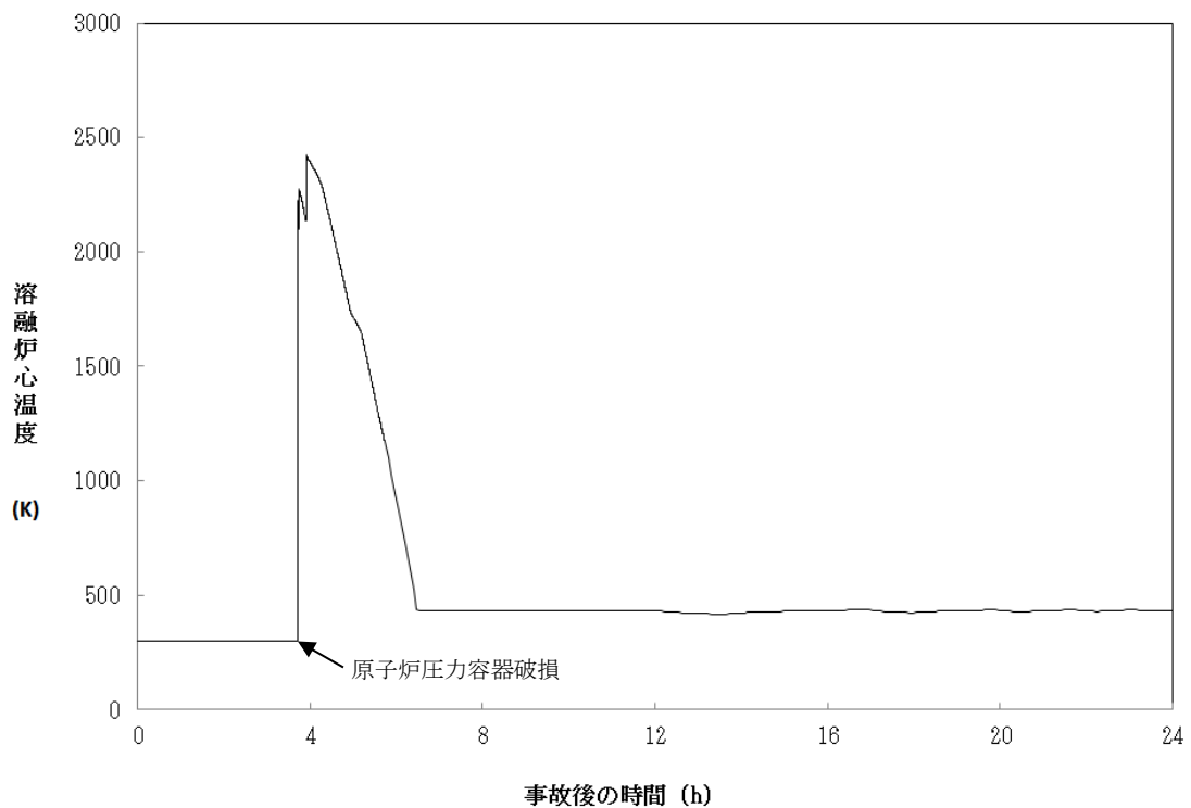
図 4-6b MCCI 評価時の溶融炉心温度
