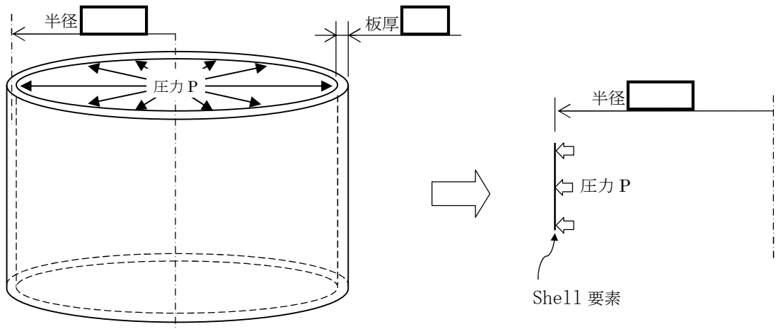
図 4-1 対象形状
