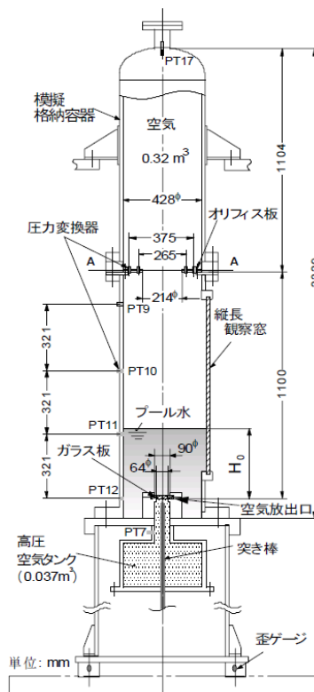
添付図 1 水撃実験装置（上：大型容器、下：小型容器）（稲坂ら，2004）
