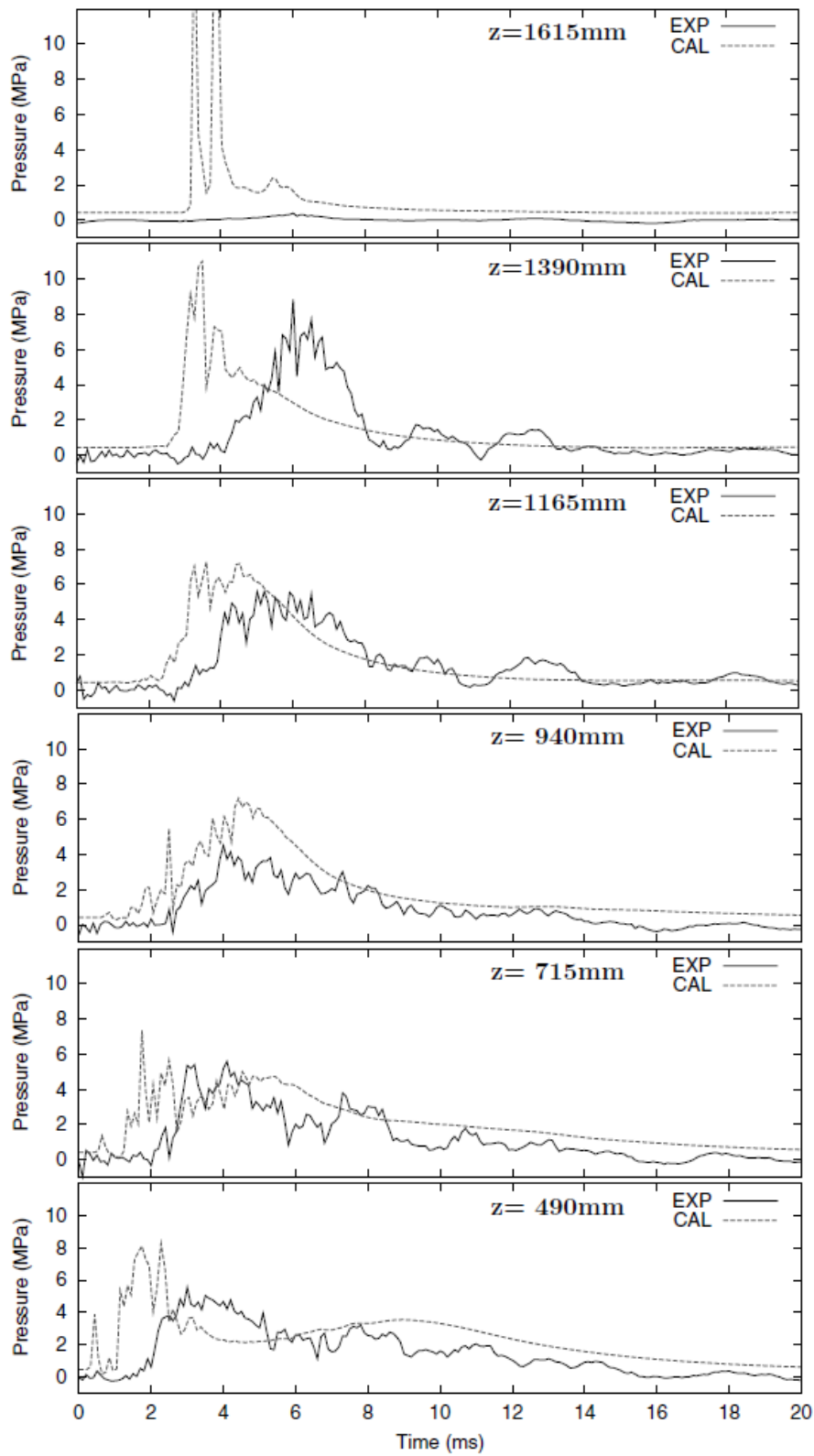
図 4.2.2.4 圧力履歴(FARO-L33)
