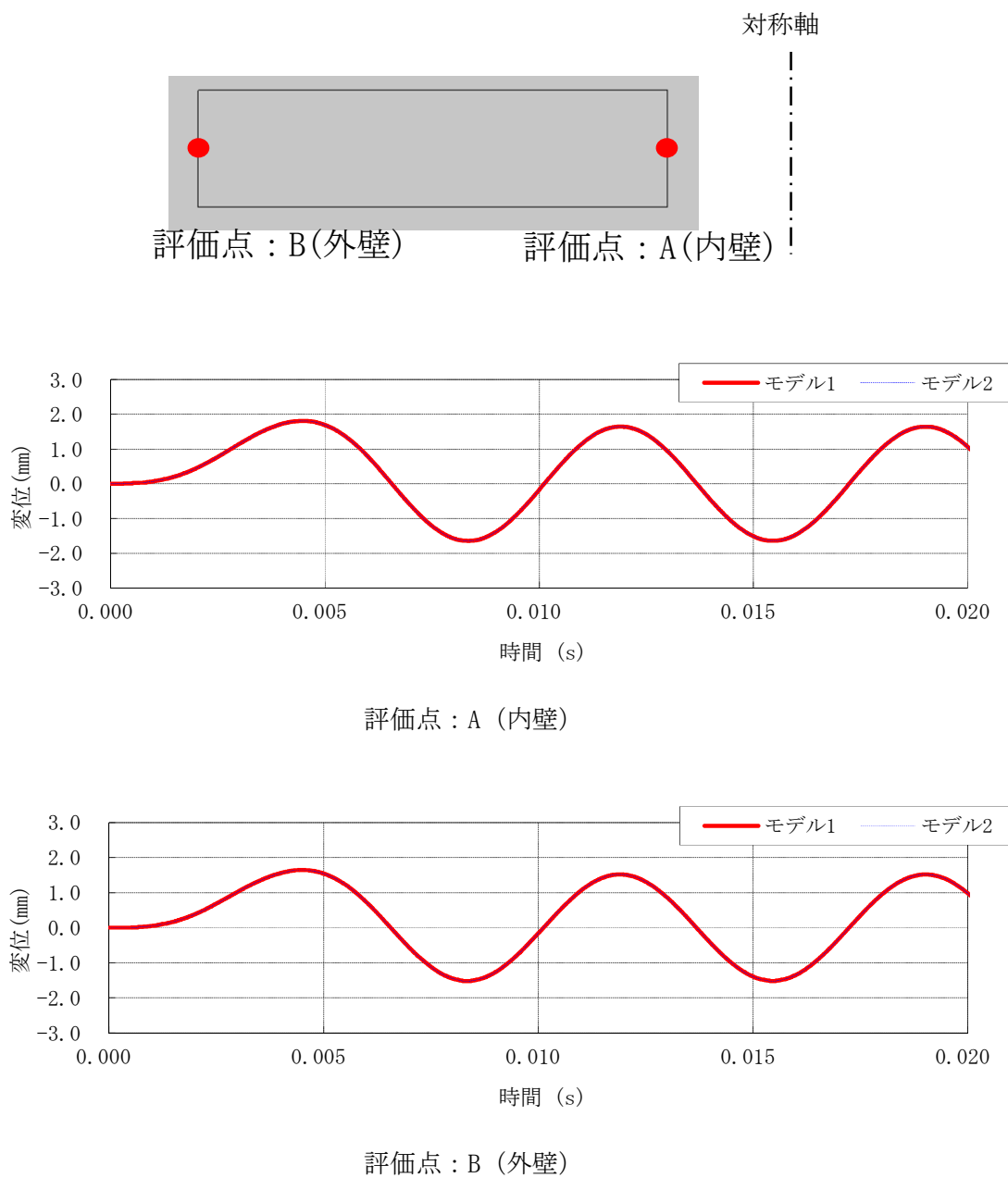
図 4-8 要素サイズの異なるモデルの動的解析結果の比較（径方向変位）
