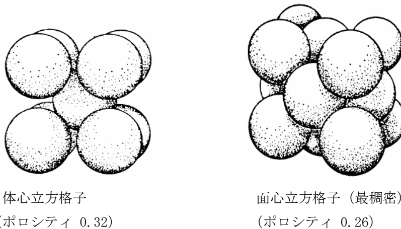
図 4-5 粒子の格子配列とポロシティ
