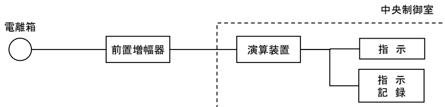
第1-5図 フィルタ装置出口放射線モニタの概略構成図
