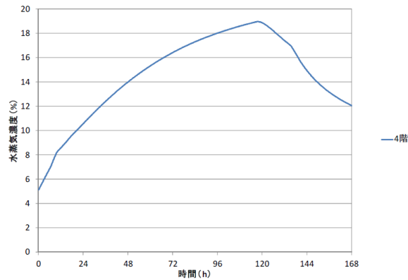
図 2-44 オペレーティングフロア水蒸気濃度 (10%/day 漏洩条件)
