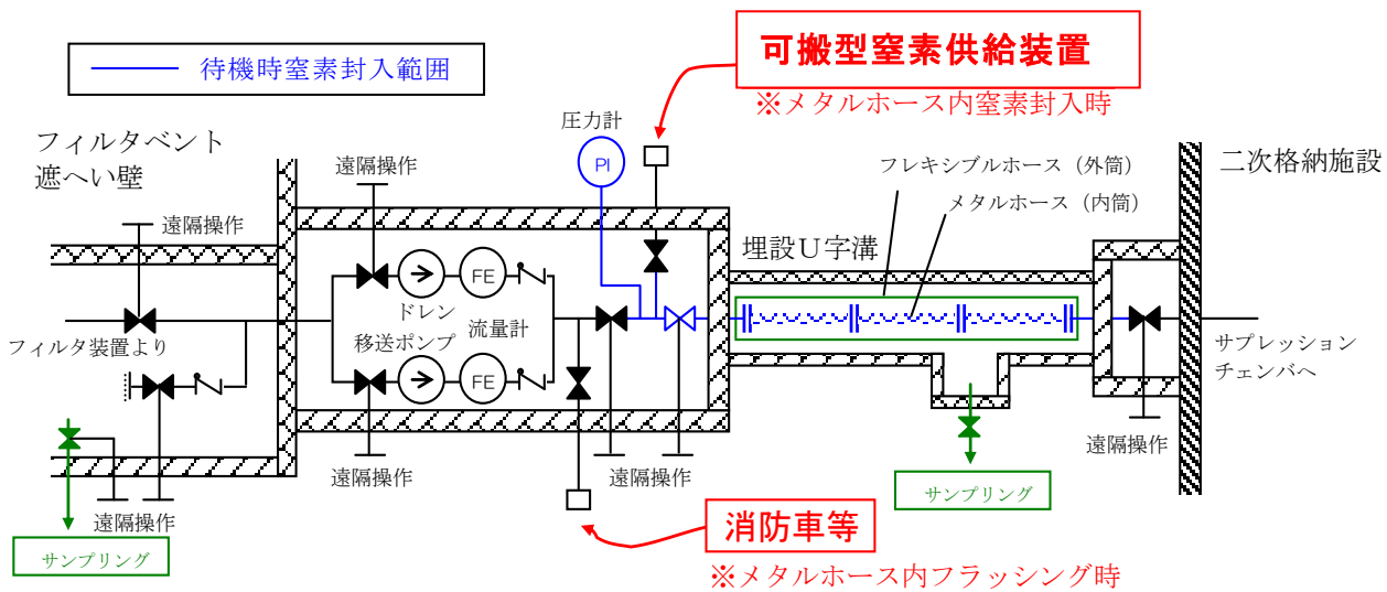
第 8 図 ドレン移送ライン概略系統図
