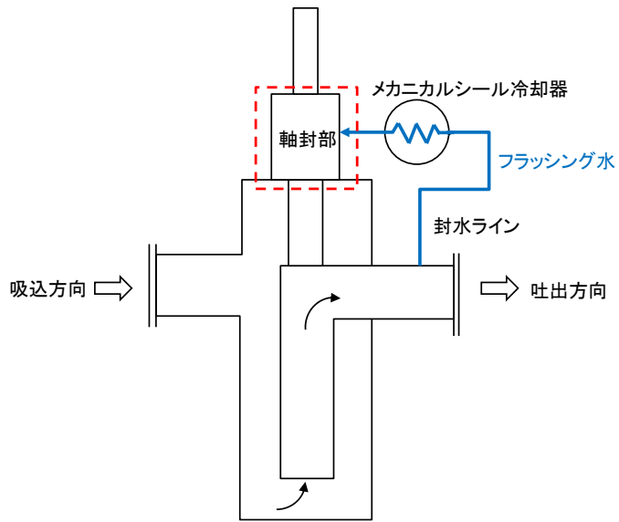
図 3.3-2 残留熱除去系ポンプ概要図
