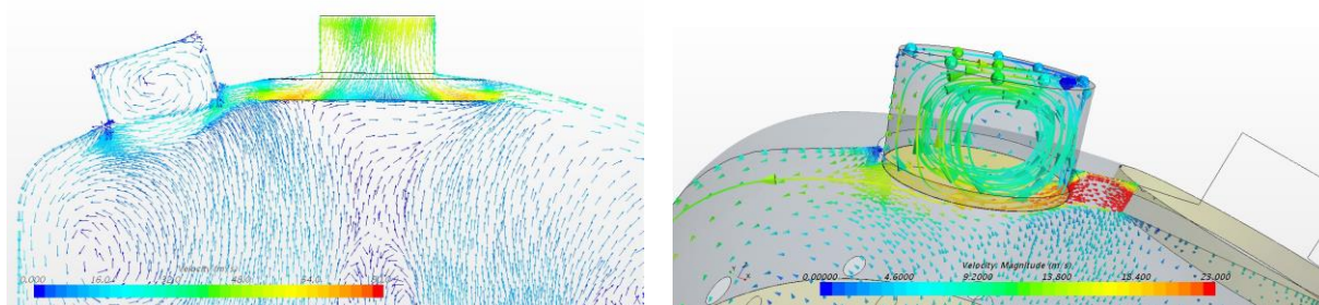
第1図 よう素フィルタ上部マンホール内ガス流れ状態 [ベントガス組成：水蒸気 100%， ガス流量：15.8kg/s]
