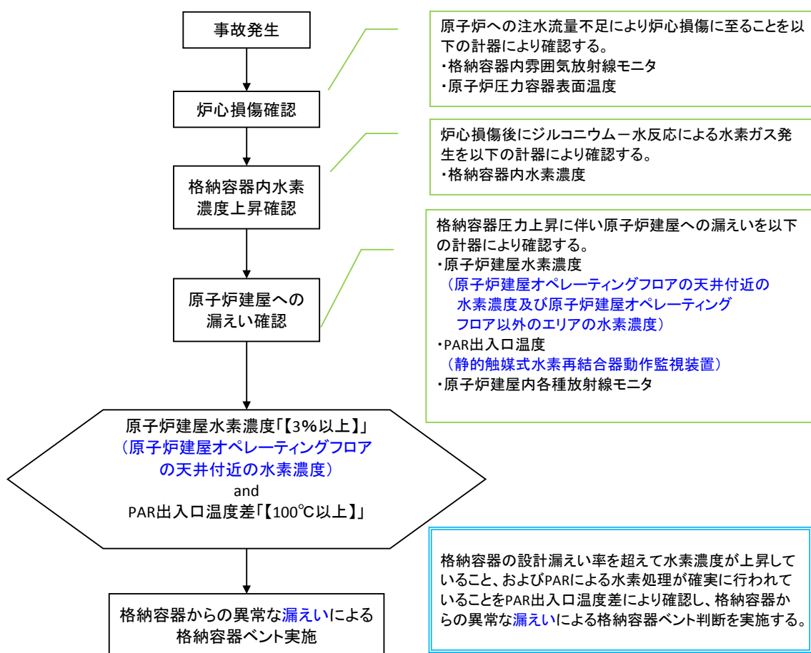
図 2-31 格納容器からの異常な漏洩による格納容器ベント操作概要
