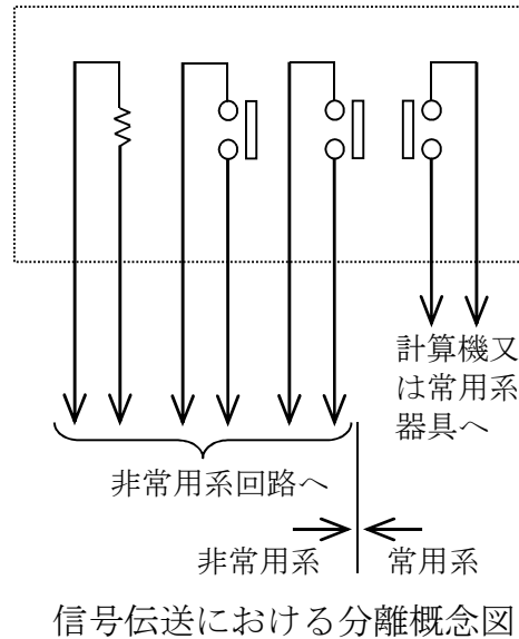
リレー回路を用いた隔離装置の代表例
