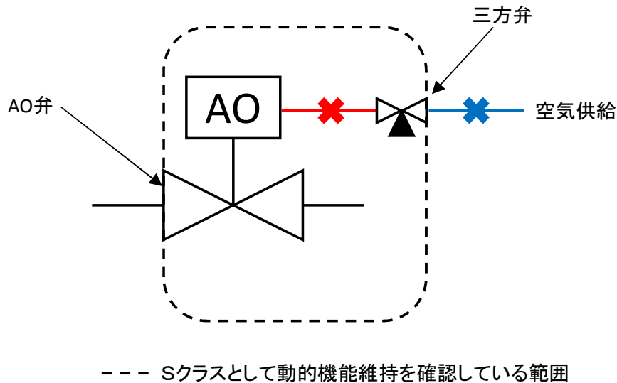
AO弁概念図
