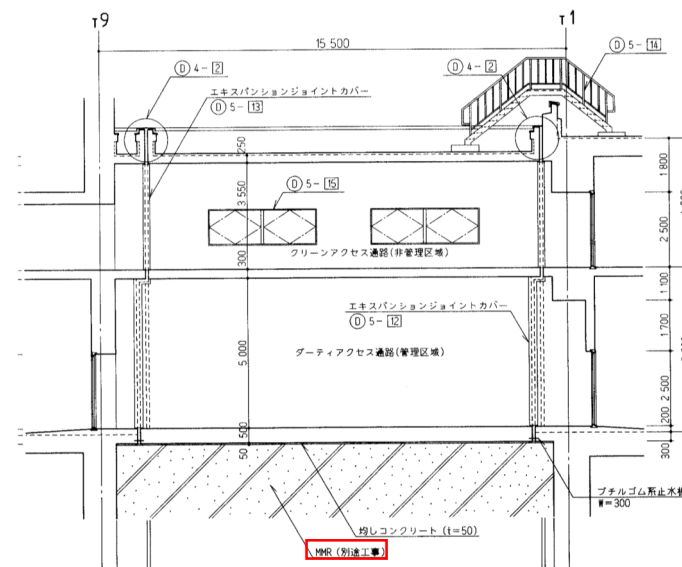
(b) B-B 断面図
