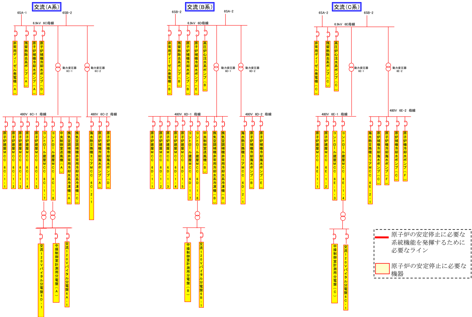
図 13 非常用電源系
