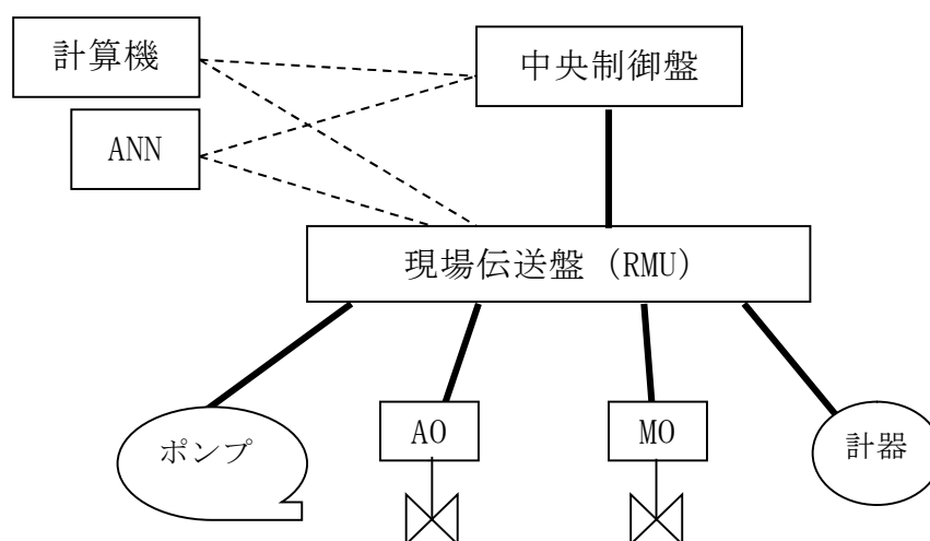
図 2-6：制御系ケーブル抽出対象範囲
