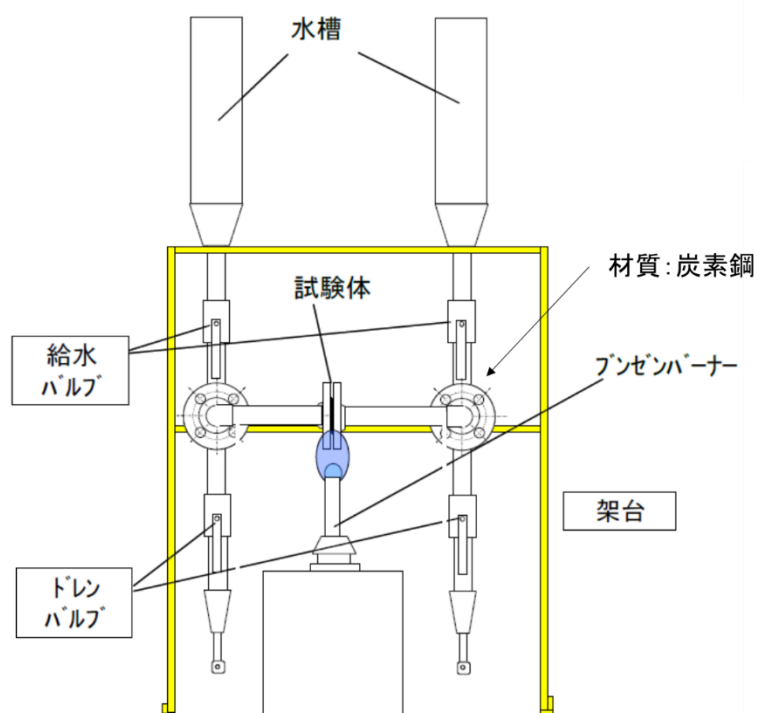
図1 加熱試験の概要
