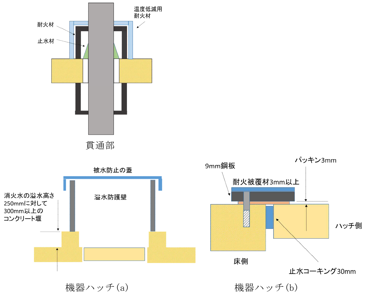
図 5-1 : タービン建屋 [redacted] (1)
