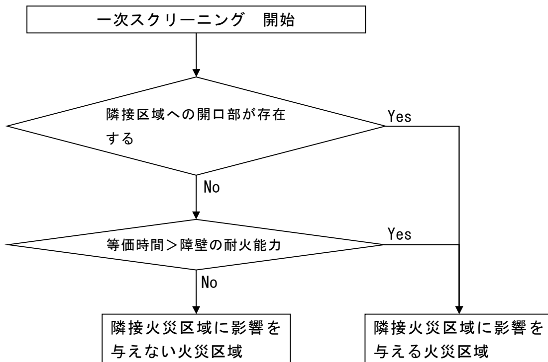
図 10-2 一次スクリーニングの概要フロー
