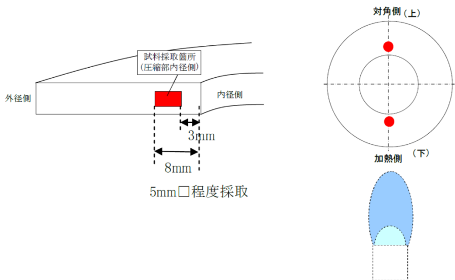
図3 熱重量測定 of 測定箇所
