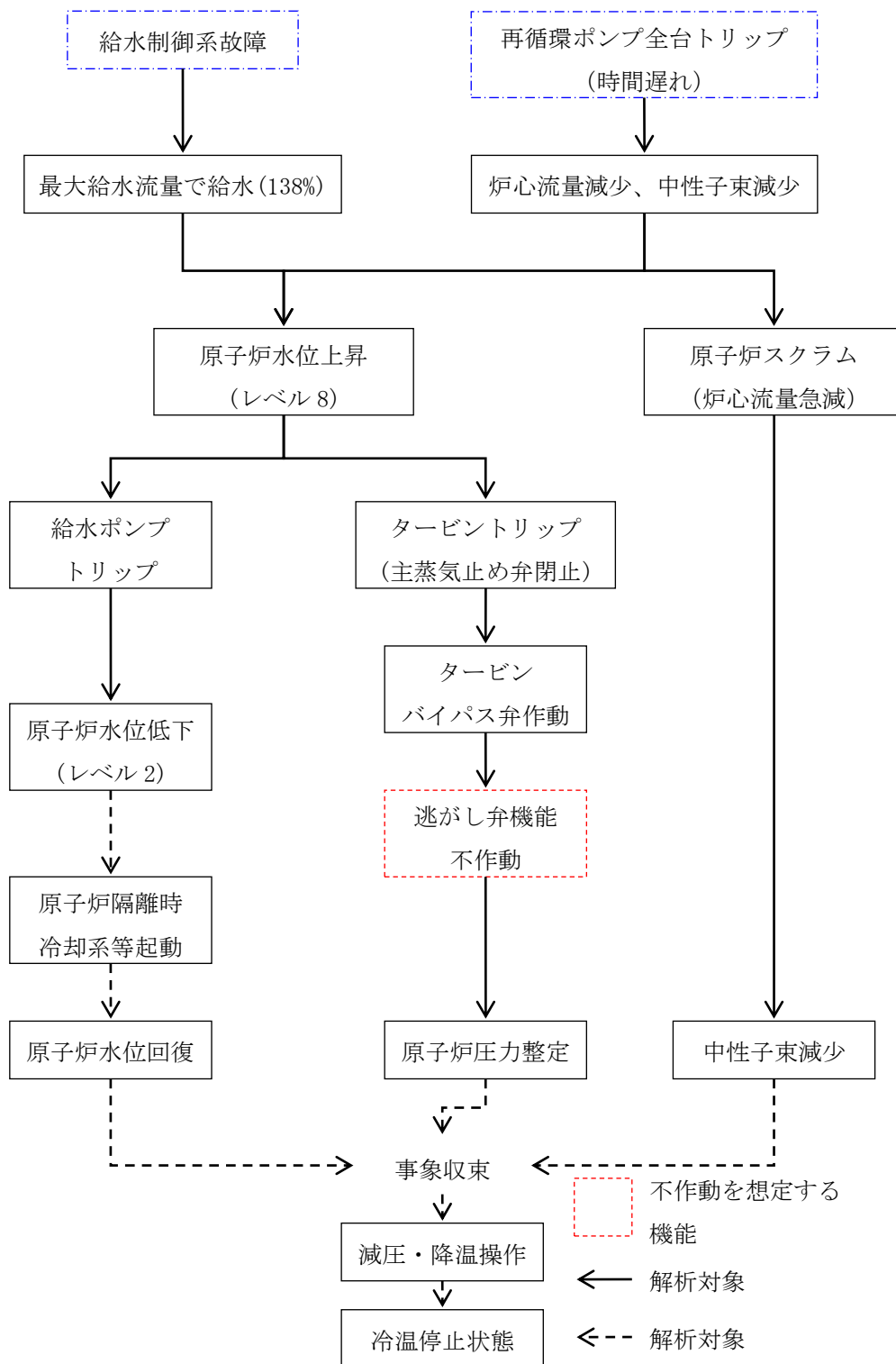
図 6-4 原子炉冷却材流量の喪失+給水制御系の故障事象進展フロー (R/B 起因)
