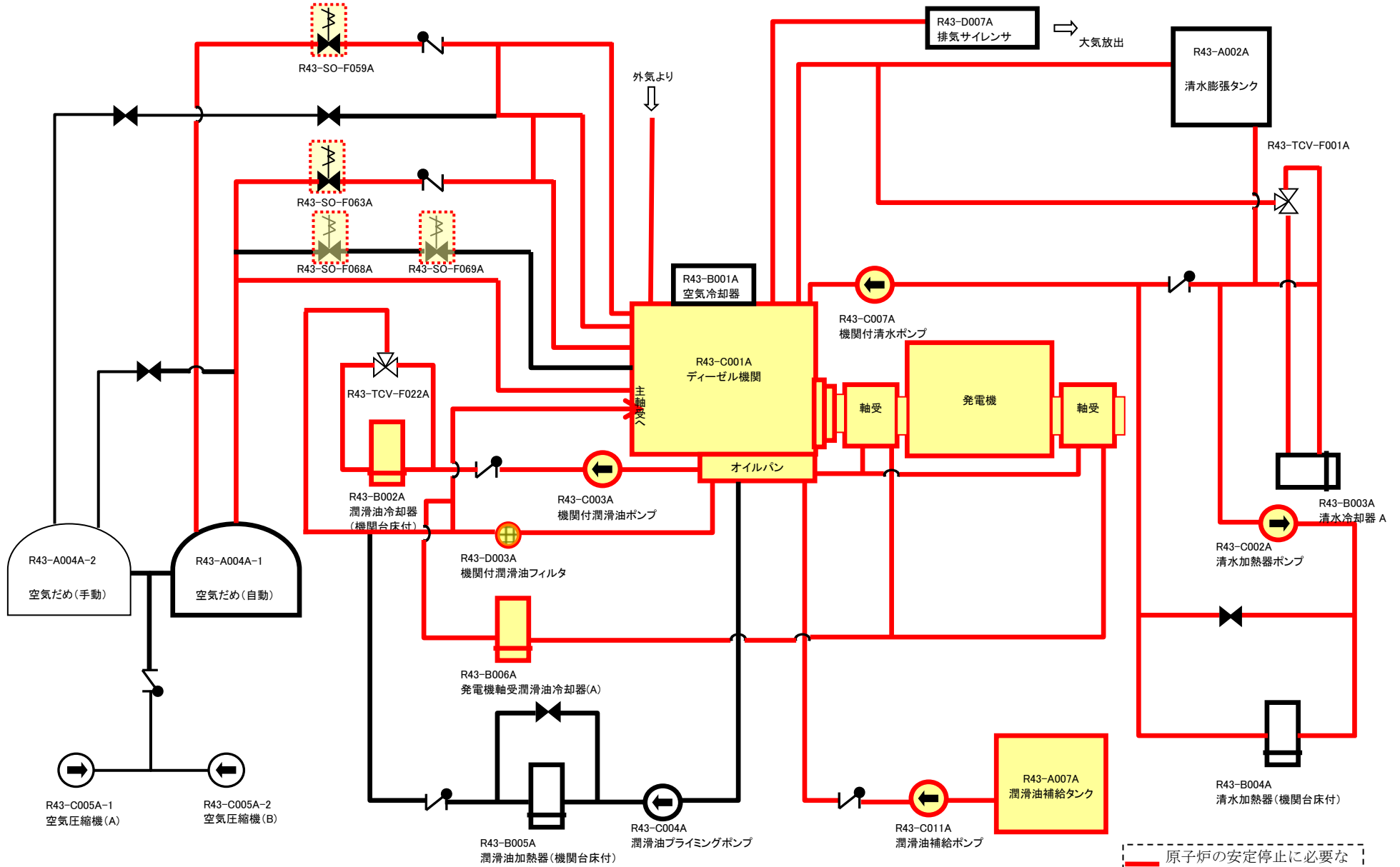
図 9 非常用ディーゼル発電機設備
