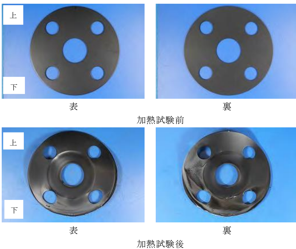
図6 加熱前後の試験体シート面（ゴム打ち抜きガスケット）
