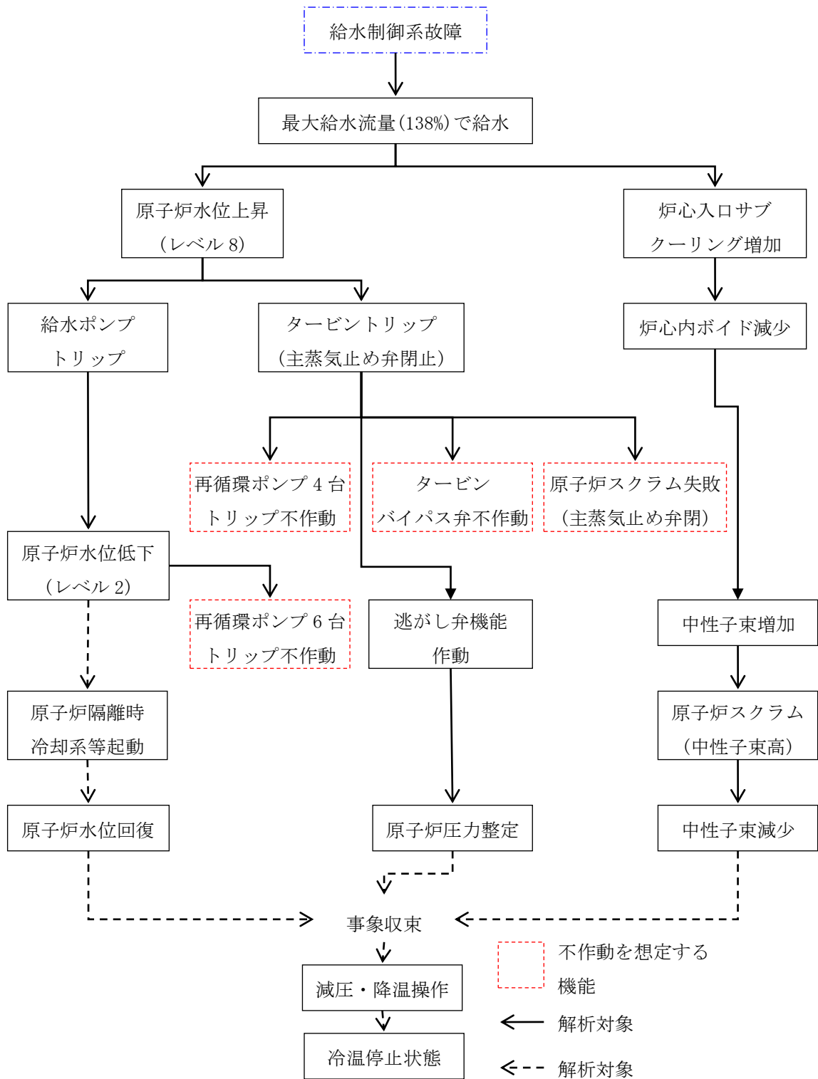
図 6-6 給水制御系の故障事象進展フロー (T/B 起因)
