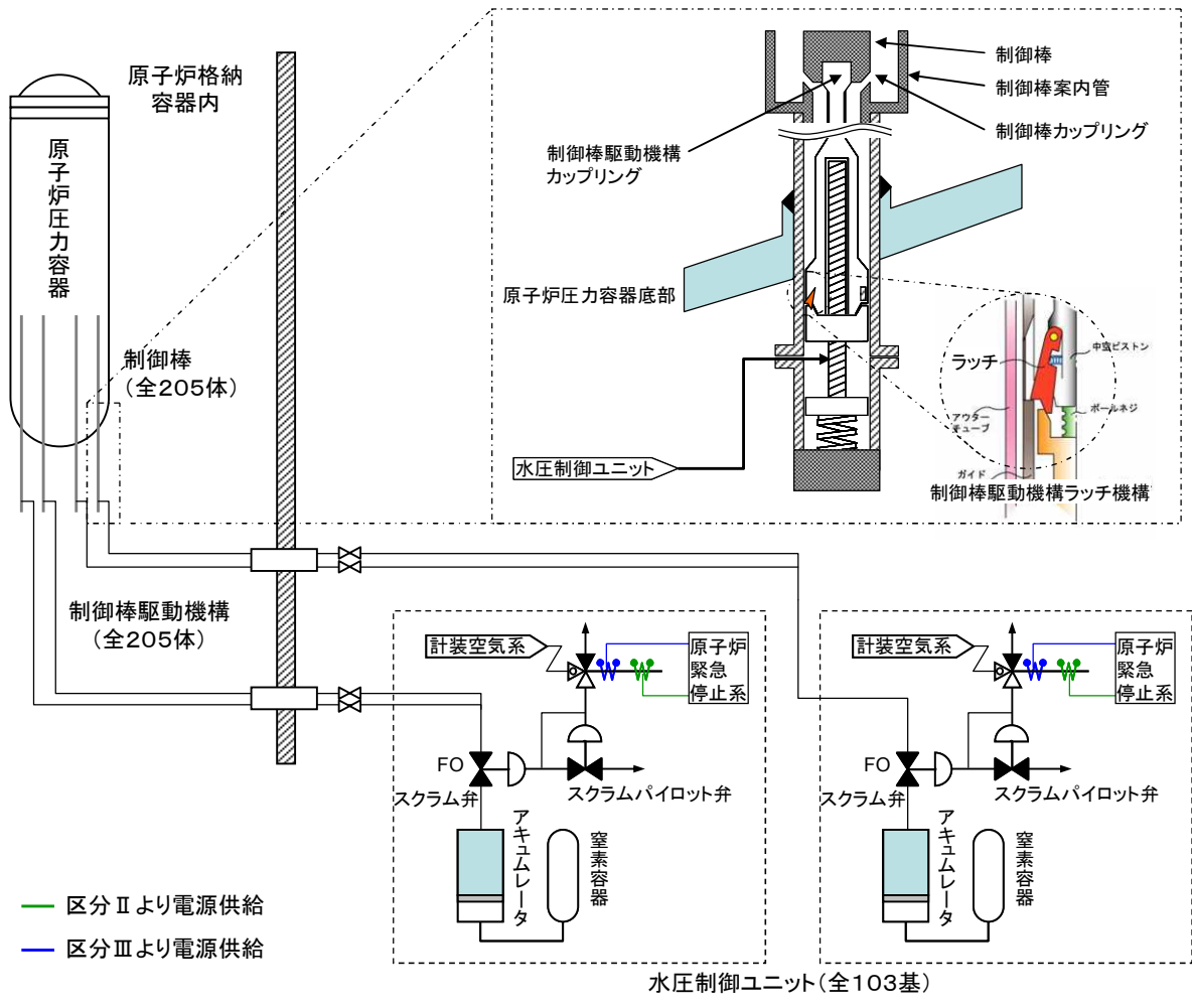
図 2-1：制御棒及び制御棒駆動系（水圧制御ユニット）の系統概略図
