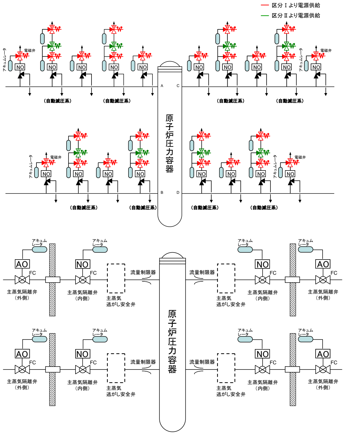
図 13 : 圧縮空気供給機能の概要
