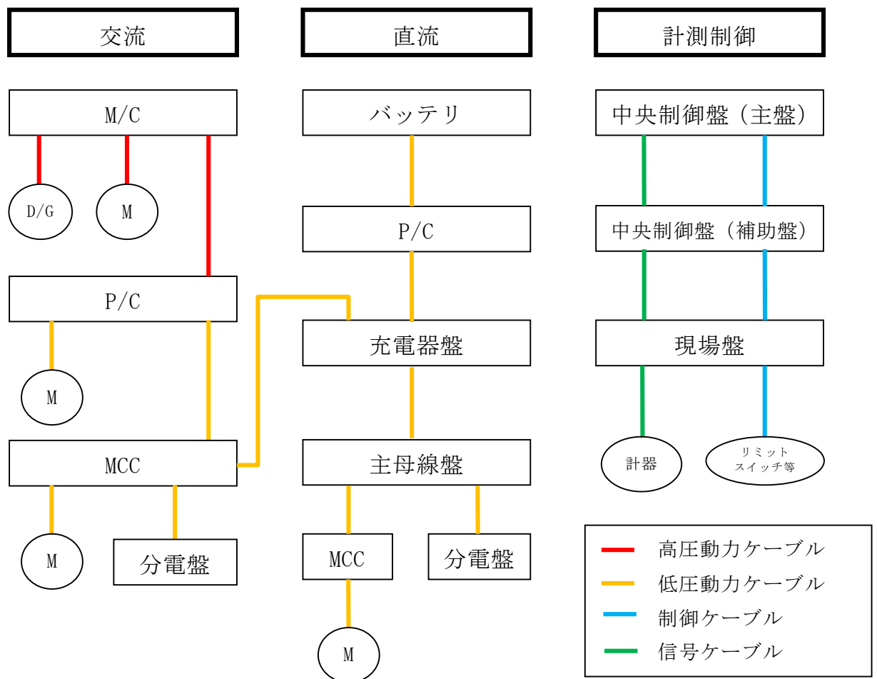
図 2-5：火災防護対策対象ケーブル調査範囲
