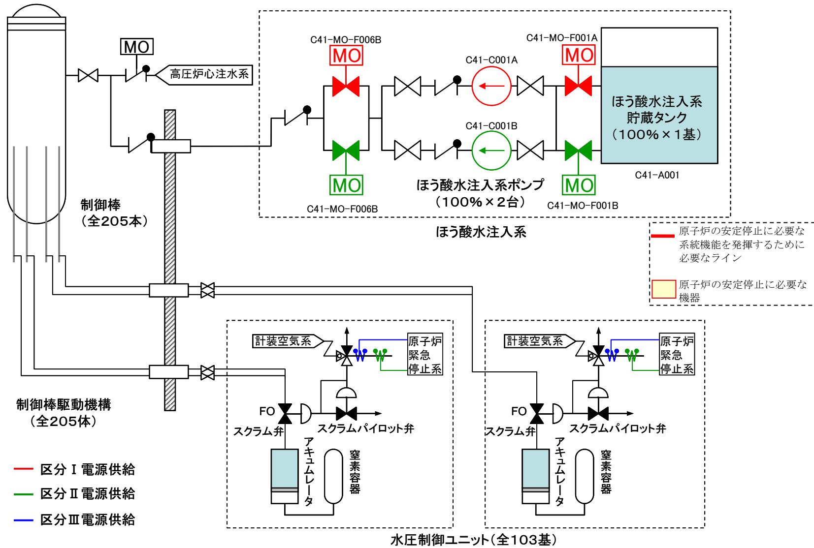
図2 ほう酸水注入系及び制御棒による系の概要
