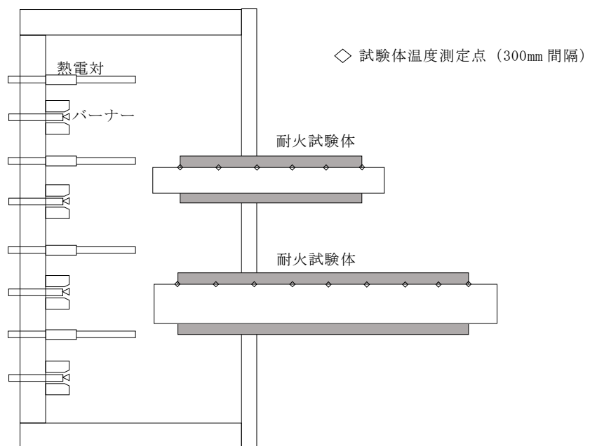
図 4-2 耐火試験炉
