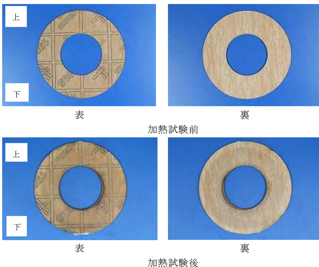
図4 加熱前後の試験体シート面（汎用非石綿ジョイントシート）
