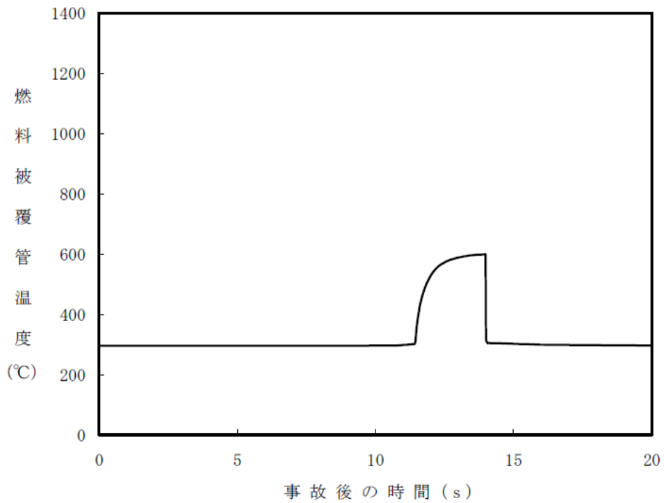
図 6-5 給水制御系の故障解析結果 (T/B 建屋起因) (2/2)
