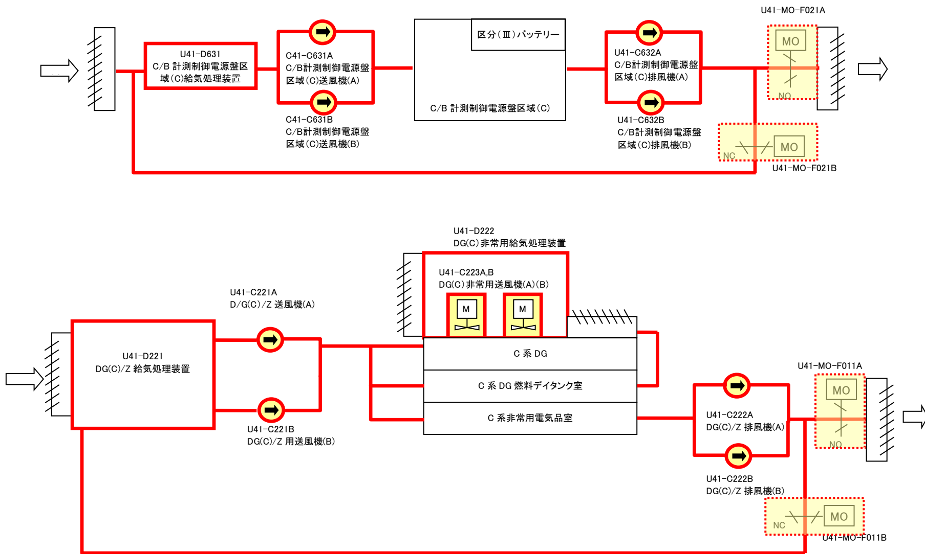
図 12 非常用換気空調系 (その 2)
