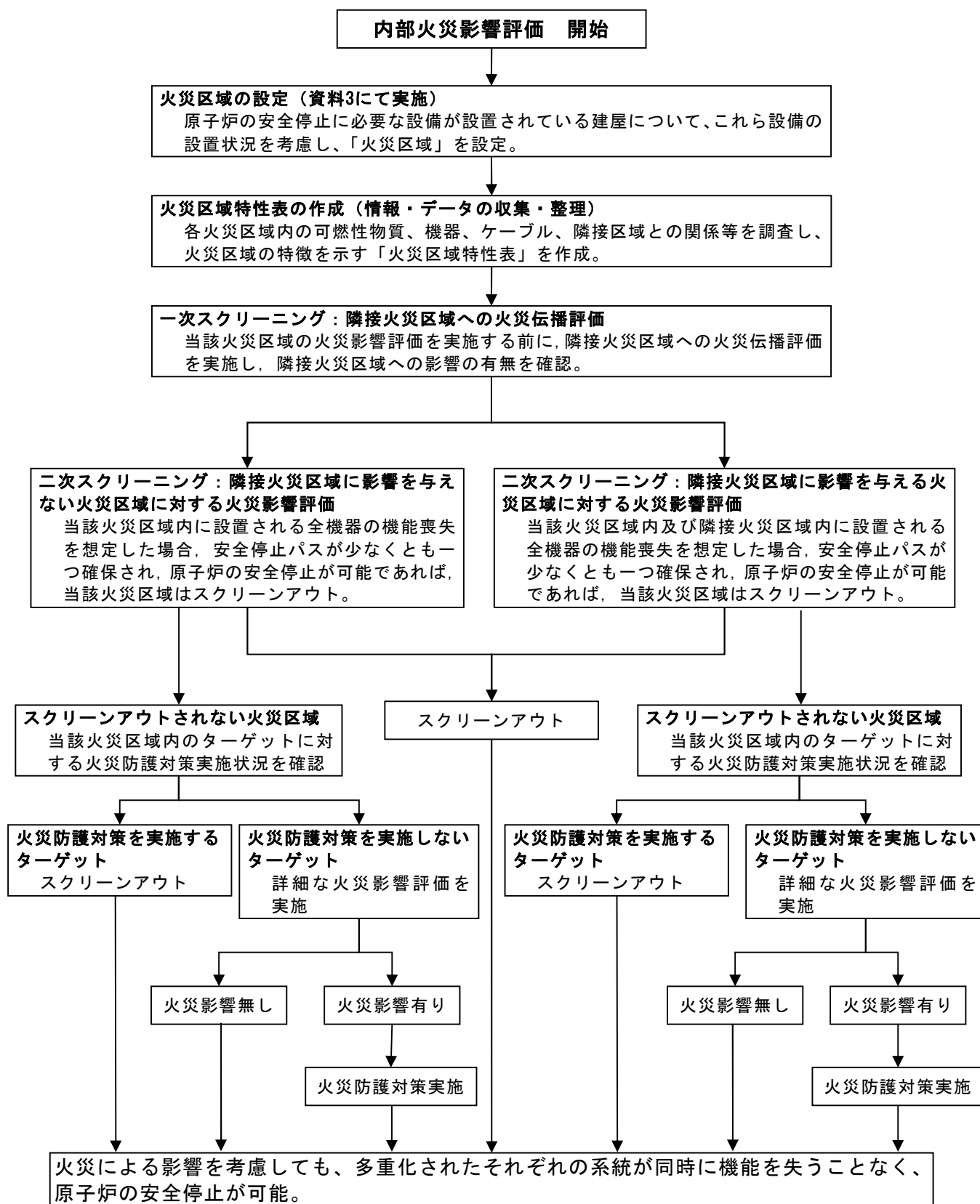
図10-1 火災影響評価の手順の概要フロー
