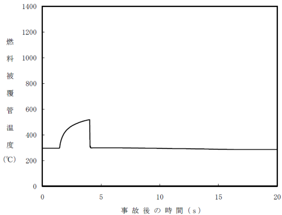
図 6-3 原子炉冷却材流量の喪失+給水制御系の故障解析結果 (R/B 起因) (2/2)
