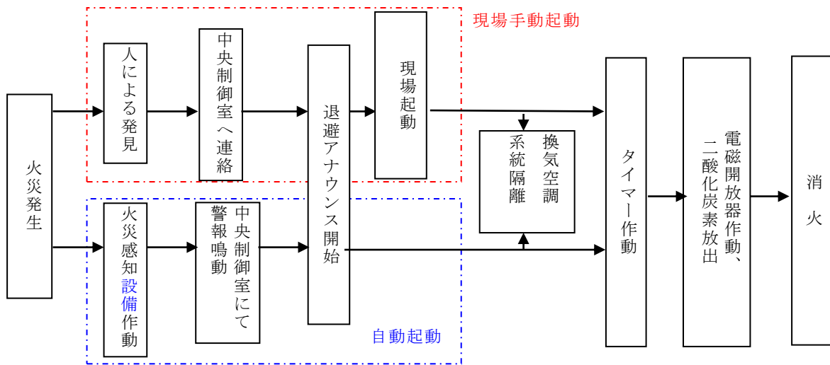
図2 火災時の信号の流れ
