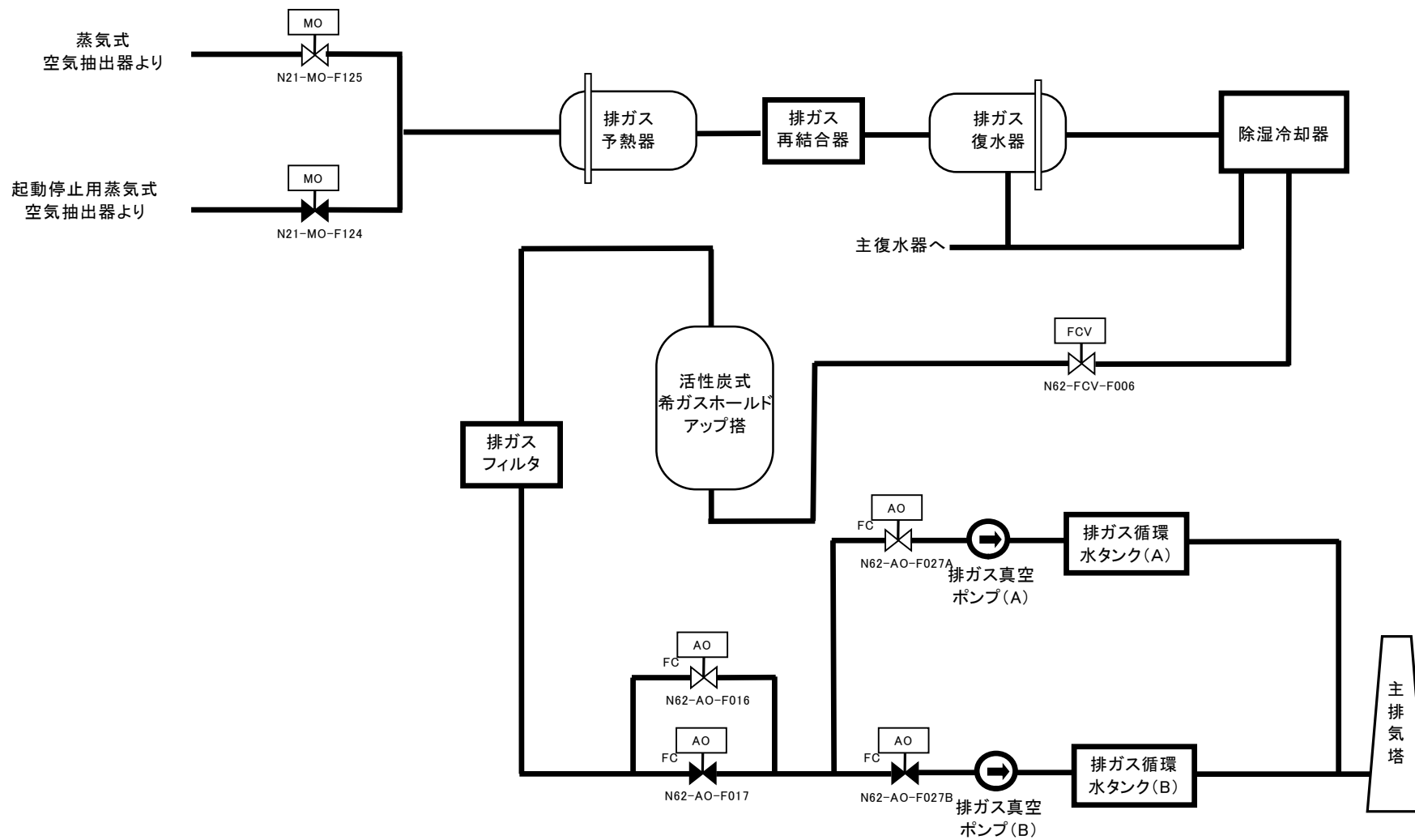
図 9-3 : 気体廃棄物処理系 系統概略図 (7号炉)
