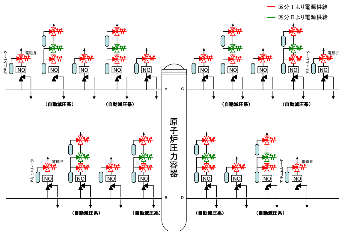
図 4：原子炉冷却材圧力バウンダリの過圧防止機能の概要
