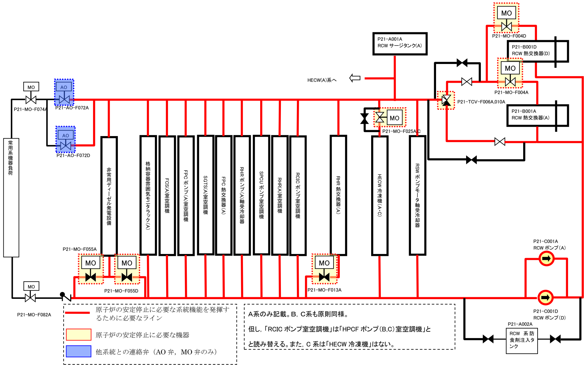
図 6 原子炉補機冷却系
