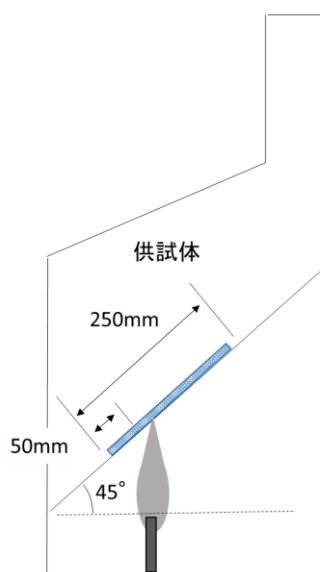
図 2 : JIS L 1091 試験概要図
