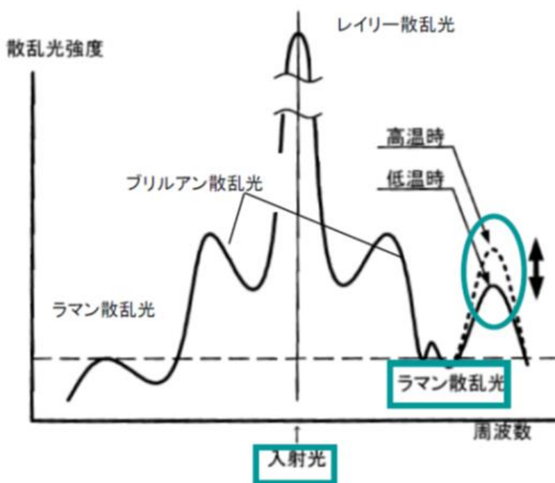
図1 温度測定の原理
