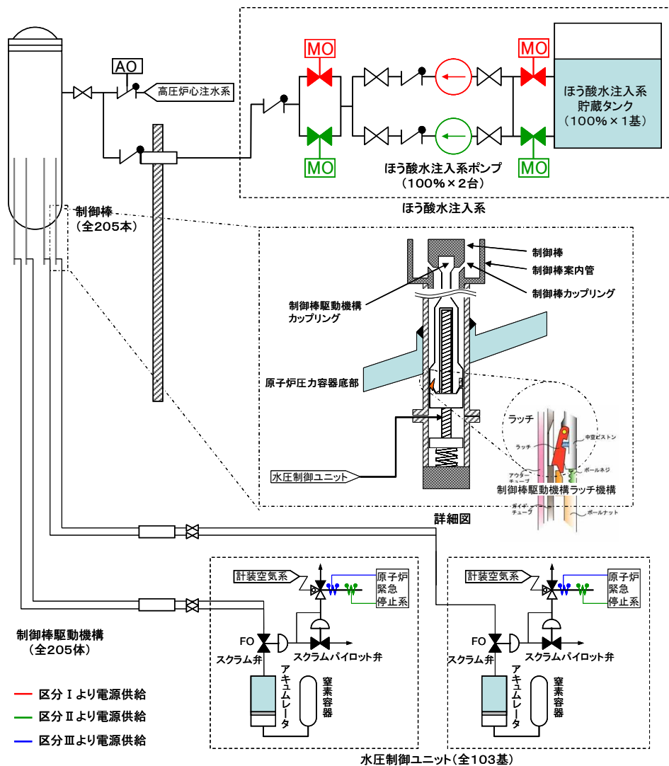
図 2-2 : ほう酸水注入系及び制御棒による系の系統概略図
