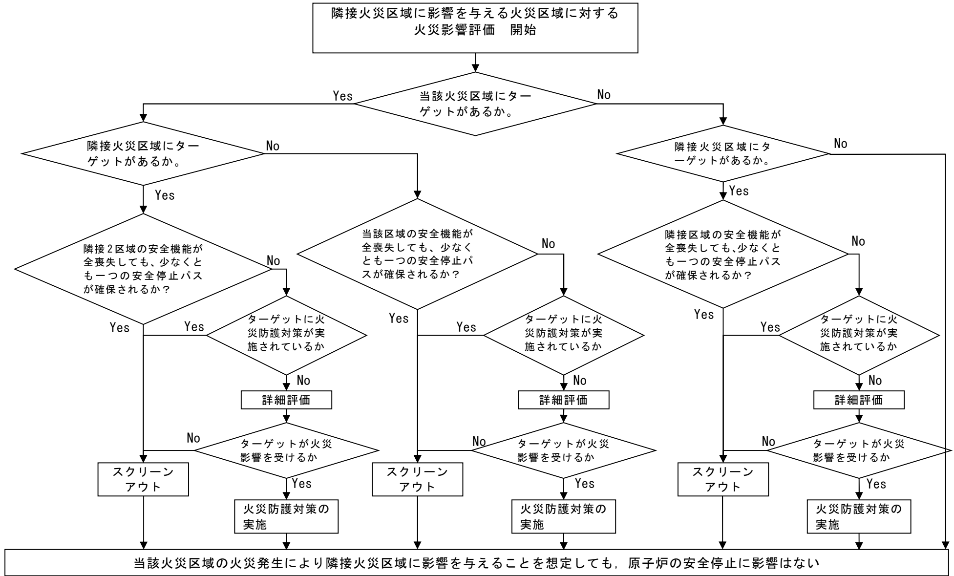
図 10-4 隣接火災区域に影響を与える火災区域に対する火災影響評価
