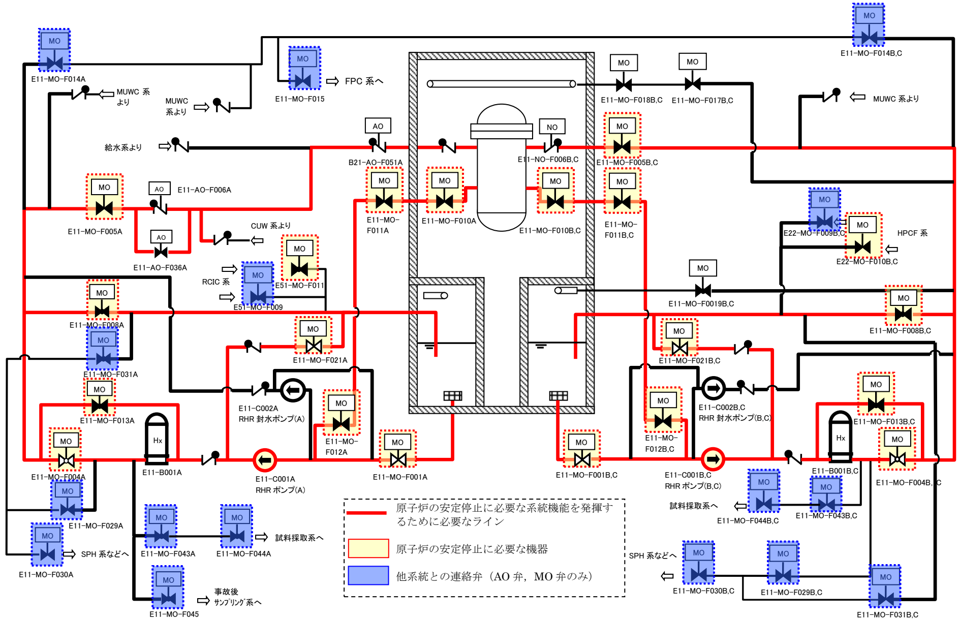
図 3 残留熱除去系
