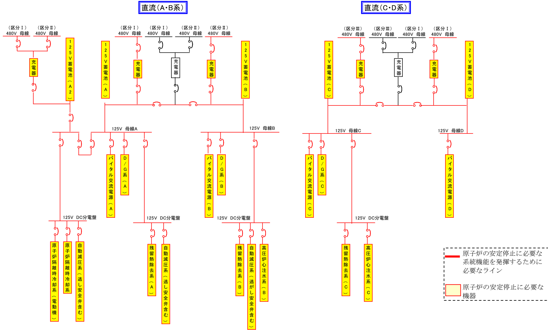
図 14 直流電源系
