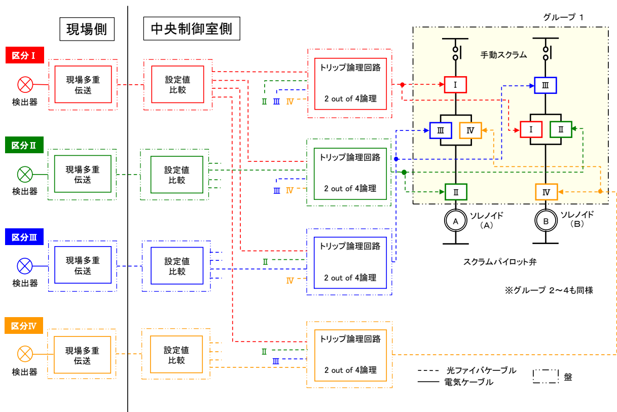
図1 光ファイバケーブルの使用箇所の概要 (原子炉緊急停止系の例)
