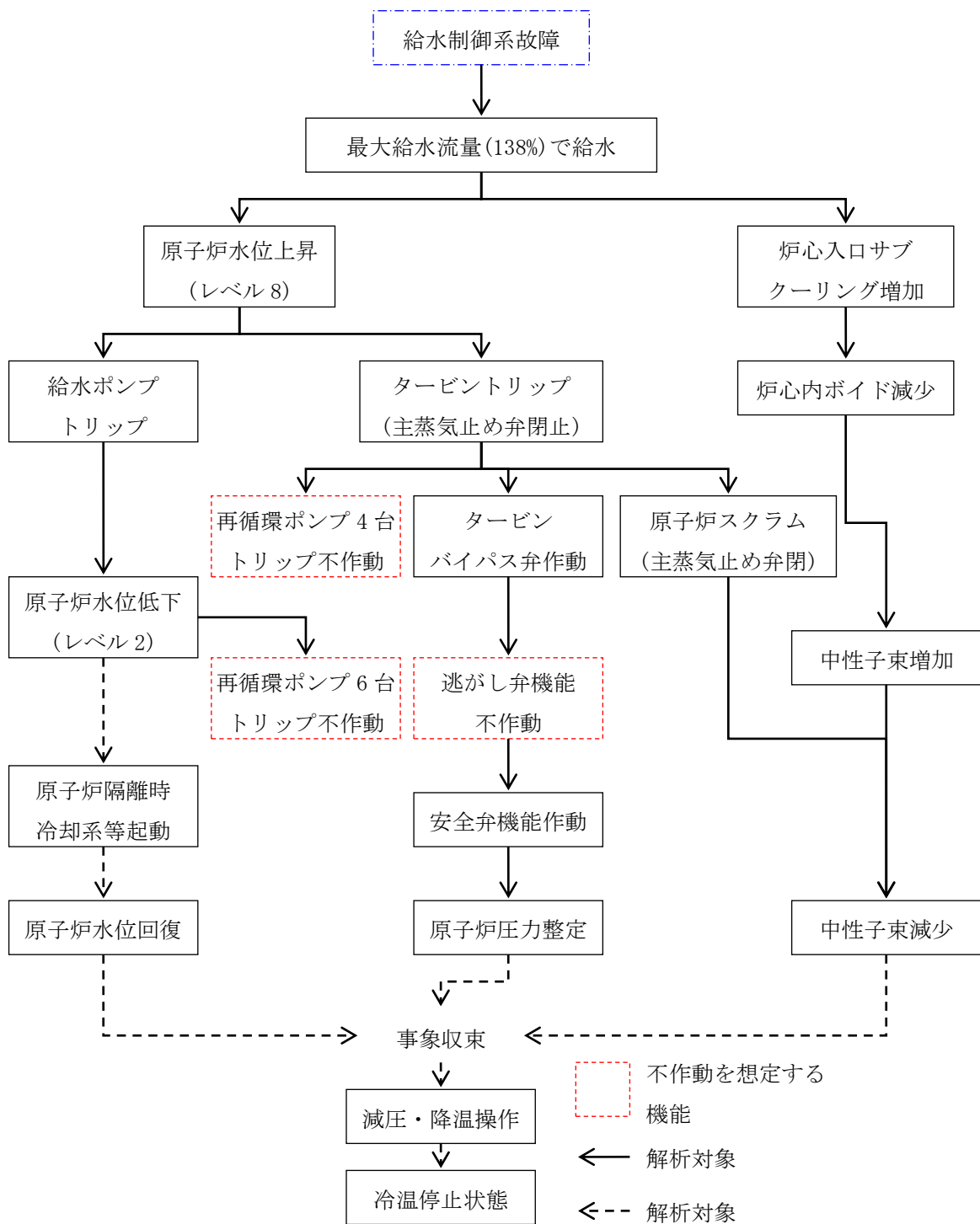
図 6-2 給水制御系故障事象進展フロー (R/B 起因)
