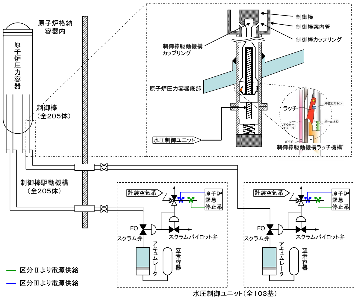
図1：原子炉の緊急停止機能の概要
