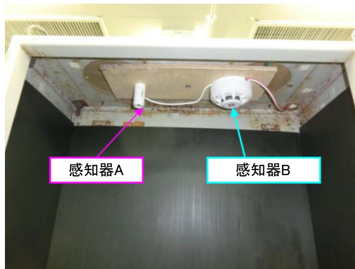
図1 模擬盤天井面への感知器設置状況
