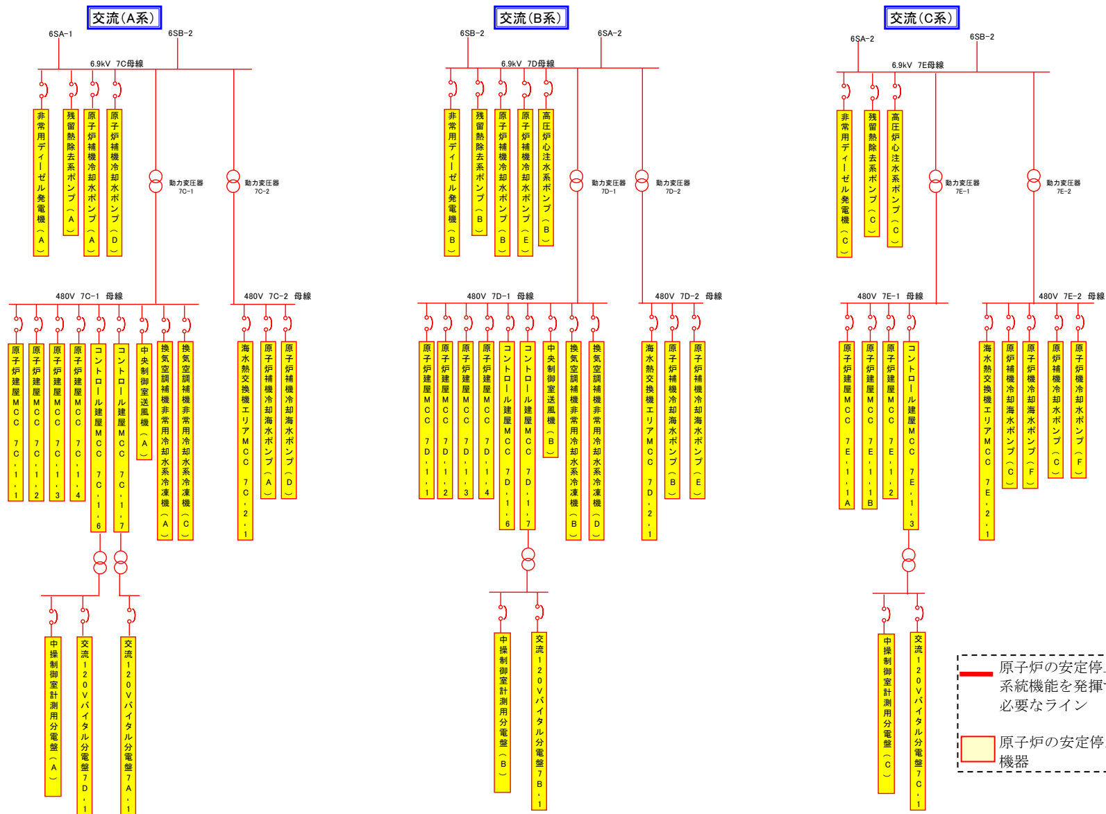
図 13 非常用電源系
