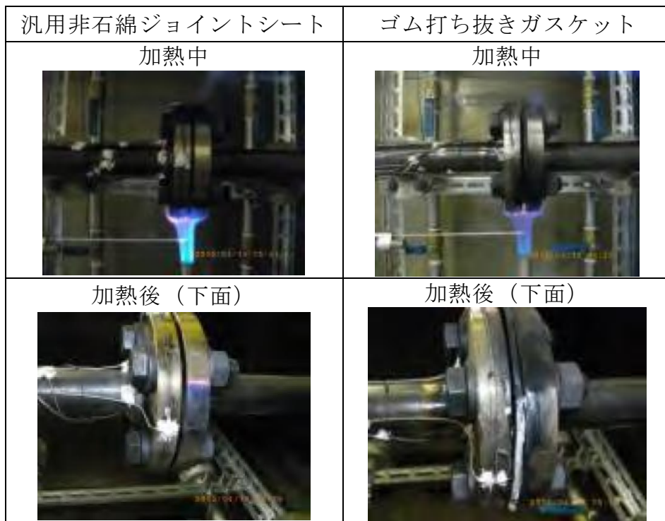
図2 試験体の加熱状況
