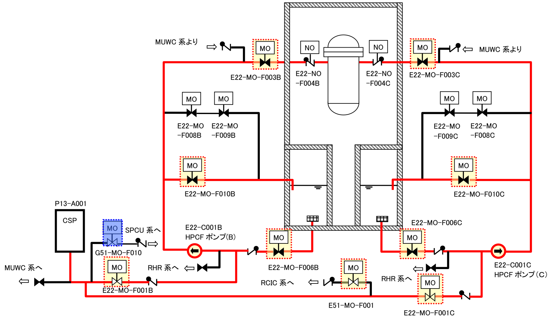
図 4 高圧炉心冷却系
