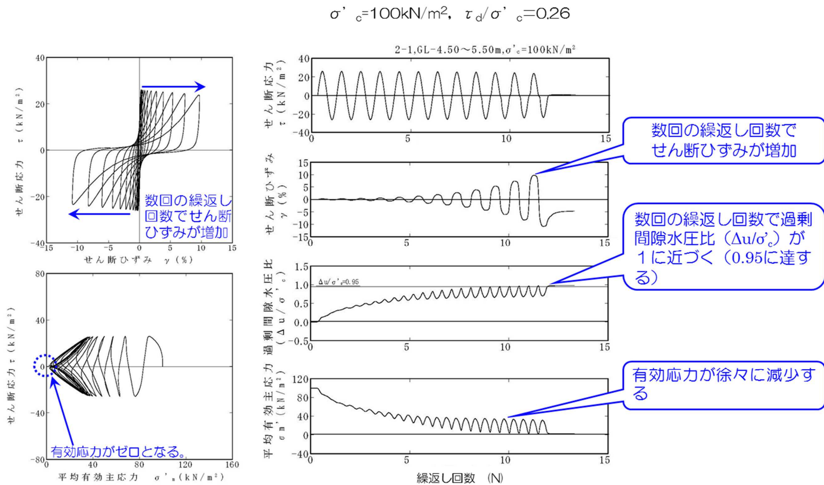
第 4.3.1 図 液状化試験結果の例 (A-1 地点の埋戻土層)
