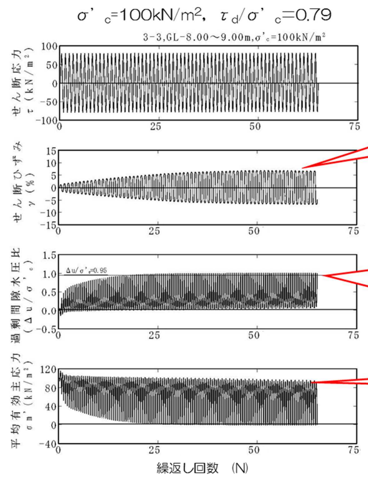
第 4.3.2 図 液状化試験結果の例 (A-1 地点の洪積砂層 I)
