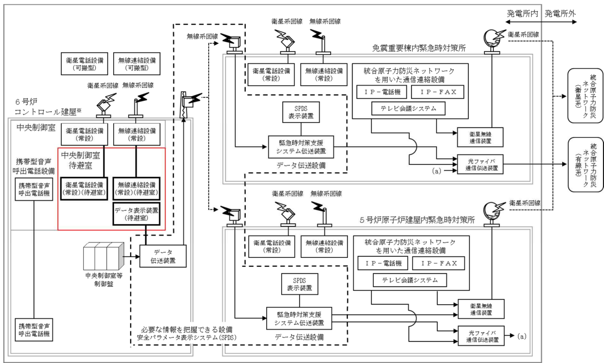
図 59-5-10 データ表示装置（待避室）の概要
