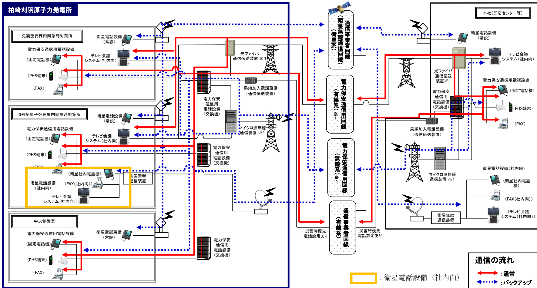
-図 62-9-1 5号炉原子炉建屋内緊急時対策所における衛星電話設備 (社内向)
