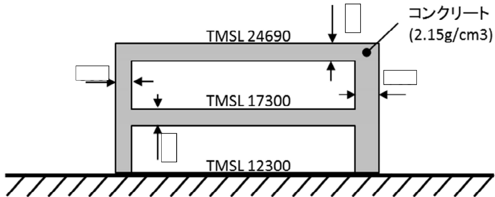
コントロール建屋断面図（B方向）
