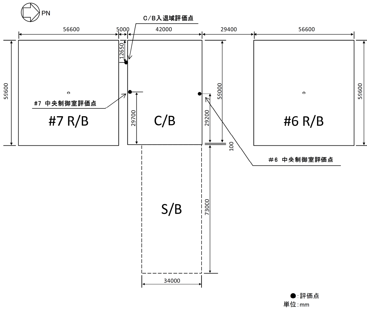
平面図
