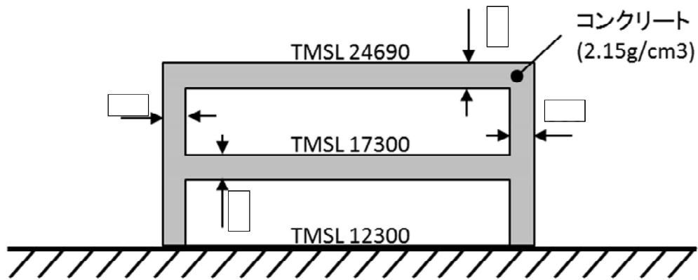
コントロール建屋断面図（A方向）
