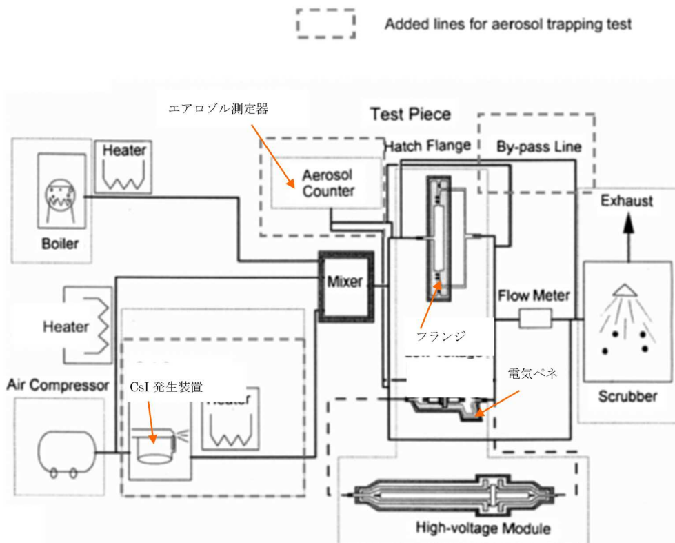
図 2-17-2 試験装置概略図（出典 1）
