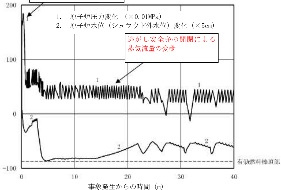
添付 8.2 図 原子炉停止機能喪失における原子炉圧力, 原子炉水位 (シュラウド外水位) の時間変化 (事象発生から 40 分後まで)
