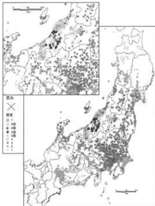
図 278-1 震度分布
