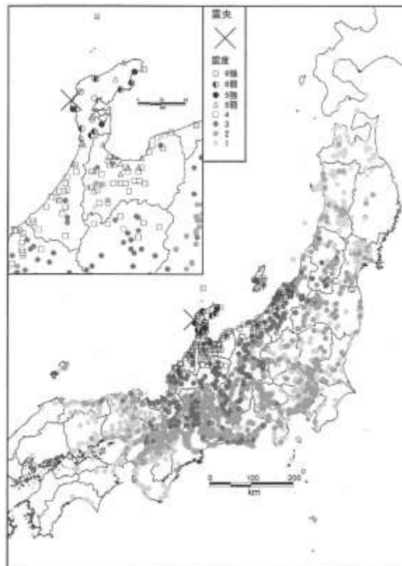
図 367-1 震度分布
