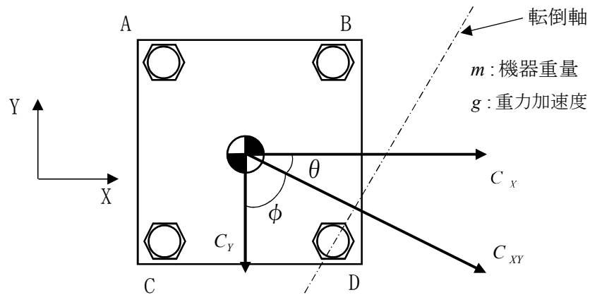
図7-3 水平2方向の地震力による応答 (概要)
