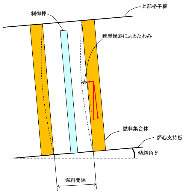
図 1 4 建屋傾斜が発生している状況での燃料集合体のたわみのイメージ
