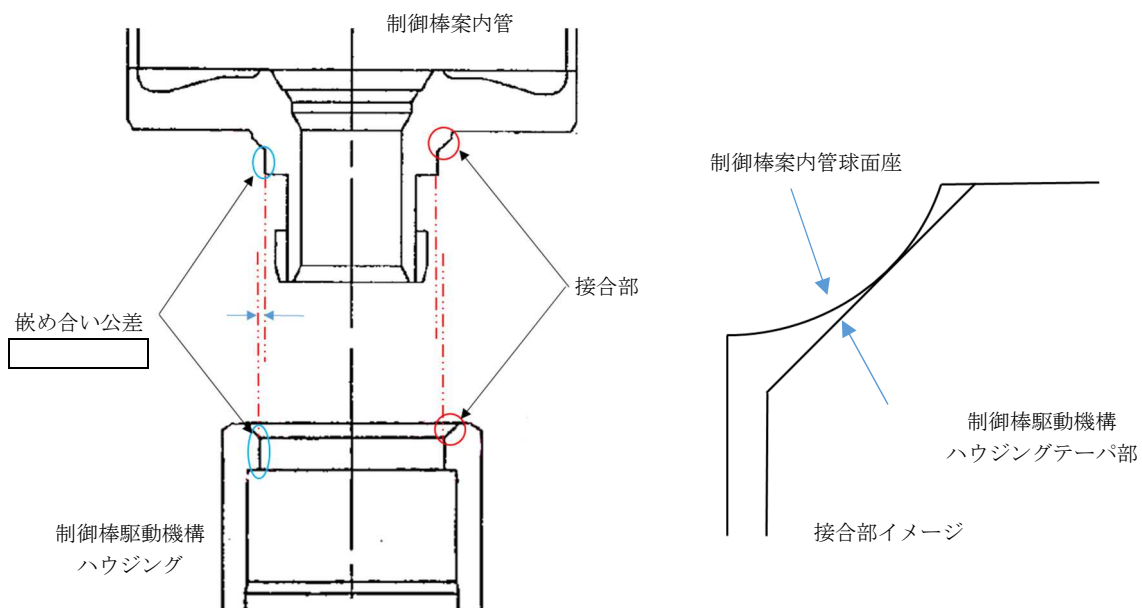
図 1 6 制御棒案内管・制御棒駆動機構ハウジング接合部概念図
