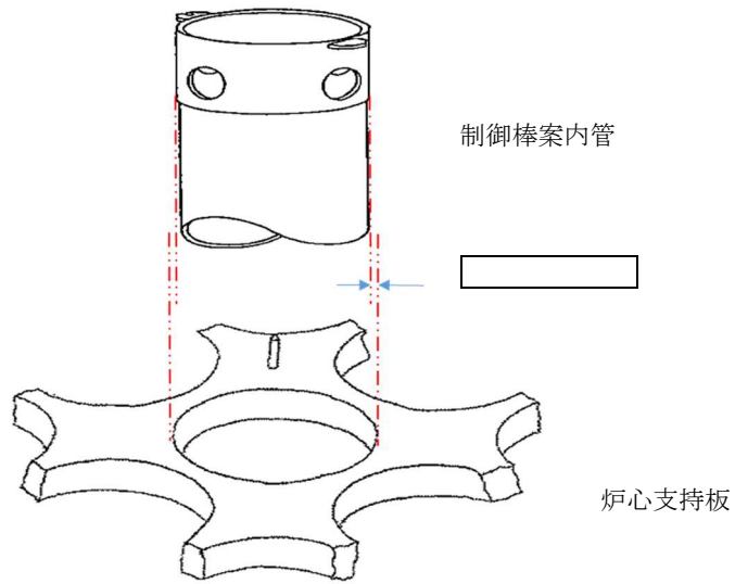
図 1 7 制御棒案内管・炉心支持板接合部概念図
