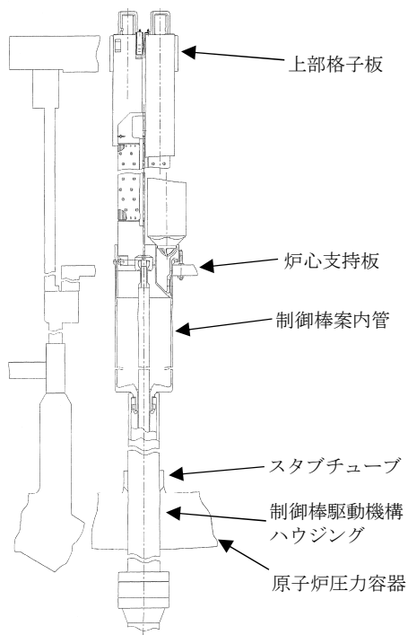
図 1 9 制御棒挿入試験における機器据え付けに対する考慮 (6号炉の例)
