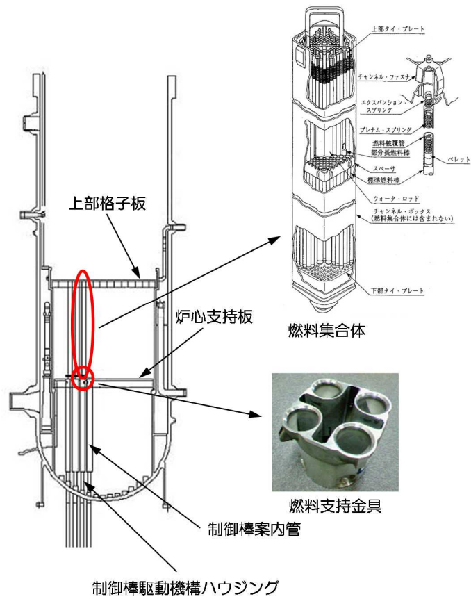
図 1 5 燃料集合体周辺機器の概念図
