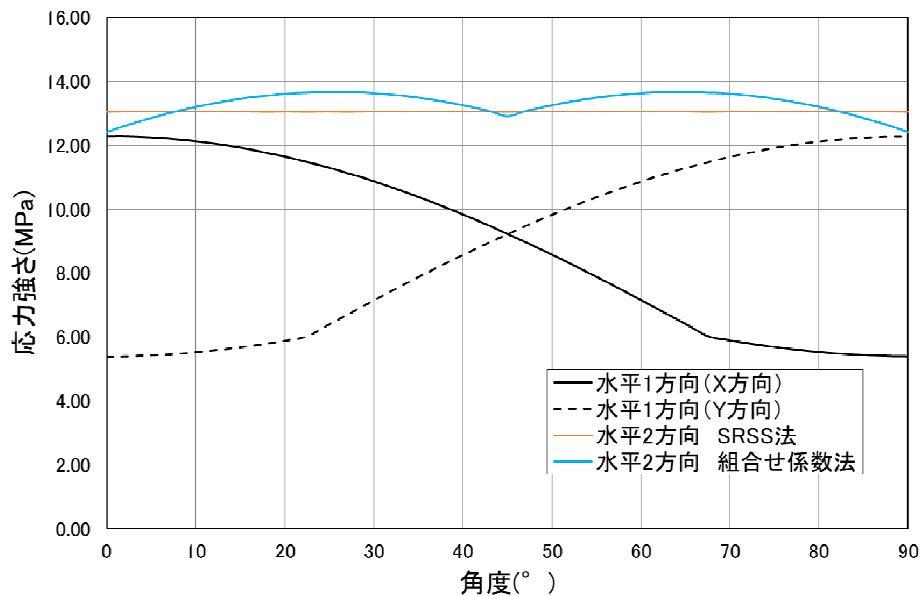
図 4-5 水平地震時組合せ応力強さ分布図
