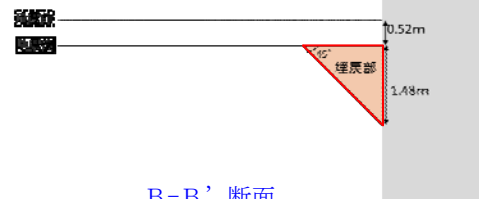
B-B' 断面
