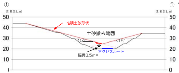
①-① '断面図
