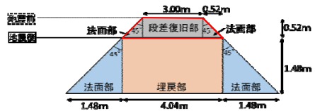
C-C' 断面
