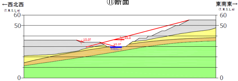
⑫断面
