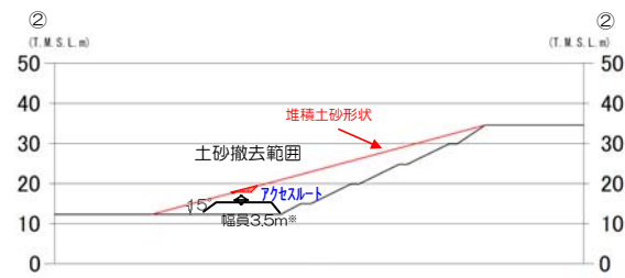
②-② '断面図
