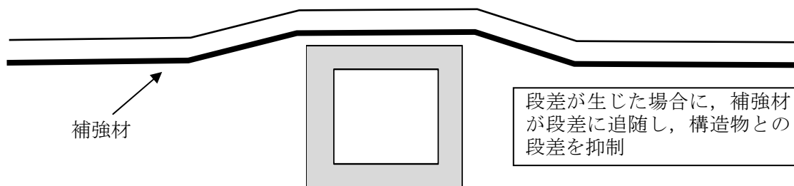
図 2 段差抑制対策イメージ
