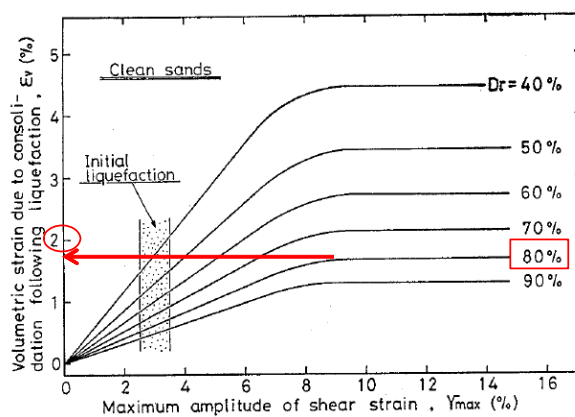
最大せん断ひずみと体積ひずみの関係 (石原ら1992)
