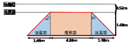
A-A' 断面
