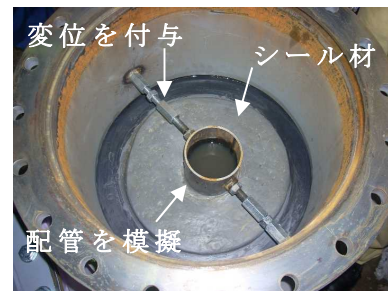
試験装置内部
