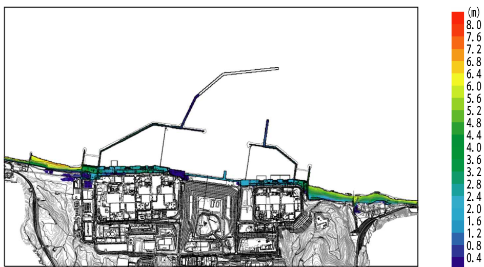
添付第 2-57 図 基準津波 3 における最大浸水深分布 (防波堤あり，防潮堤あり，現地形)
