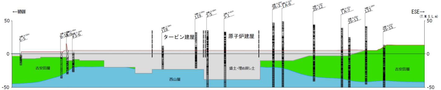
3号炉汀線直交断面
