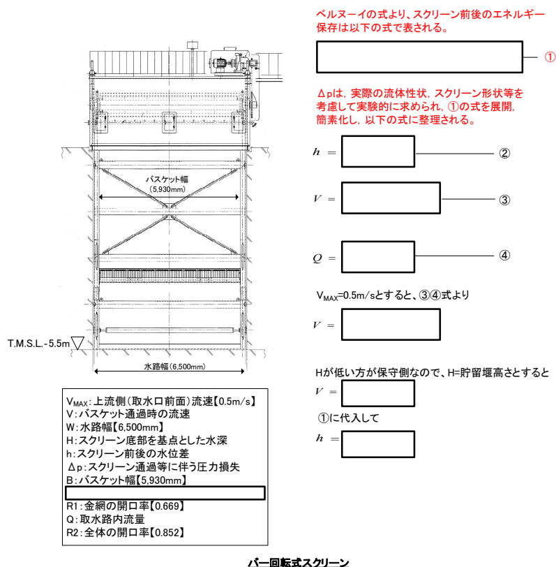
第 2.5-29 図 津波流速により生じるスクリーン部水位差
