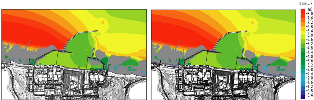
1) 防潮堤あり／沈下・斜面崩壊なし
