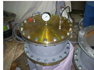
試験装置外観
