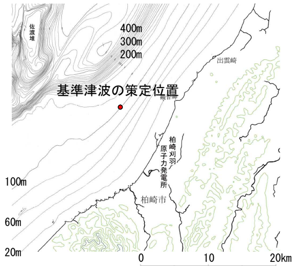
評価位置 (水深100m，敷地の沖合約7km)
