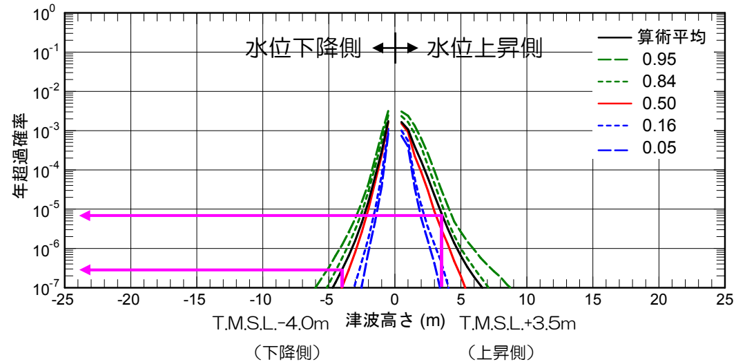
フラクタイルハザード曲線（基準津波策定位置）
