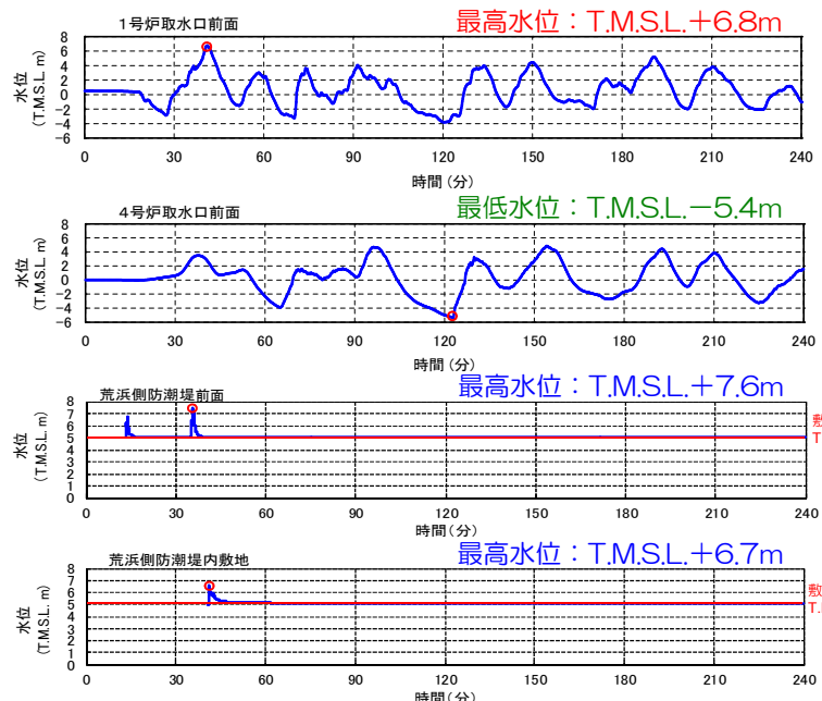
時刻歴波形 (上から、取水口前面上昇側、取水口前面下降側、荒浜側防潮堤外、荒浜側防潮堤敷地)
