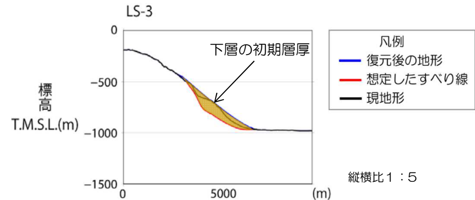
初期土砂層厚の設定例（LS-3）
