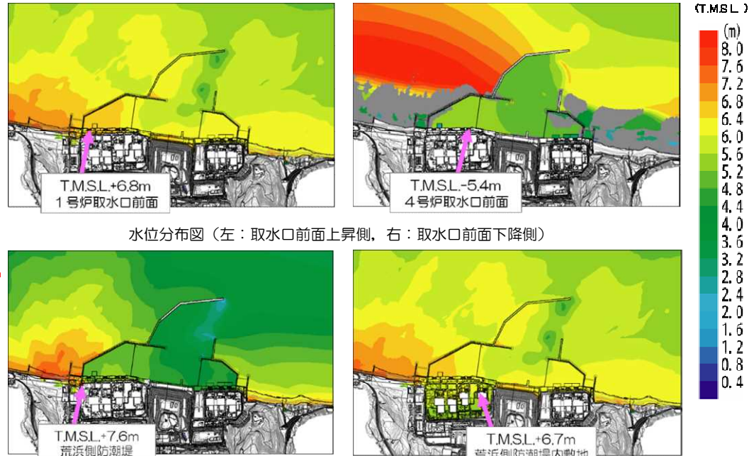
水位分布図 (左：荒浜側防潮堤外上昇側，右：荒浜側防潮堤敷地内上昇側)
