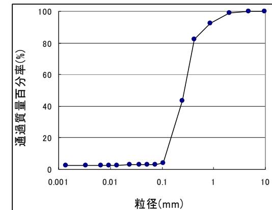
海底砂の粒度分布
