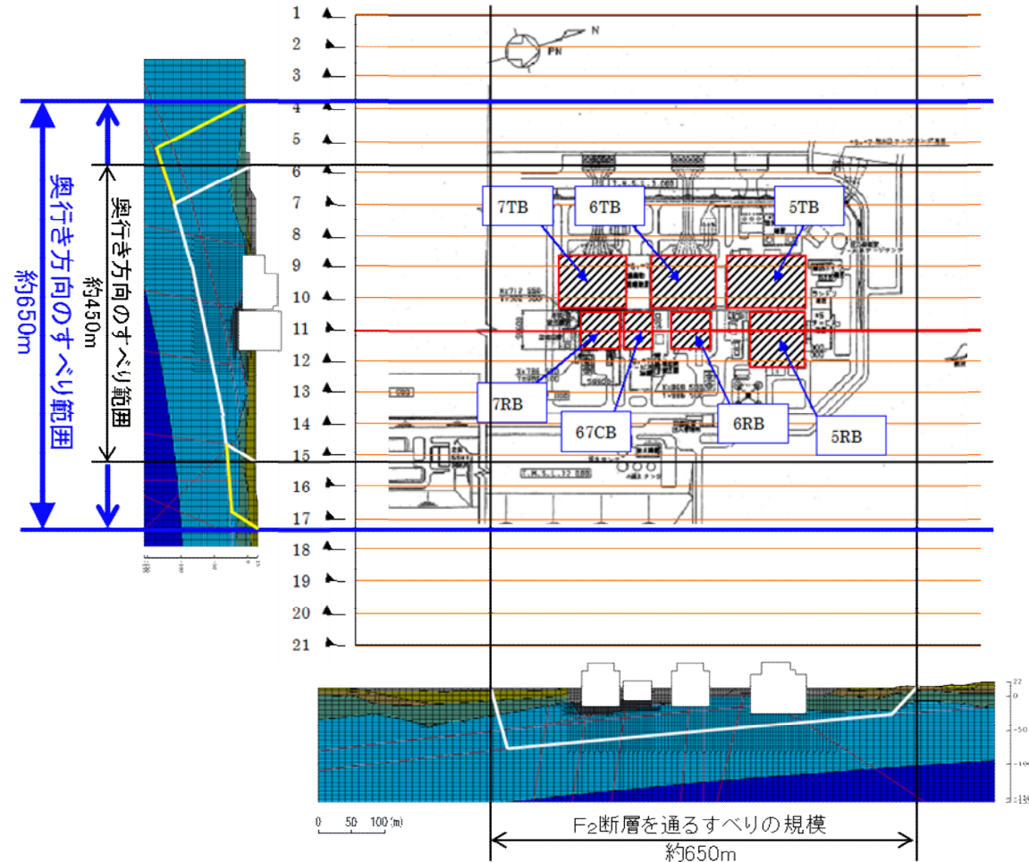
5, 6, 7号炉原子炉建屋 汀線平行断面
