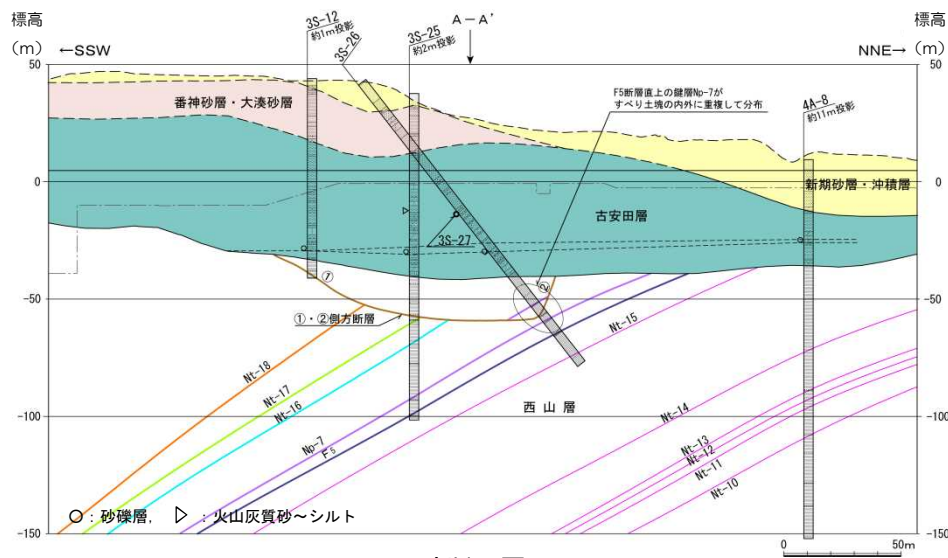
5-5' 断面図
