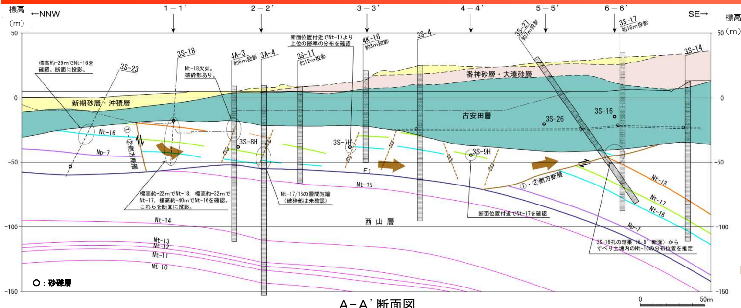
A-A' 断面図
