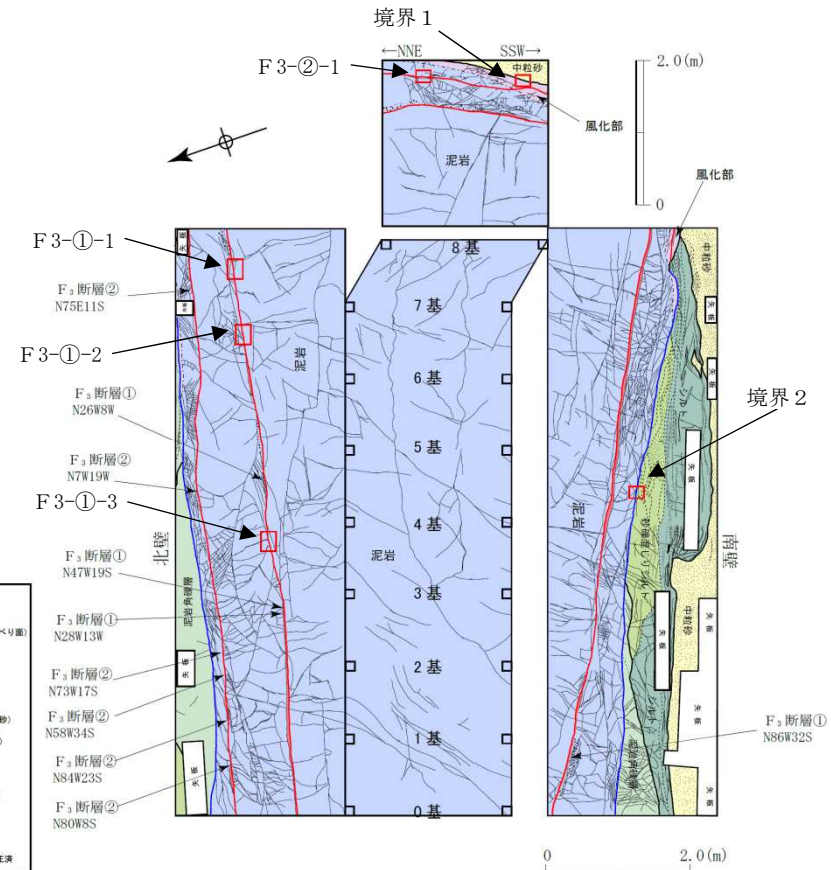
F3立坑試料採取位置
