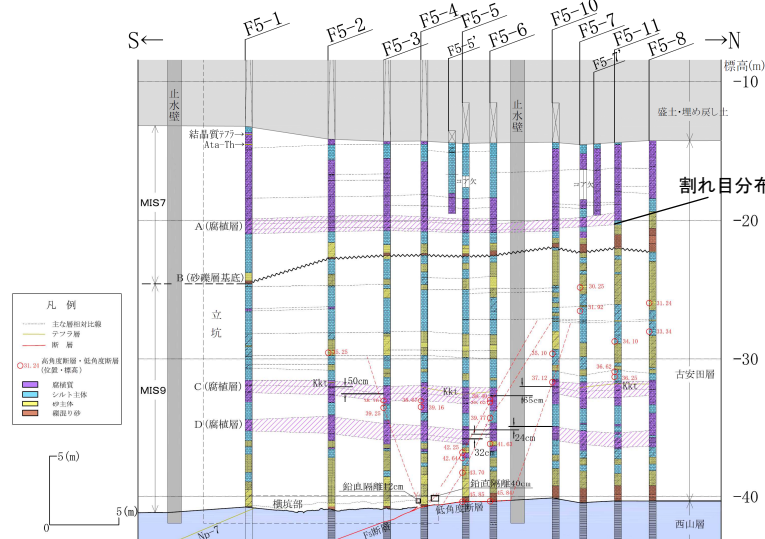
F5立坑近傍の地質断面図※
