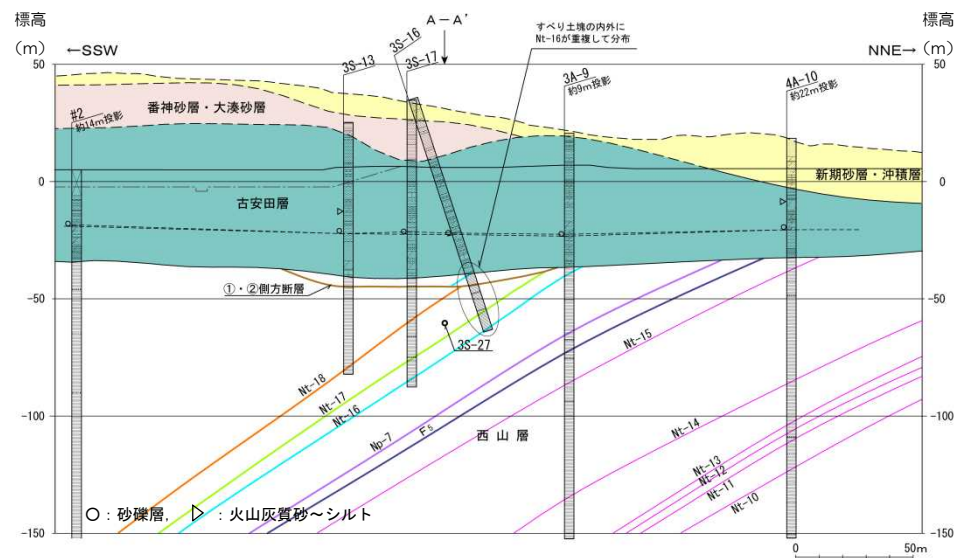
6-6' 断面図
