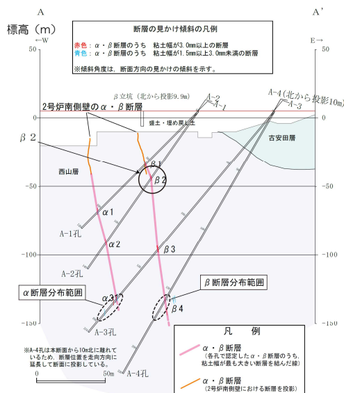
1・2号炉間地質断面図 (A-A' 断面)
