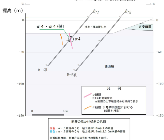
X線回折分析試料採取位置図 (1号炉南方面断面図)
