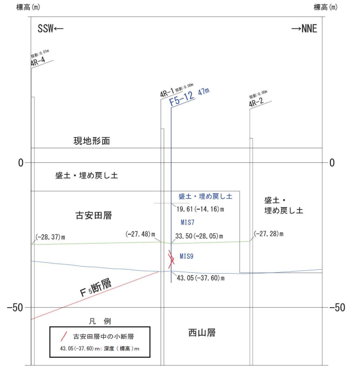
地質断面図
