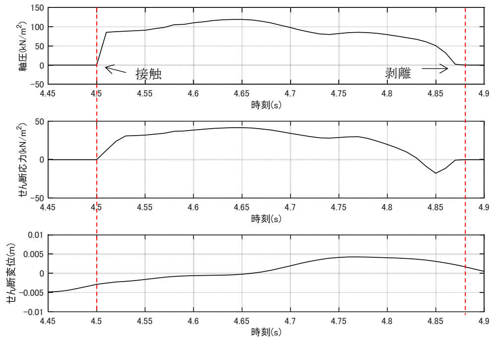
第 4.5 図 軸圧，せん断応力及びせん断変位の時刻歴波形（4.45 秒～4.90 秒拡大）
