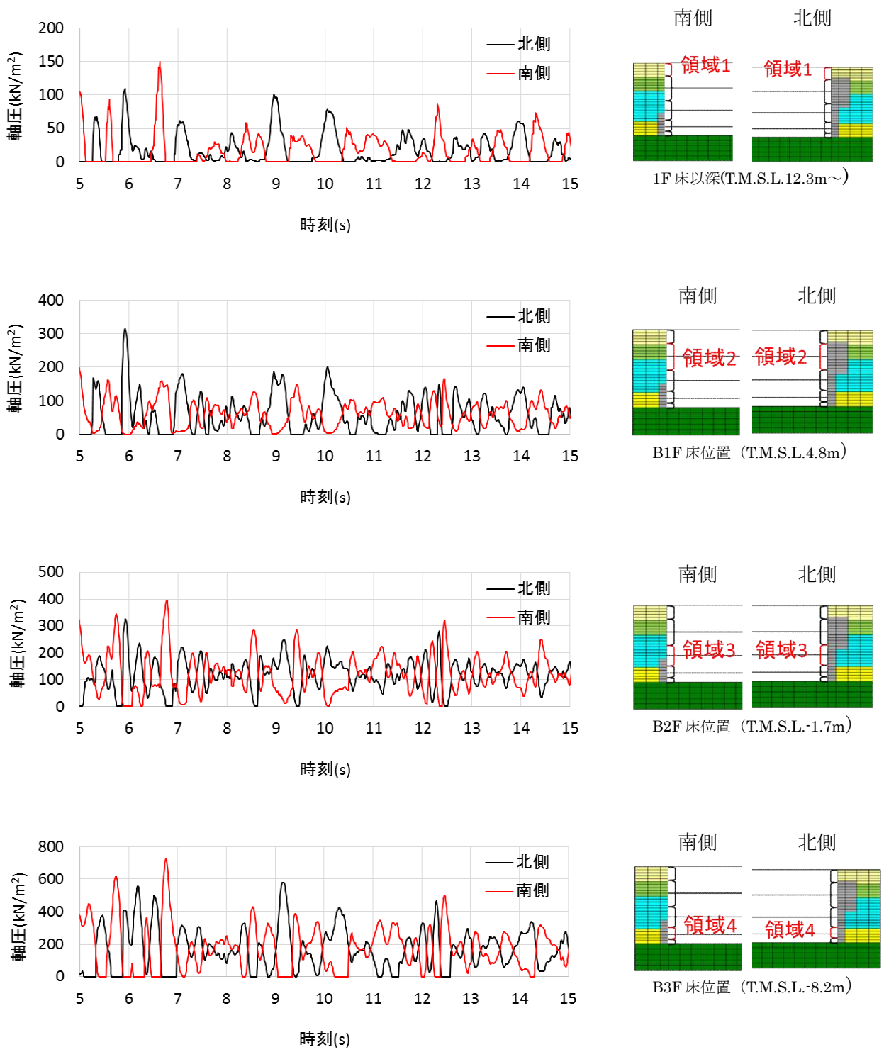
第 4.2.1.3 図 南側と北側の軸ばねの軸圧の時刻歴の比較 (NS 方向基本モデル)
