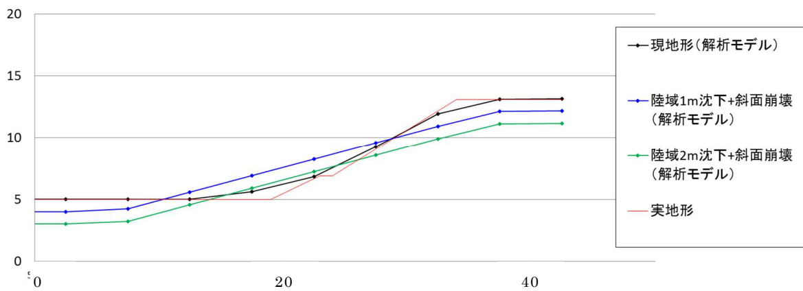
(2) 荒浜側防潮堤内敷地 山側斜面 添付第 3-2 図 実地形とモデル化した地形の比較
