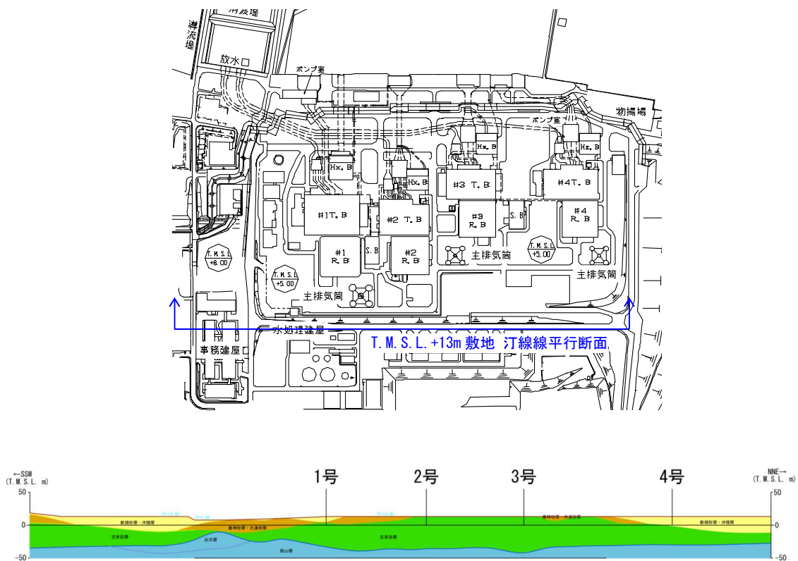
添付第 9-8 図 地質断面図 (荒浜側敷地汀線平行断面)
