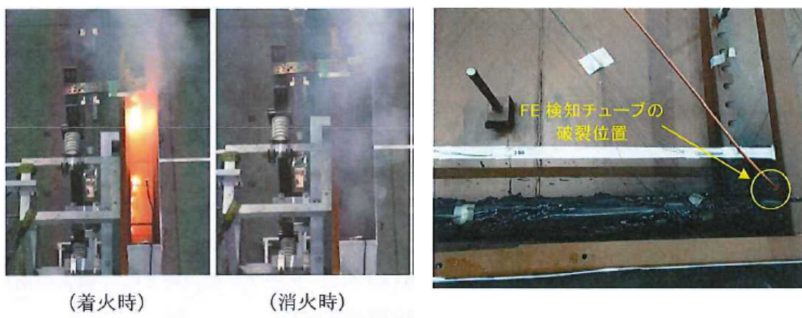
第 9 図：試験 V1 における発火・消火時の状態
