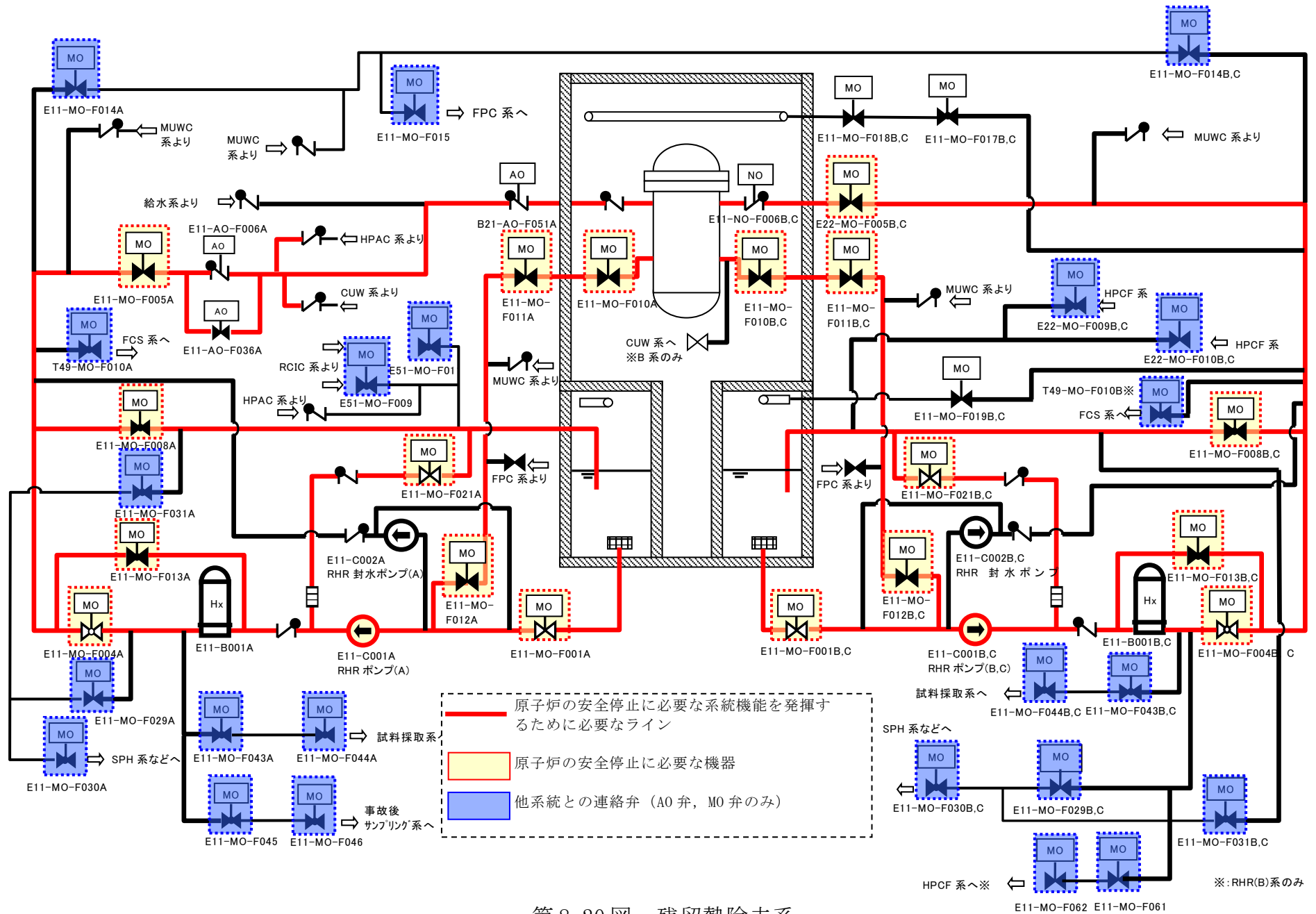
第8-20図 残留熱除去系
