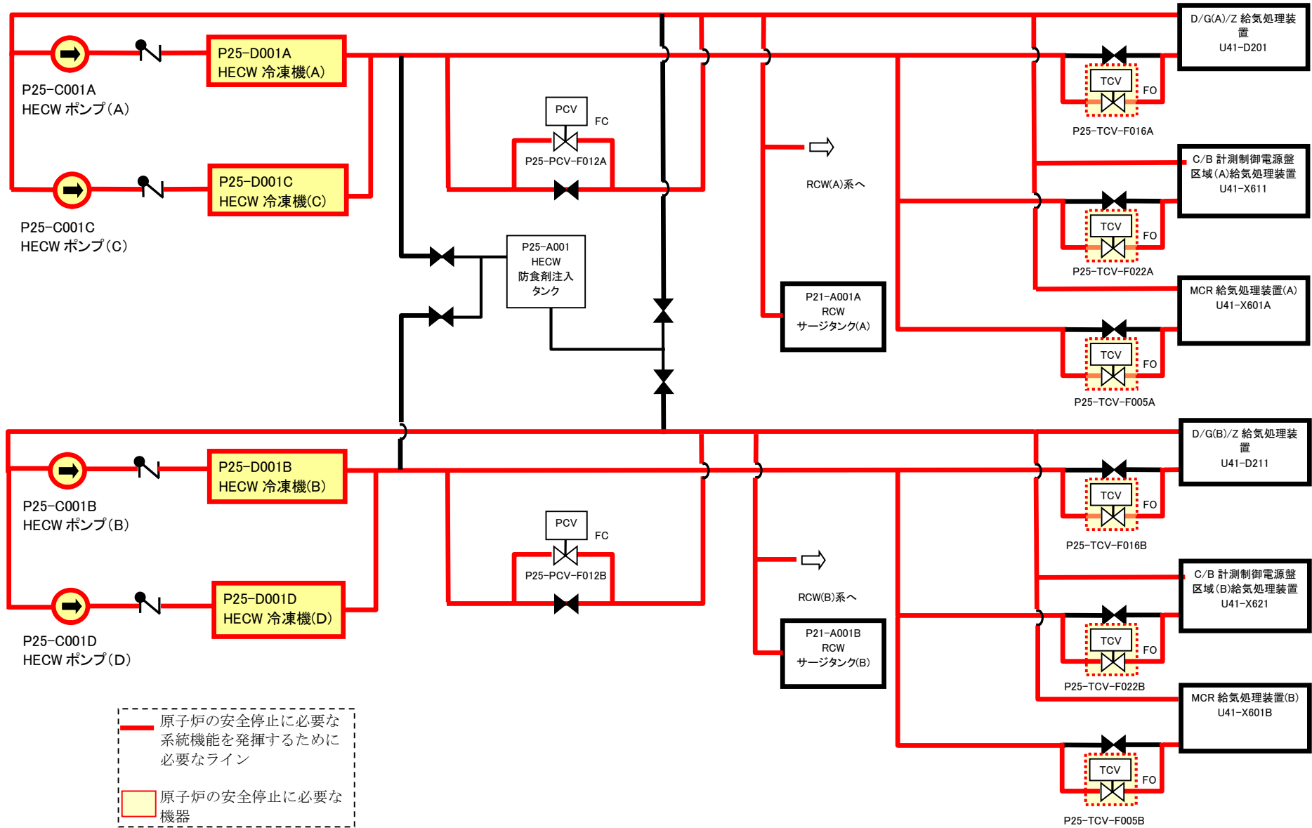
第 8 図 換気空調補機非常用冷却系
