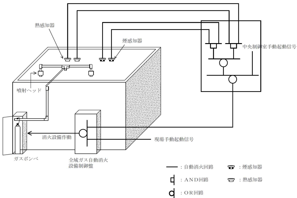
第 1-20 図：全城ガス消火設備の概要
