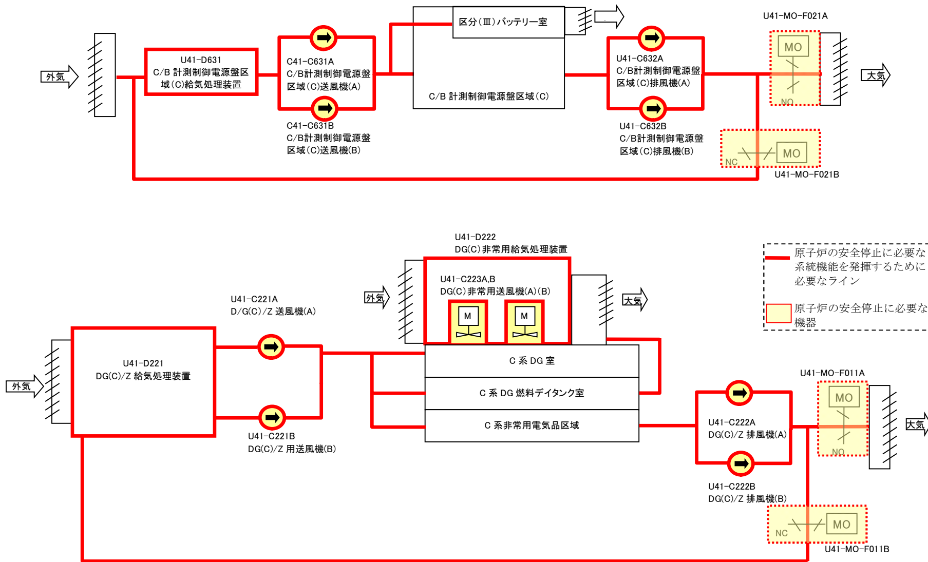
第 13 図 非常用換気空調系 (その 2)
