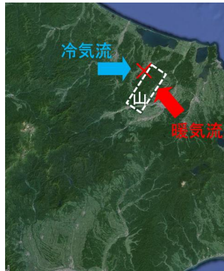
親雲の発生位置（点線内）と移動方向 竜巻の発生位置（×）と影響が指摘される山（点線部）
