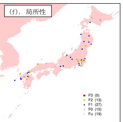
図 2.2.2.1 総観場ごとの竜巻発生地点の分布(1961年～2012年) (気象庁竜巻等の突風データベースのデータをもとに作成)
