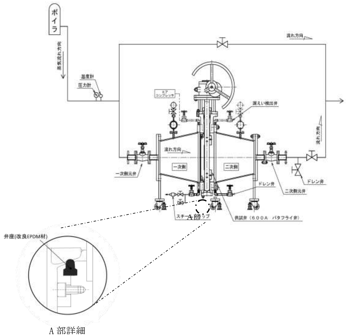
図 8-8 蒸気通気試験装置概要図
