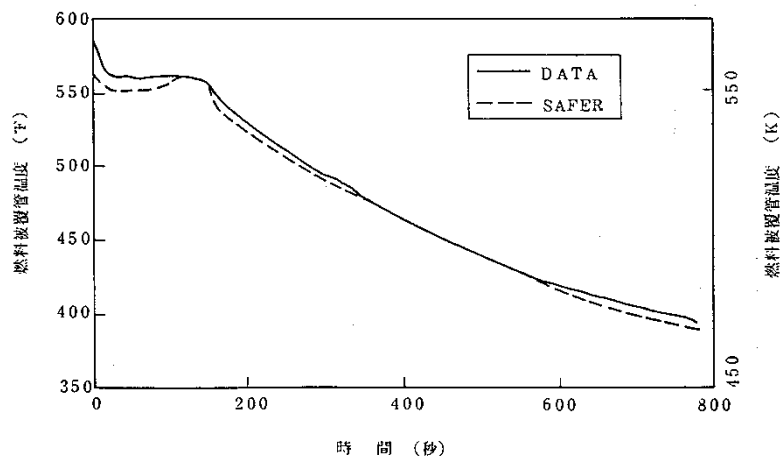
图 4-32 燃料被覆管温度变化 (F I S T - A B W R, C S 配管破断)
