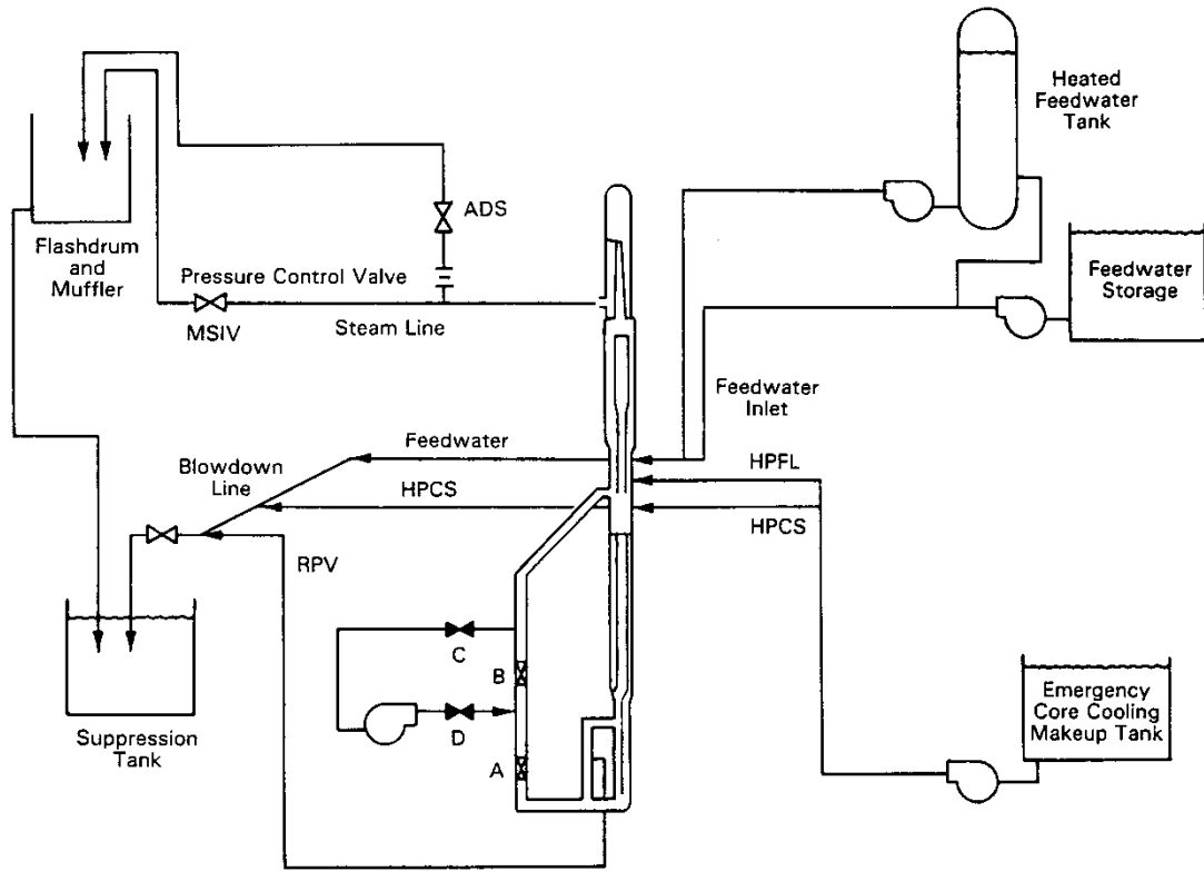
図 4-24 F I S T - A B W R 系統図
