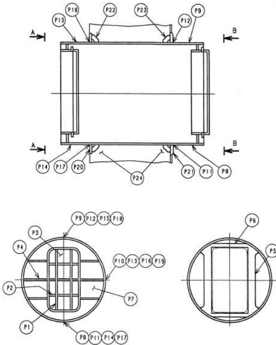
図5-3 上部ドライウェル所員用エアロック
