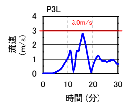
基準津波3 地点P3L 第二波
