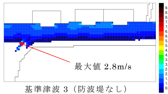
第 2.5-28 図 大湊側護岸部における海域方向最大流速
