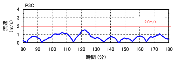
基準津波1 地点P3C(代表例)
