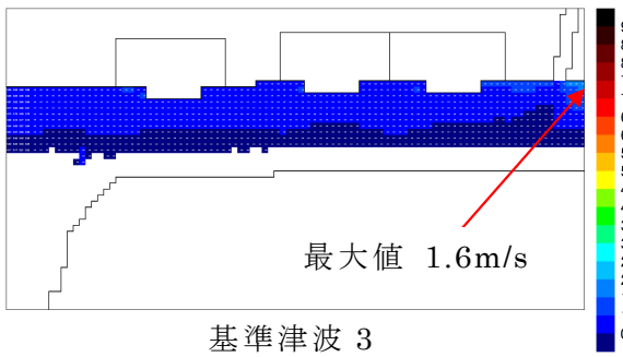
第 2.5-28 図 大湊側護岸部における海域方向最大流速
