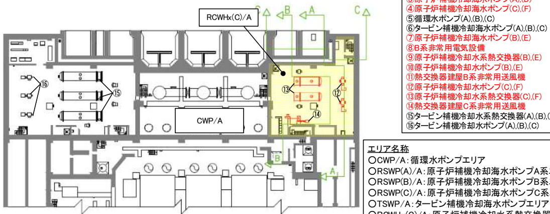
タービン建屋地下2階 平面図
