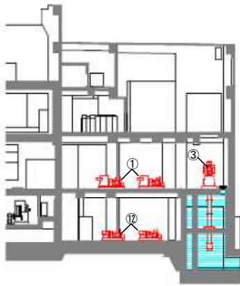
A-A断面
