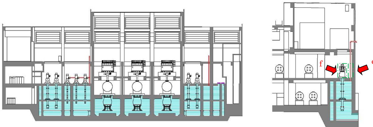
A-A 断面
