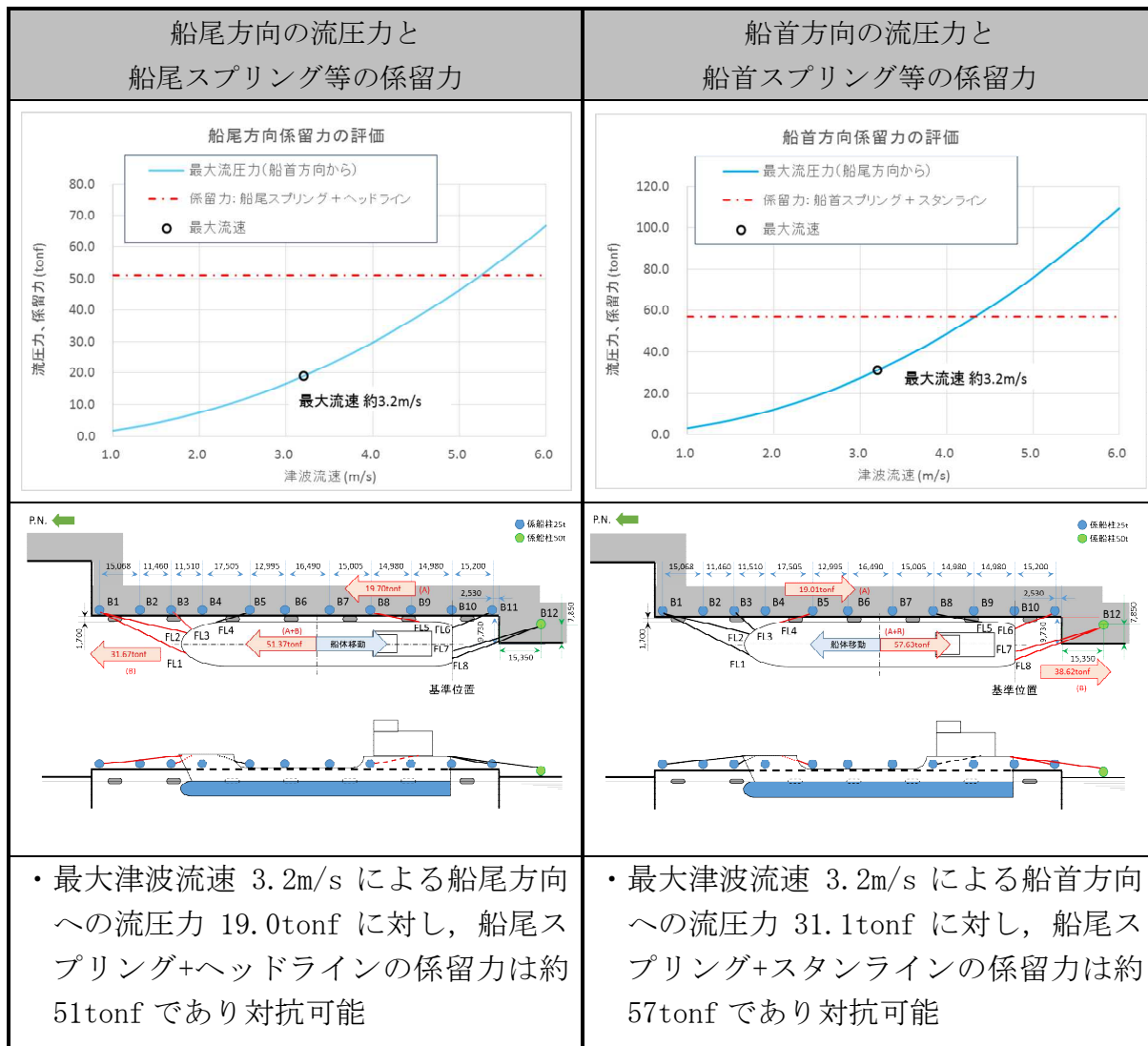
添付第 21-6 図 流圧力と係留力の比較
