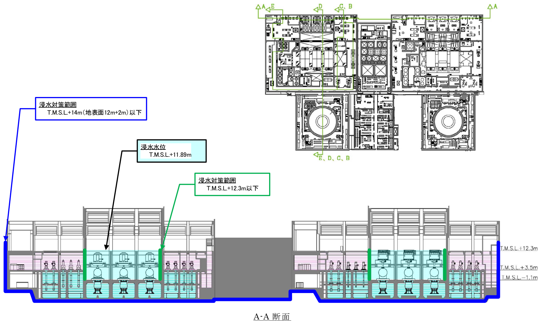
添付第 14-5 図 貫通部止水処置及び床ドレンライン浸水防止治具の実施範囲 (7号炉縦断面) (1/2)
