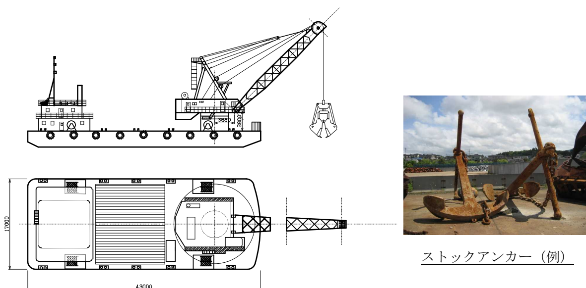
添付第 23-1 図 浚渫船の外形図
